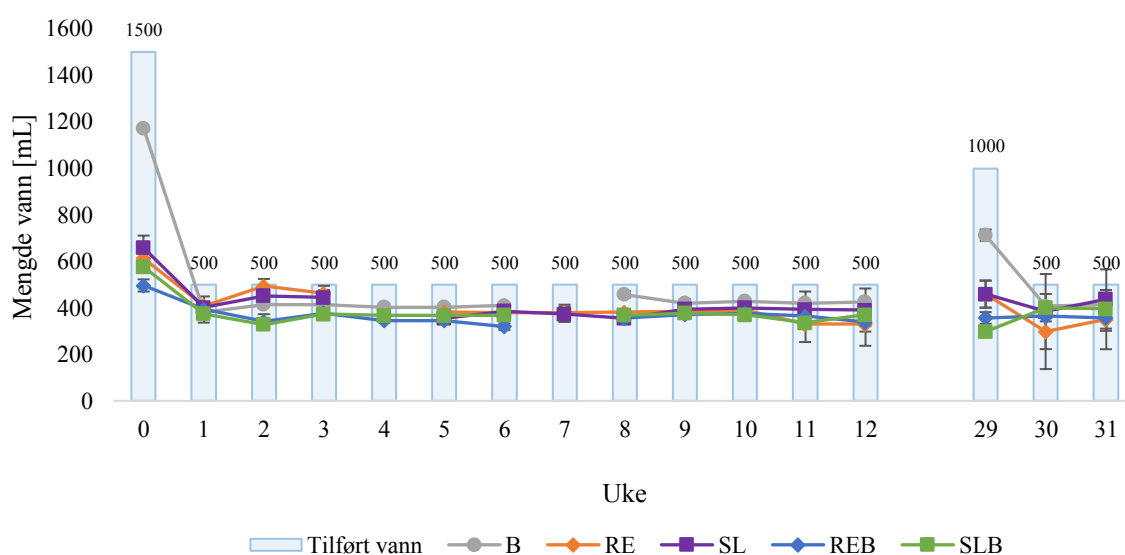
Figur 10- Ukentlig mengde tilført vann til kolonnene vist med blå søyler. Alle kolonnene mottok samme mengde vann. Gjennomsnittlig mengde drenert eluat fra de ulike kolonnenegjentakene vises som punkter inkludert standardavvik som viser variasjon i drenert eluat imellom kolonnenegjentakene av samme type. (B: n=2, RE: n=2, SL: n=2, REB: n=3, SLB: n=3).
