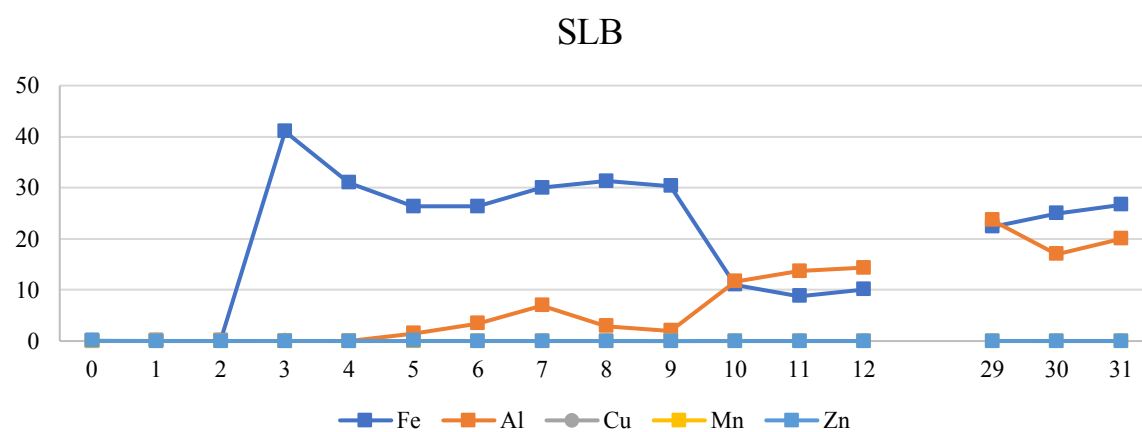
Figur F.8 - Analyseresultater Fe, Al, Cu, Mn, Zn [mg/L].
