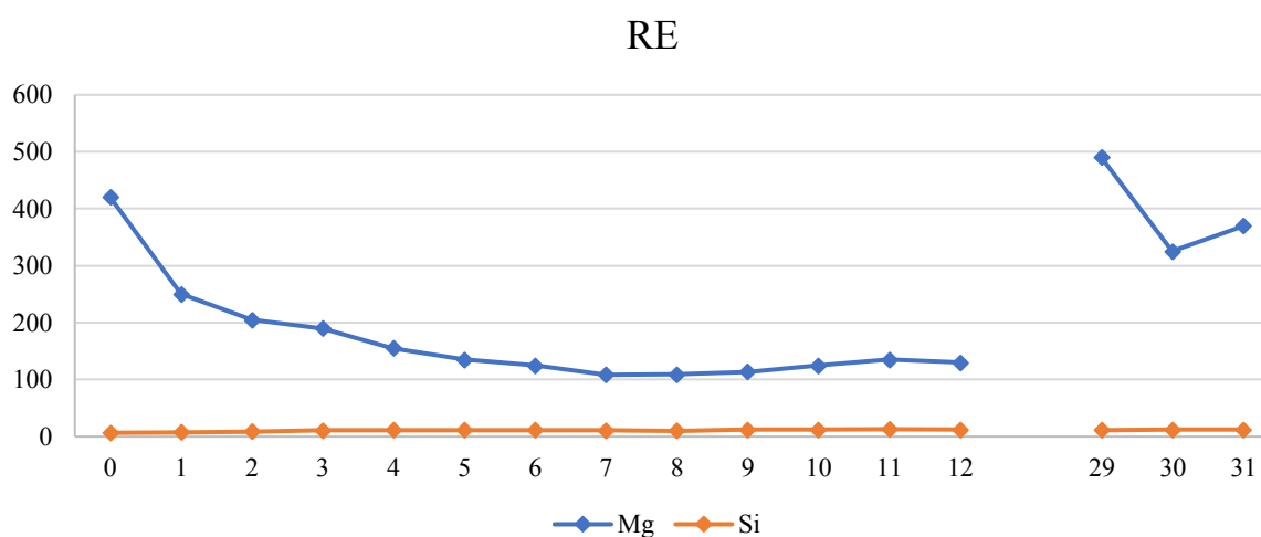
Figur F.13 - Analyseresultater Mg og Si [mg/L].
