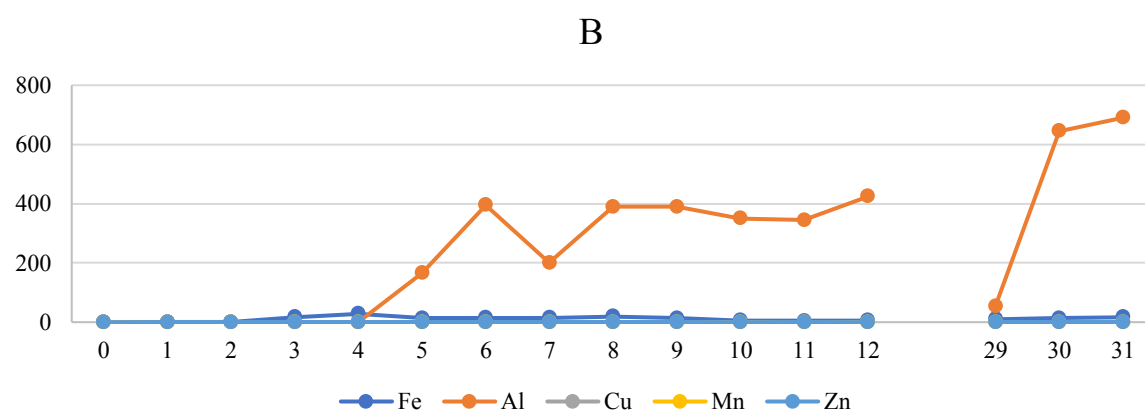
Figur F.26 - Analyseresultater Fe, Al, Cu, Mn, Zn [mg/L].
