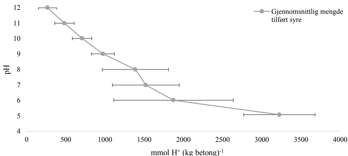
Figur 9- Gjennomsnittlig målt pH og mengde tilført syre i tre titreringsforsøk av betong. Punkter representerer gjennomsnittlig tilført syre uttrykt som \text{mmol H}^+ ( \text{kg betong}^{-1} ) ved hvert pH- nivå. Standardavvik viser variasjonen i mengde tilført syre ved hvert pH- nivå
