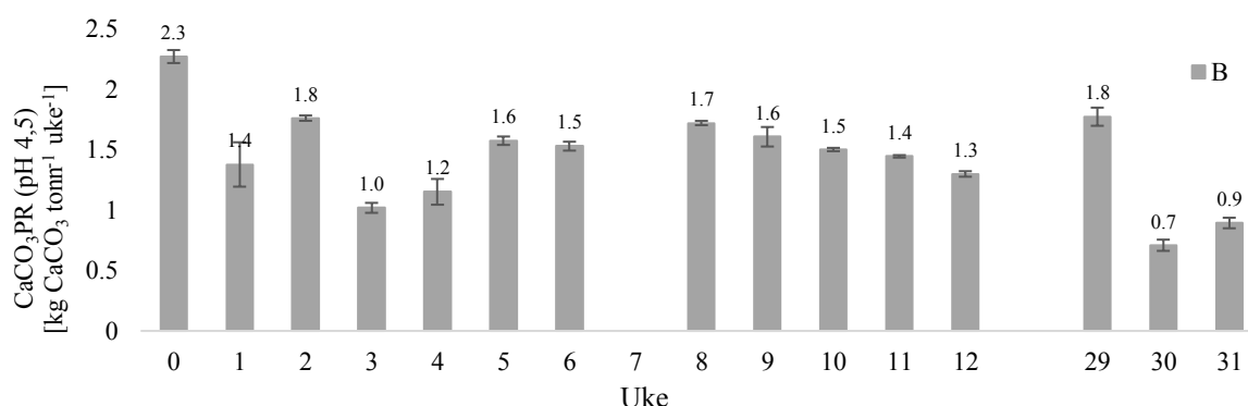
Figur 16- Ukentlig gjennomsnittlig alkalinitet for betongkontrollene ved pH 4,5 uttrykt som \text{CaCO}_3\text{PR} [ \text{kg CaCO}_3 \text{ tonn}^{-1} \text{ uke}^{-1} ] i samtlige uker, foruten uke 7 hvor mengde eluat ikke ble registrert, samt standardavvik som representerer variasjonen imellom betongkontrollene i ukentlig beregnet SPR. (B: n=2).
