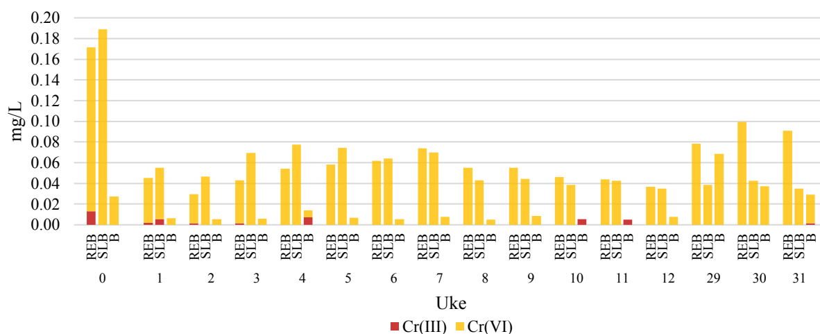
Figur 26- Gjennomsnittlig utlekking av Cr(III) vist i rødt og Cr(VI) vist i gult i betongbehandlede aluskerkolonner (REB: n=3 og SLB: n=3) og betongkolonner (B: n=2). Summen av Cr(III) og Cr(VI) antas å representere total Cr.
