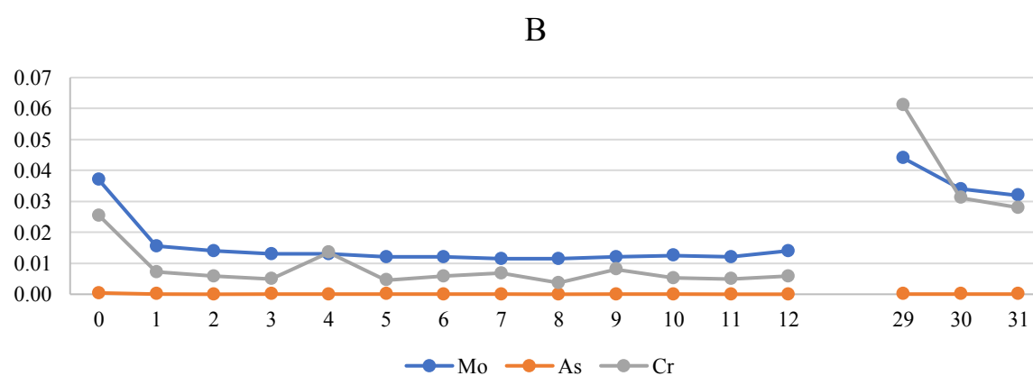
Figur F.27 - Analyseresultater Mo, As, Cr [mg/L].
