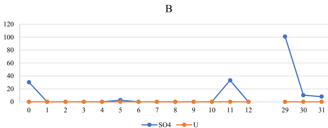
Figur F.28 - Analyseresultater SO4 og U [mg/L].
