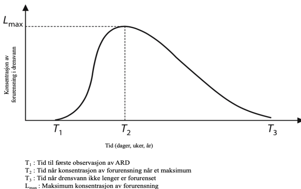
Figur 30- Illustrert utvikling av konsentrasjonen av en forurensning i ARD. Modifisert figur fra Fig. 3.7 av Lottermoser (2007).
