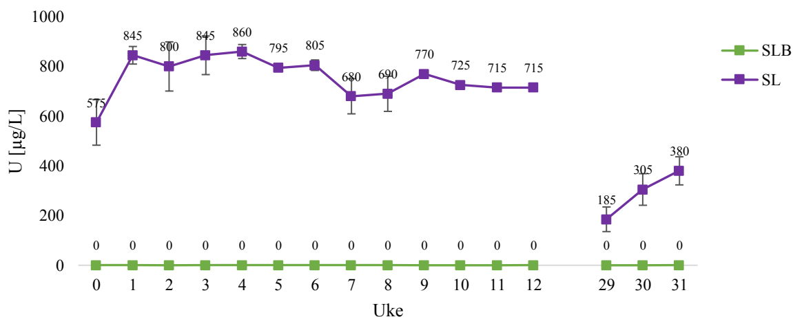
Figur 20- Ukentlig gjennomsnittlig utlekking av U fra ubehandlet (SL) og behandlet (SLB) alunskifer fra Slemmestad [ \mu\text{g/L} ]. Standardavvik representerer variasjonen i målt U imellom kolonnegjentakene. (SL: n=2, SLB: n=3).
