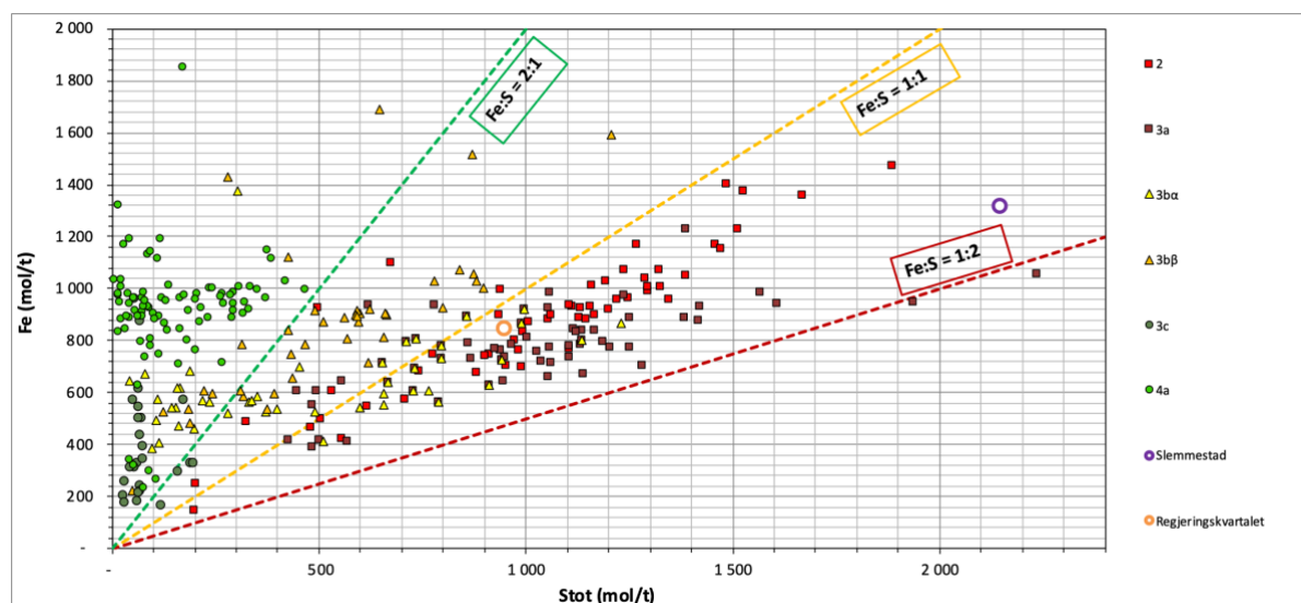
Figur D.6- Fe-S- diagram fremstilt med exceldokument med datasett utarbeidet av NGI.
