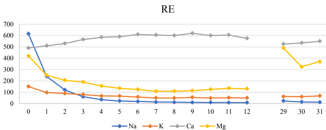
Figur F.12 - Analyseresultater Na, K, Ca, Mg [mg/L].
