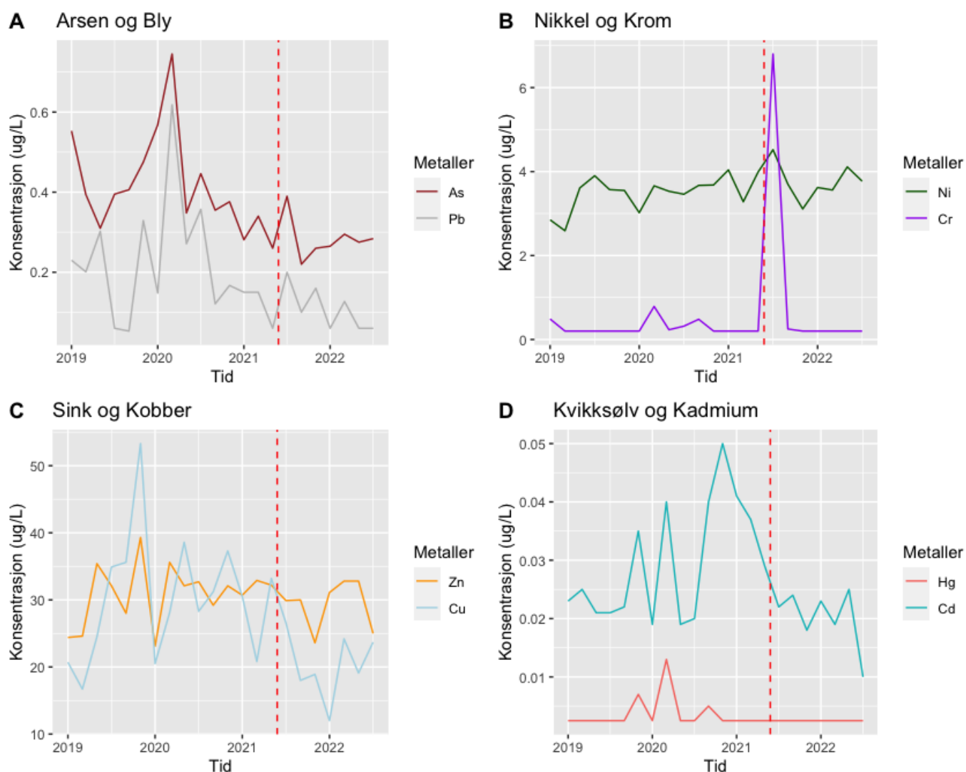
Figur 6: Utslipp av tungmetaller fra BRA i perioden 2019-2022. Stiplede linje representerer oppstart av prøveperioden etter oppgradering av renseanlegget. A) Utslipp av arsen og bly; B) Utslipp av nikkel og krom; C) utslipp av sink og kobber; D) utslipp av kvikksølv og kadmium.
