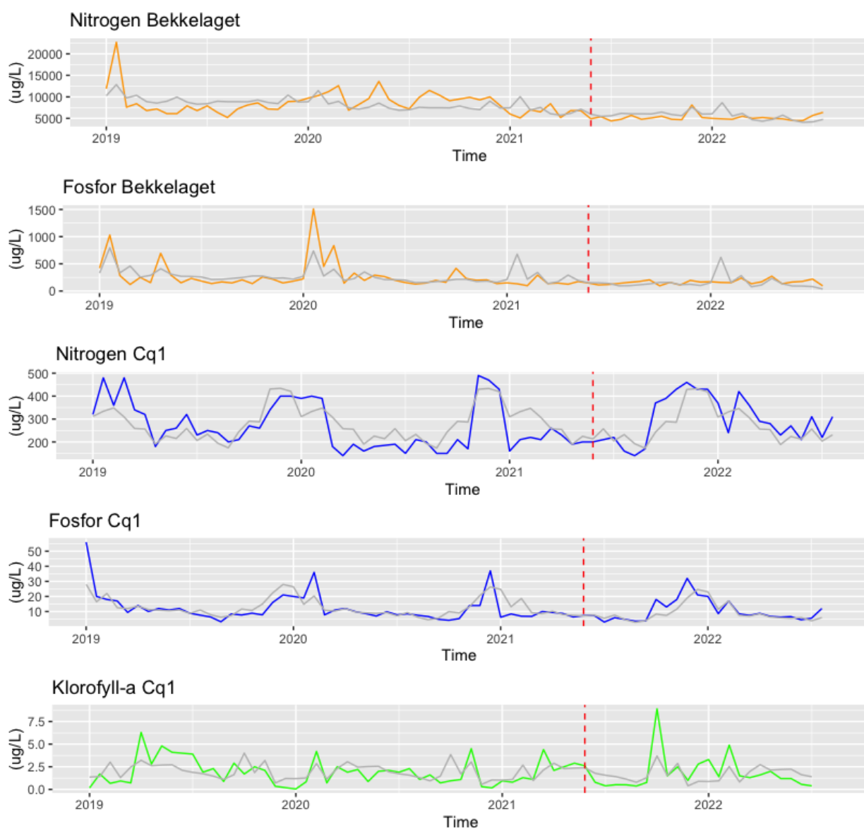
Figur 5: Rød stiplete linje markerer starten på prøveperioden for det oppgraderte renseanlegget. Fra toppen: (1) Bekkelagets utslipp av nitrogen (oransje) og trendlinjen (grå). (2) Bekkelagets utslipp av fosfor (oransje) og trendlinje (grå). (3) Målingene av nitrogen ved Cq1 (blå) og trendlinjen (grå). (4) Målingene av fosfor ved Cq1 (blå) og dens trendlinje (grå). (5) målingene av klorofyll-a ved Cq1 (grønn) og dens trendlinje (grå). Alle konsentrasjoner er oppgitt i mikrogram per liter ( \mu\text{g/L} ), og målingene ved Cq1 ble gjort i overflatelaget (0-2 meter).
