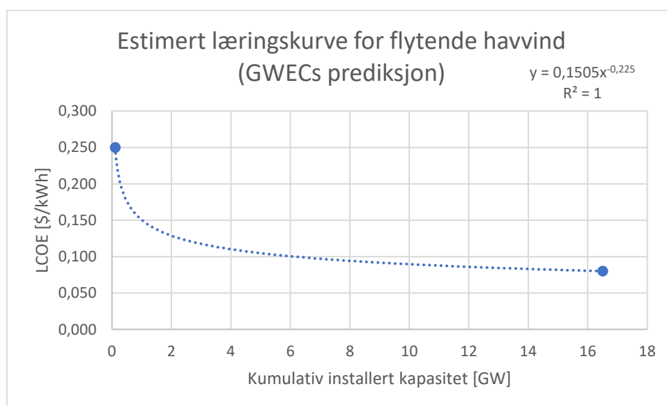
Figur 14: Estimert læringskurve for flytende havvind basert på GWECs prediksjon til installert kapasitet i 2030, og NVEs estimat for LCOE, som også ble brukt i forrige kurve. GWEC har noe høyere forventning enn Bloomberg, med 16,5 GW installert kapasitet innen 2030. Læringsraten for denne kurven blir 14,4 %. Læringsraten for denne
