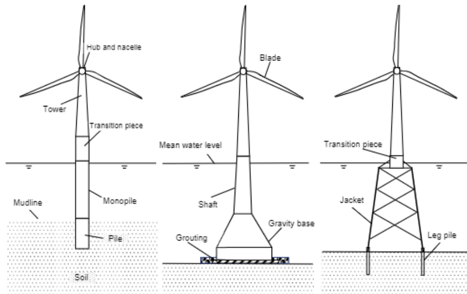
Figur 2: Bunnfaste fundamenter for havvind. Kilde: (Jiang, 2021) , gjengitt med tillatelse etter CC BY-lisensregler ( https://creativecommons.org/licenses/by/4.0/ ).
