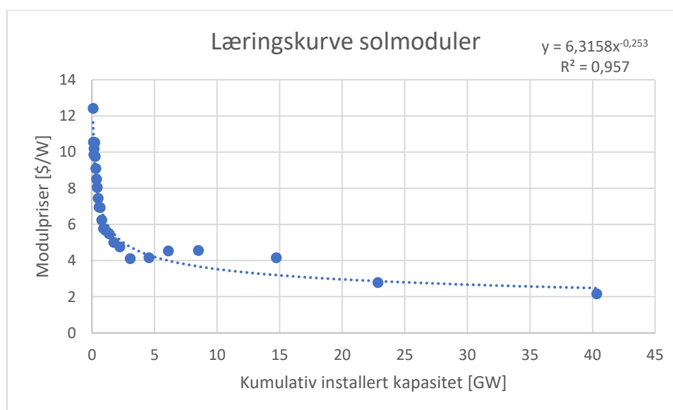
Figur 6: Historisk læringskurve for solmoduler mellom 1983-2010.
