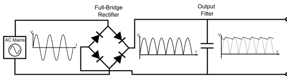
Figur 9 AC-input blir omformet til DC gjennom en helbro likeretter (2 og 2 dioder parallelt), (Hudson, 2022)
