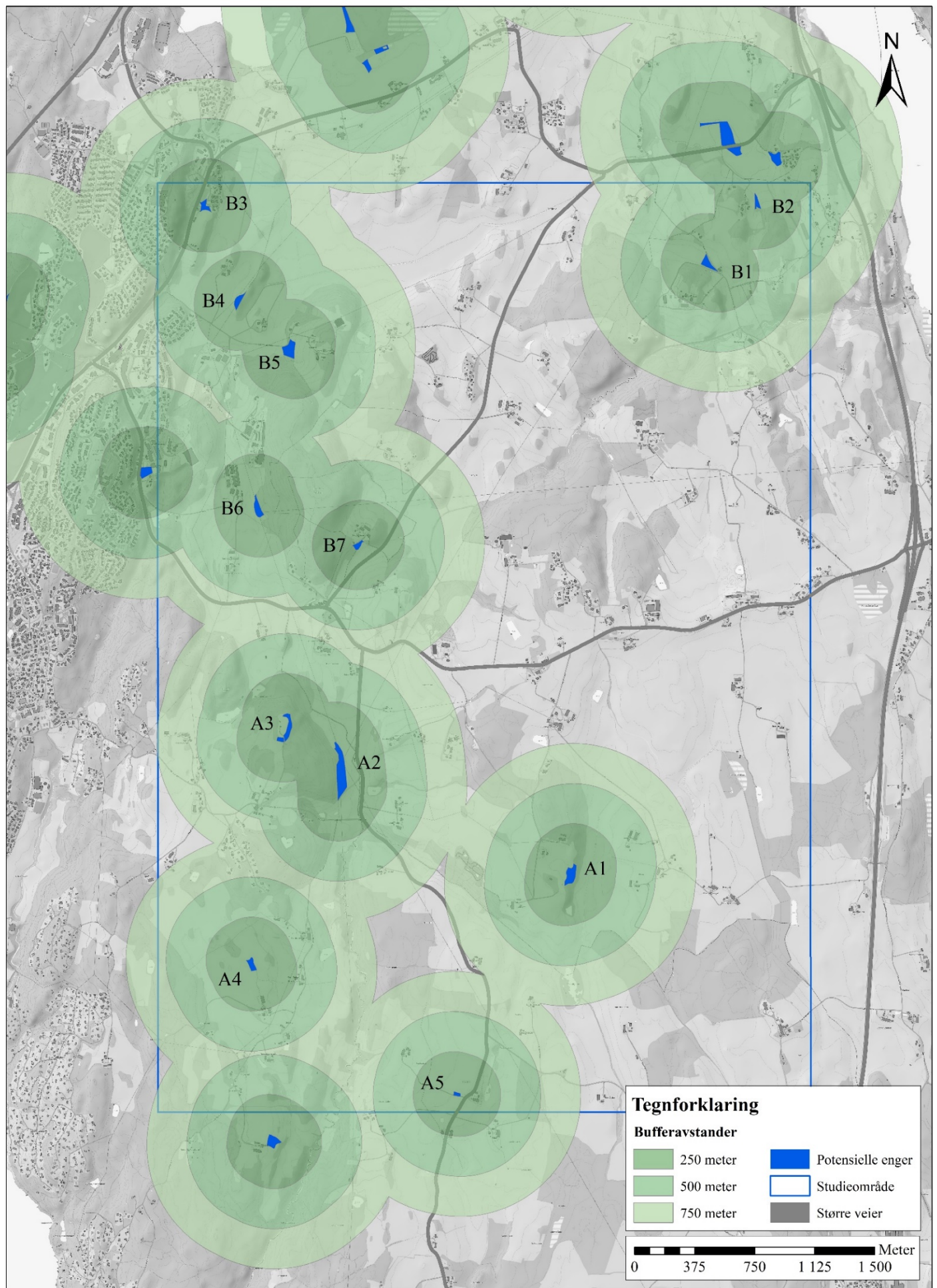
Figur 4, Bufferanalyser som viser den euklidske sammenkoblingen mellom alle patcher definert som "potensiell eng" i avstander på 250, 500 og 750 meter.
