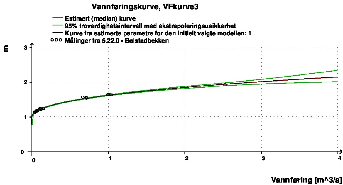
Figur 3.2. Vannføringskurve fra VFkurve3. Vannstand [m] på y-akse og vannføring [ \text{m}^3/\text{s} ] på x-aksen. Sirklene viser vannføringsmålingene, rød linje er den estimerte kurven, svart linje er kurven fra estimerte parametre for den valgte modellen. De grønne linjene representerer troverdighetsintervallet.
