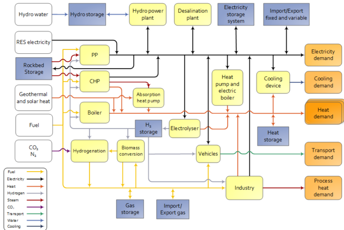
Figur 3.2: Oversikt over energisystemmodellen EnergyPLAN. Gjengitt fra EnergyPLAN – Advanced analysis of smart energy systems av H. Lund et al, 2021, Smart Energy volum 1 . Opphavsrett 2021 av Elsevier, ScienceDirect.
