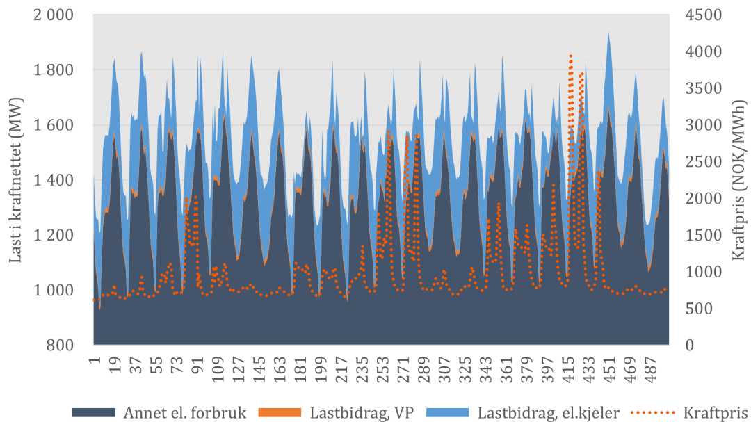
Figur 5.5: Normalår: Last i kraftnettet, med lastbidrag fra fjernvarme og annet forbruk, og kraftpriser. Pr. time gjennom treukersperiode med høyest gjennomsnittlig last (for analyseåret).
