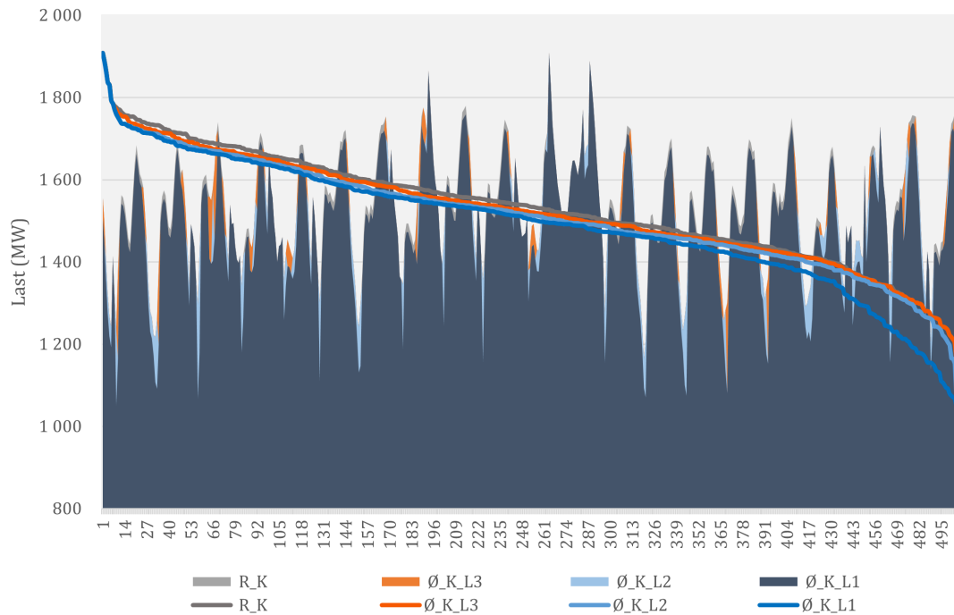
Figur 5.10: Kaldt år: Last- og varighetskurve (MW) før og etter bruk av sesonglager med økonomisk driftsstrategi.
