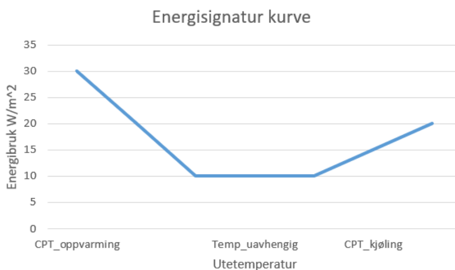
Figur 2.2: Energisignatur kurve, hvor CPT_opppvarming/kjøling viser økt behov ved lave/høye temperaturer og Temp_uavhengig er temperaturuavhengig behov.
