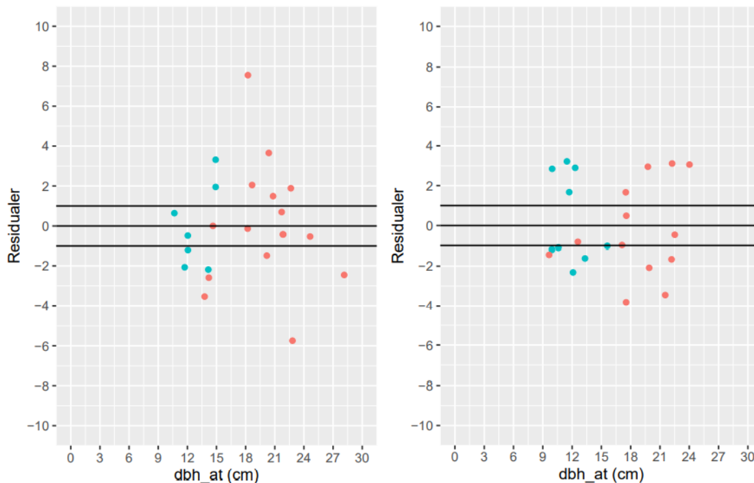
Figur 4. Residualgrafer med tynningsreaksjonen ( d_ig ) som residualer over brysthøydiameter ( dbh_at , cm), med eksempel fra bestand 1794 prøveflate 1 (t.v) og 2 (t.h). Furu er vist med rød prikker og gran med blå prikker.
