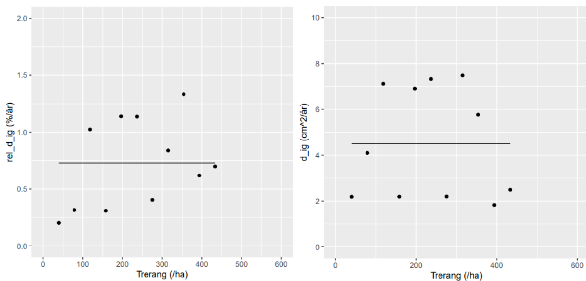
Figur 12. Lineære regresjoner med relativ tynningsreaksjon (rel_d_ig) og trerang (/ha) (t.v) og absolutt tynningsreaksjon (d_ig) og trerang (/ha) (t.h). Eksempel fra bestand 2 prøveflate 2. Linjen indikerer middelverdier for responsvariabelen.
