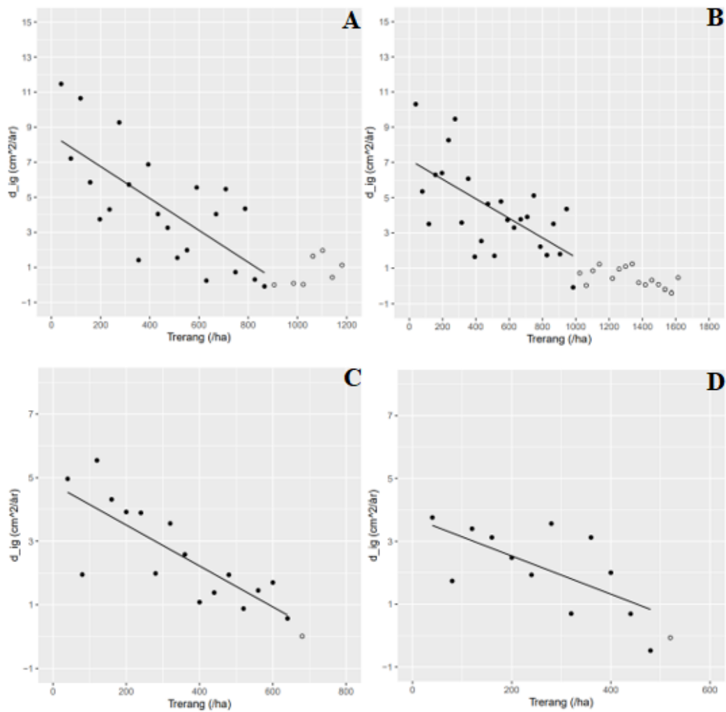
Figur 10. Resultater fra lineære regresjoner med en signifikant sammenheng mellom tynningsreaksjon ( d_{ig} ) og trerang ( /ha ). Eksempel fra bestand 1794 prøveflate 2 (A) og prøveflate 3 (B) fra barblandingsdata og bestand 3 prøveflate 1 (C) og bestand 12 prøveflate 3 (D) fra furudata. Linjen indikerer treantall/ ha med en tynningsreaksjon ( d_{ig} ) i prøveflaten. Punkter uten fyll er trær uten tynningsreaksjon ( d_{ig} ned mot 0) og er ikke inkludert i analysen.
