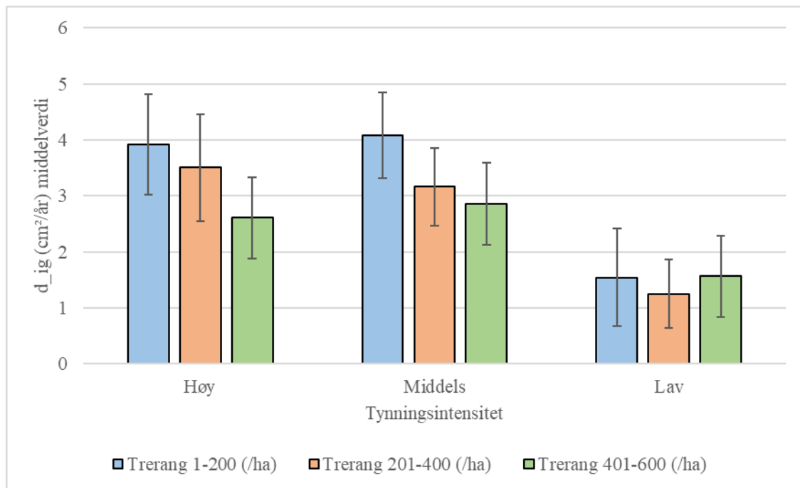
Figur 20. Middelerverdi ( \pm 95% konfidensintervall) for tynningsreaksjonen ( d_{ig} ) ved høy, middels og lav tynningsintensitet (TI) hos trær med trerang 1 - 200 ( n = 22 for høy TI, 21 for middels TI og 22 for lav TI), 201 - 400 ( n = 22 for høy TI, 21 for middels TI og 22 for lav TI) og 401-600 ( n = 16 for høy TI, 20 for middels TI og 18 for lav TI).
