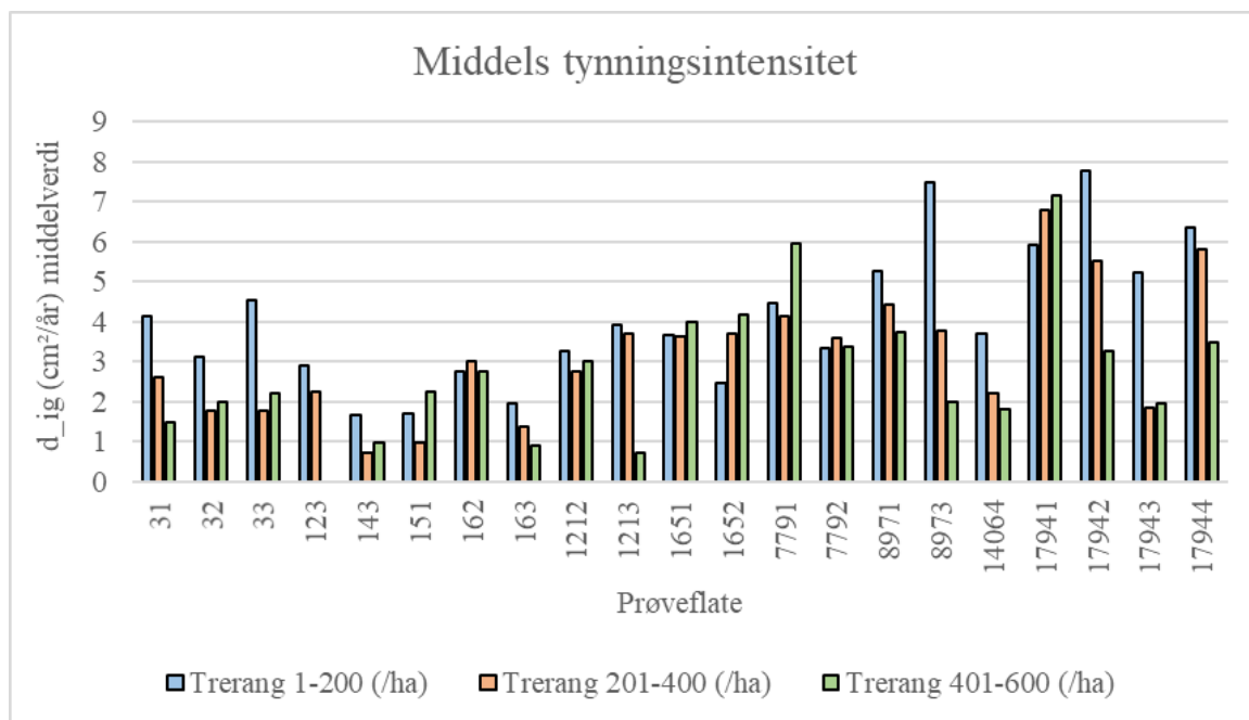
Figur 18. Middelværdier for tynningsreaksjonen ( d_{ig} ) hos trær med trerang 1 - 200, 201 - 400 og 401 - 600 (/ha) for prøveflater med middels tynningsintensitet. Bestandsnummer er etterfulgt av prøveflatenummer (siste siffer). Middelværdier for d_{ig} hos trær med trerang 401 - 600 (/ha) er kun oppgitt i prøveflater med mer enn 600 trær/ha.
