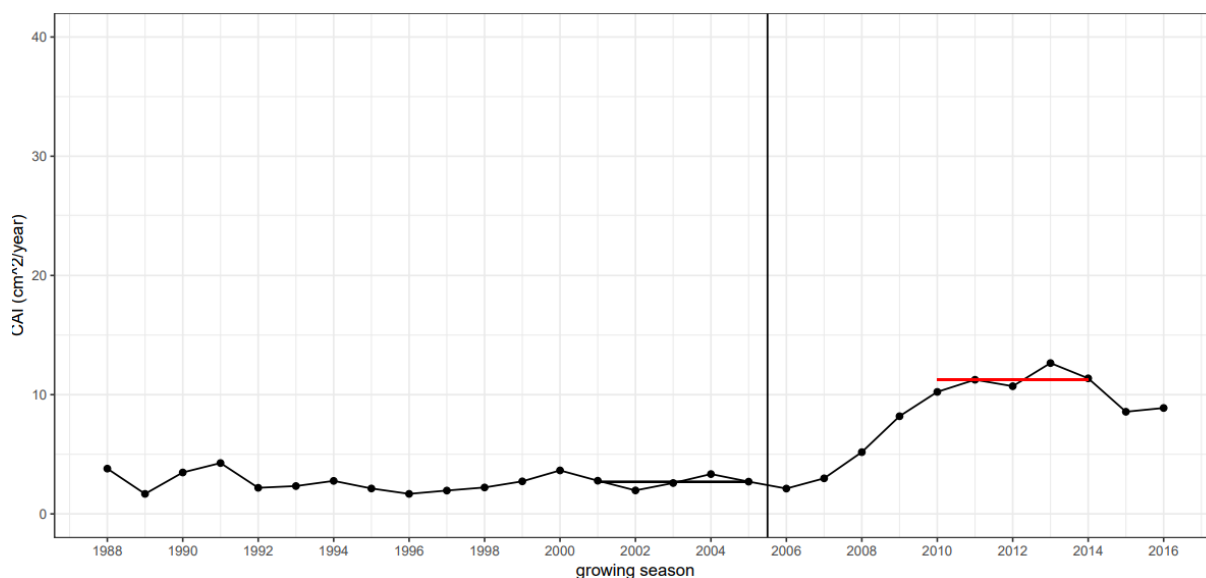
Figur 2. Grunnflatetilveksten (CAI, cm 2 per år) før og etter tynning (vertikal svart linje) for ett enkelt grantre fra bestand 779, prøveflate 1 fra barblandingsdata. Svart horisontal linje indikerer middelveiden for grunnflatetilveksten 5 år før tynning. Rød horisontal linje indikerer 5-årsperioden etter tynning med høyest grunnflatetilvekst. Figuren er hentet fra datamateriale fra undersøkelsen til Houtmeyers & Brunner (2020).
