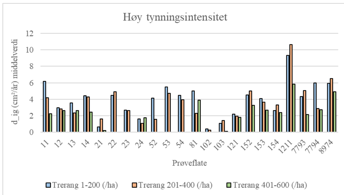
Figur 19. Middelværdier for tynningsreaksjonen ( d_{ig} ) hos trær med trerang 1 - 200, 201 - 400 og 401 - 600 (/ha) for prøveflater med høy tynningsintensitet. Bestandsnummer er etterfulgt av prøveflatenummer (siste siffer). Middelværdier for d_{ig} hos trær med trerang 401 - 600 (/ha) er kun oppgitt i prøveflater med mer enn 600 trær/ha.
