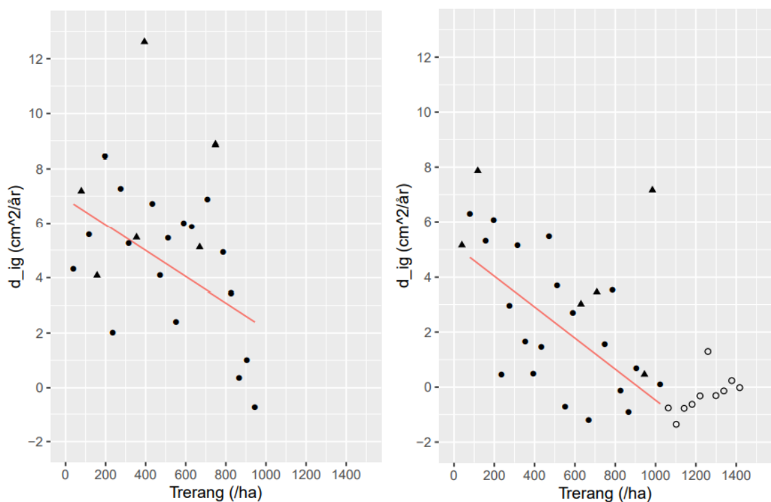
Figur 13. Lineære regresjoner med tynningsreaksjon ( d_{ig} ) og trerang (/ha) uten kantrær ved stikkveier. Eksempel fra bestand 897 prøveflate 4 (t.v) og bestand 1406 prøveflate 1 (t.h). Linjen indikerer treantall (/ha) med en tynningsreaksjon ( d_{ig} ). Kantrær ved stikkveier er markert med trekant og punkter uten fyll er trær uten tynningsreaksjon ( d_{ig} ned mot 0) og er ikke inkludert i analysen.
