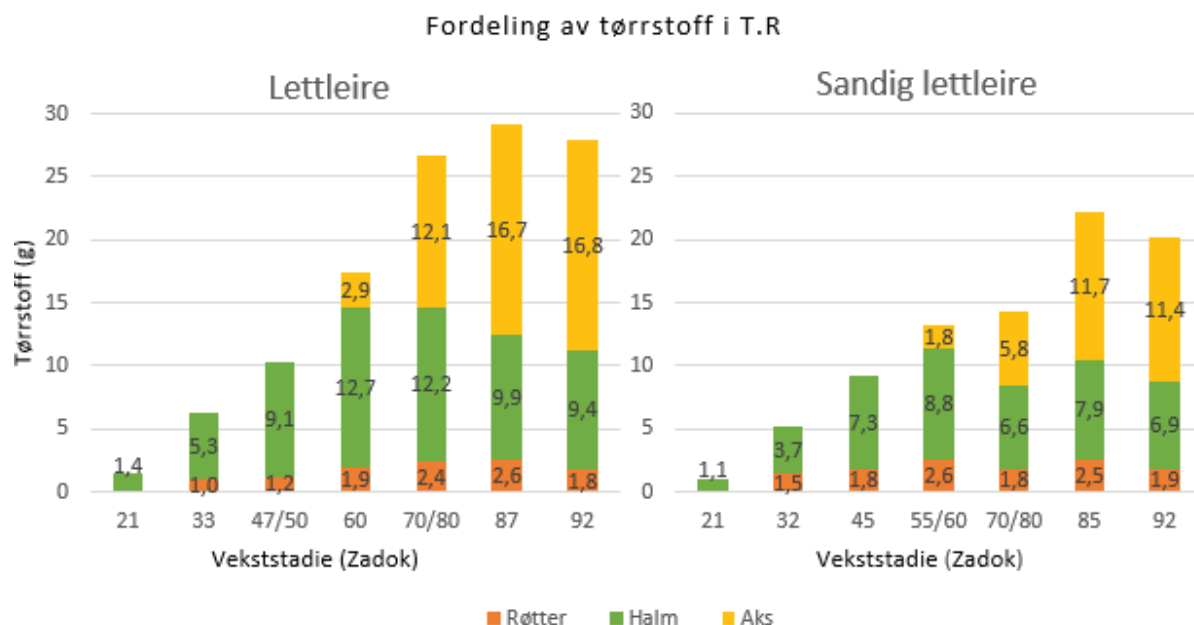
Figur 2: Fordeling av tørrmateriale i røtter, halm og aksedanning frå dag 63. X akesen er Zadok veksstadiet ved uttaket.
