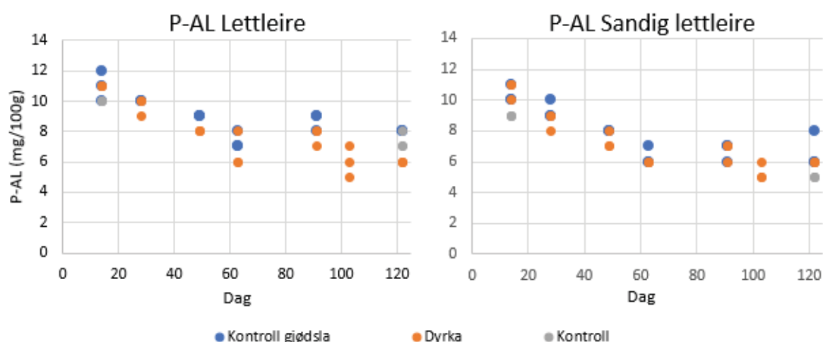
Figur 5. P-AL(mg/100g) verdier i kvar jordart og behandling ved kvart uttak
