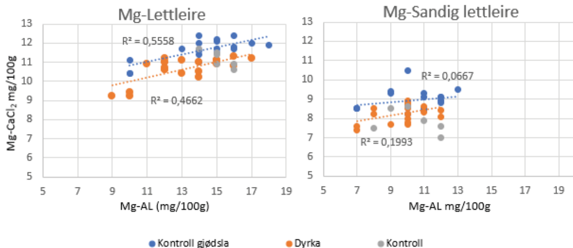
Figur 17 korrelasjonen mellom Mg-AL (x-aksen) og Mg-CaCl 2 (Y-aksen)
