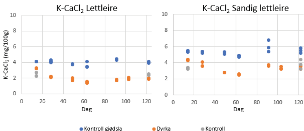
Figur 8 K-CaCl 2 (mg/100g) verdier i kvar jordart og behandling ved kvart uttak
