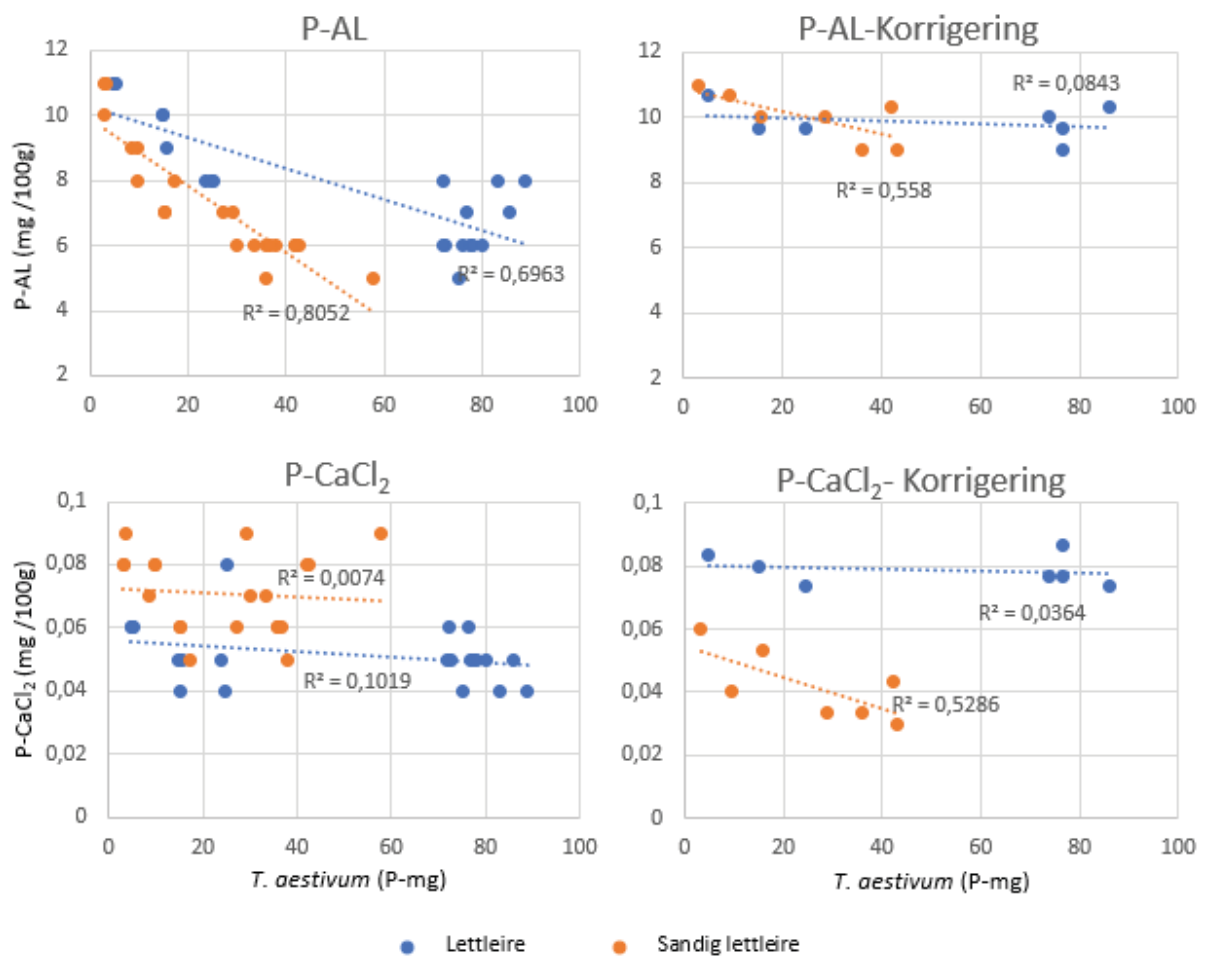
Figur 13 korrelering med P i T. aestivum og ekstraksjonsmetode på venstre side og korrigert metode til høgre
