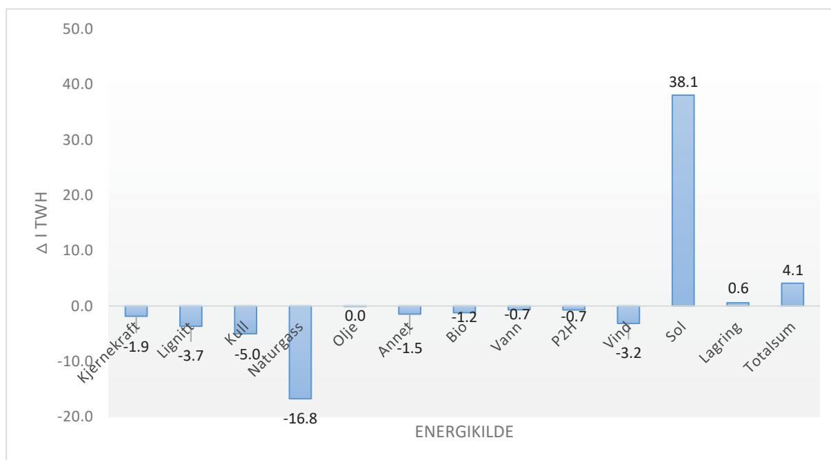
Figur 16 - Endring i kraftproduksjon ved scenario 4: Innføring av PV fra Norge, CO 2 -kvotepris på 30 euro per tonn CO 2 -ekvivalenter og investeringer i transmisjonsnettet utover det allerede planlagte..
