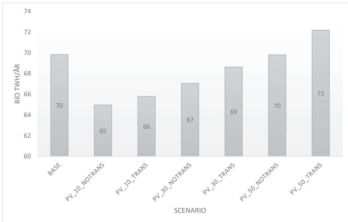
Figur 24 - Endring i kraftproduksjon fra bio i 2030 etter innføring av 38,8 TWh/år solenergi fra Norge.
