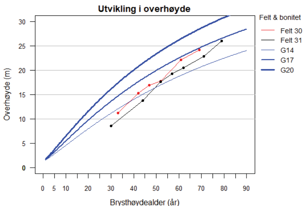
Figur 3. Utvikling i overhøyde til de 50 grøvste trær i gran-undersjiktet i felt 30 og 31 (F30 og F31). Bonitetskurver for gran (H40): G14, G17, G20.
