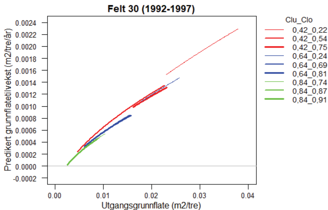
Figur 7. Predikert grunnflatetilvekst i felt 30. Kurvene viser predikert tilvekst ved ulike nivåer av CI_u og CI_o .
