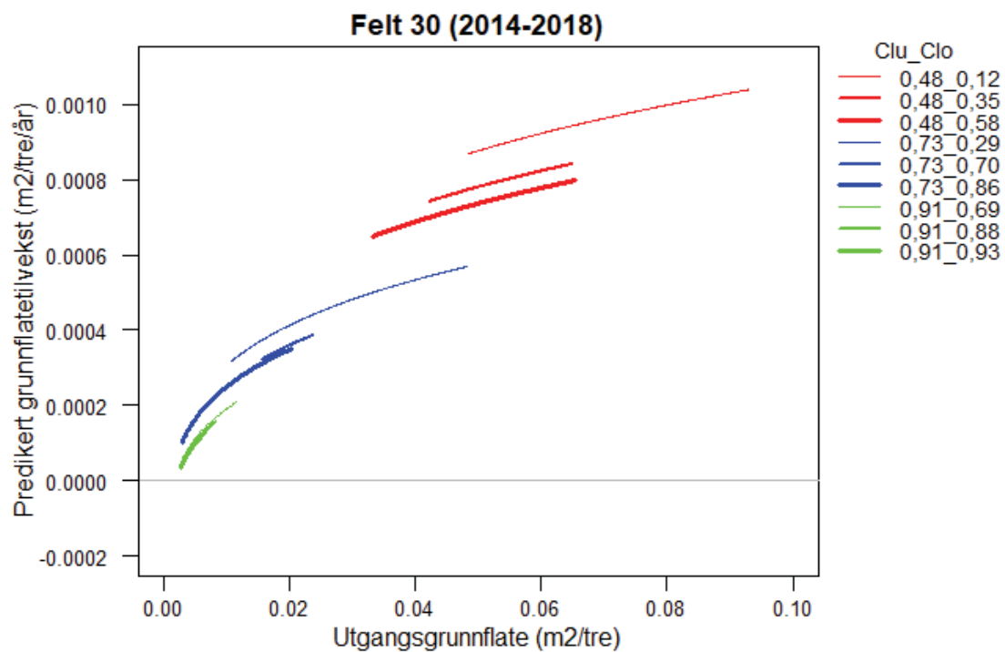
Figur 21. Predikert grunnflatetilvekst i felt 30. Kurvene viser predikert tilvekst ved ulike nivåer av CIu og CIo .
