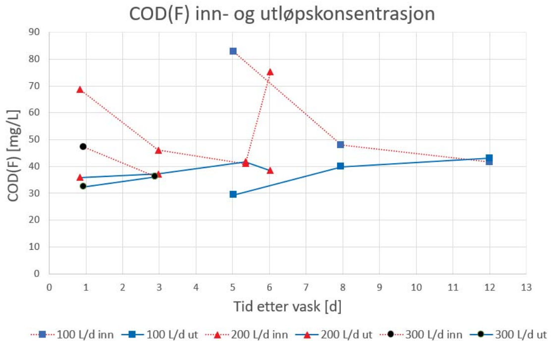
Figur 4.2: Inn- og utløpskonsentrasjoner for COD(F), gitt ved ulike hydrauliske belastninger. Blå heltrukken linje representerer utløp, mens rød stiplet innløp. Måling av drift på 100 L/d, begynte først etter 5 dager.
