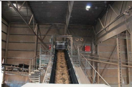
Figur 6. Skreddersøm med metallsorterer øverst.
