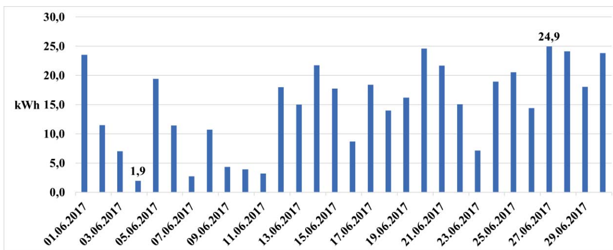
Figur 13 Solcelleproduksjon per døgn i juni
