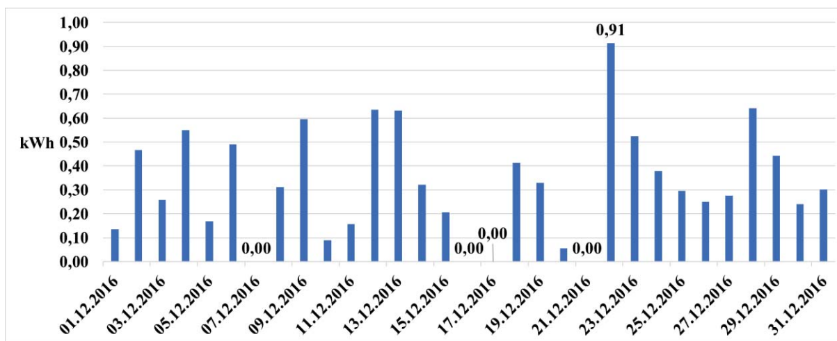
Figur 12 Solcelleproduksjon per dag i desember
