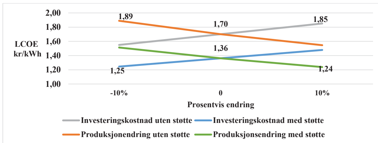
Figur 26 LCOE med en endring i investeringskostnad eller produksjon på +/- 10%, med og uten støtte fra Enova
