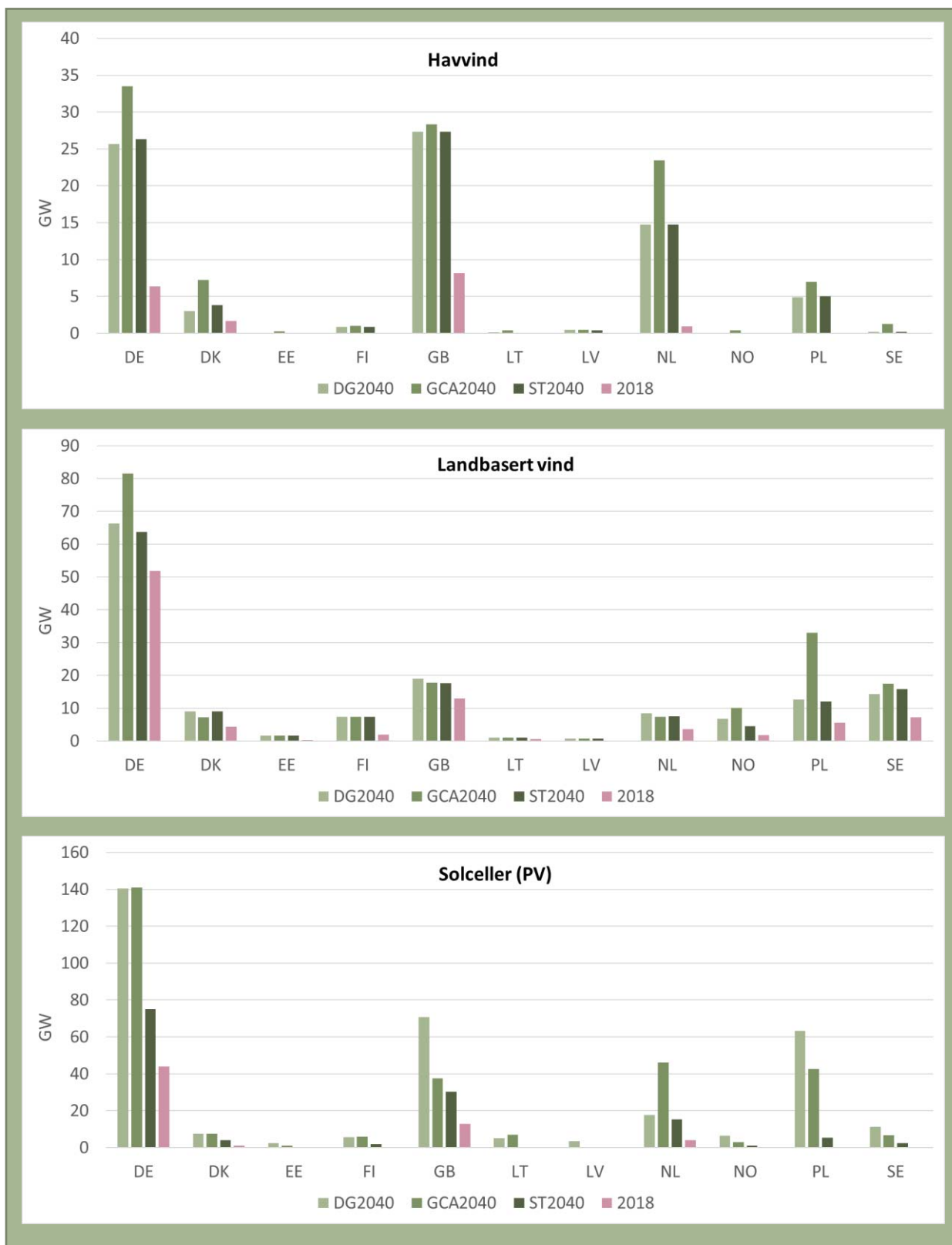
Figur 5: Installert kapasitet for havvind, landbasert vind og solceller (PV) for de analyserte scenariene. Installert kapasitet per 2018 er markert i rosa til sammenligning.
