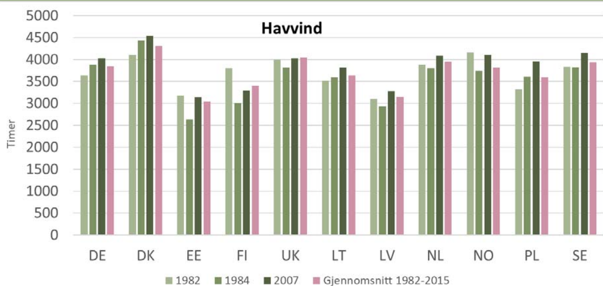
Figur 6: Fullasttimer for analyserte år og for gjennomsnitt mellom 1982-2015.
