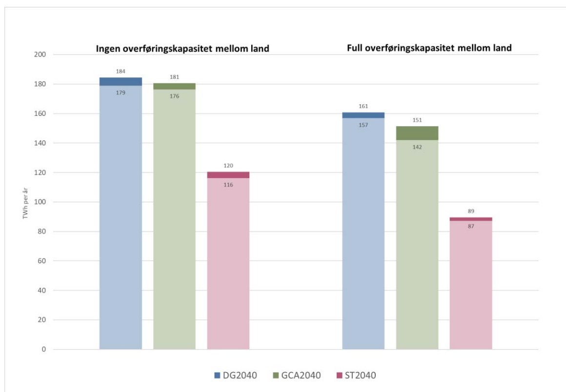
Figur 18: Daglig fleksibilitetsbehov over tre ulike scenarier for kraftsystemet i 2040.
