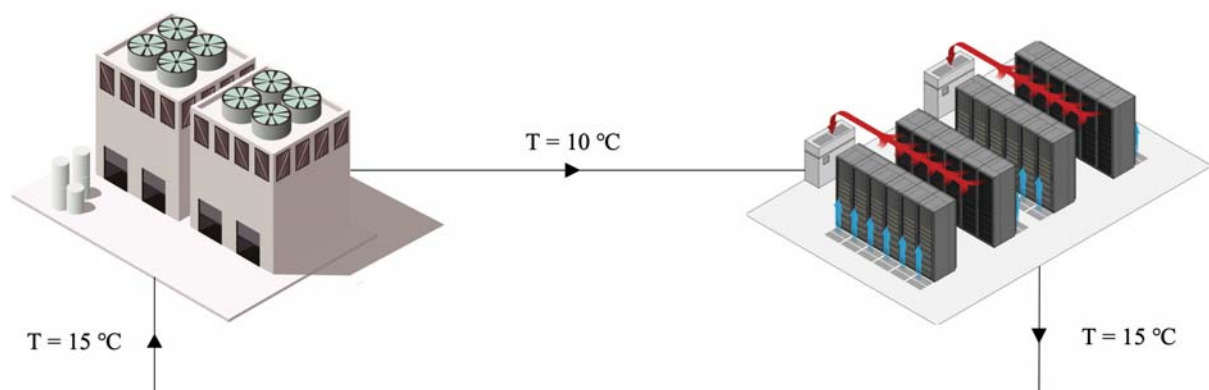
Figur 6: Prinsippskisse over dagens energisystem og kjøleløsning ved DigiPlex. Kjølemaskinene og tørrkjøleren (til venstre) leverer 10 °C til datasenteret (til høyre) som gir et temperaturløft til 15 °C før den transporteres tilbake for ny avkjøling.
