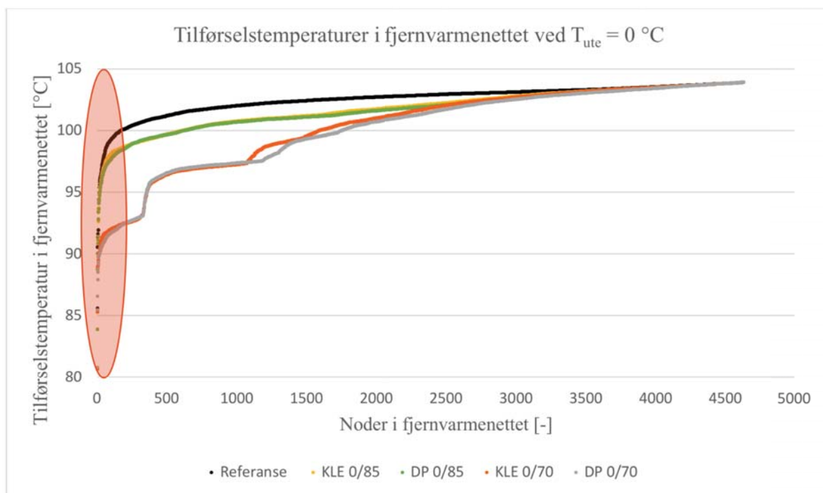
Figur 14: Illustrasjon av temperaturfall ved simuleringenes mest utsatte noder. Fenomenet illustreres i simuleringene for T_{ute} = 0\text{ °C} , men forekommer også i øvrige scenarier.
