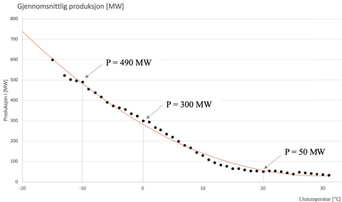
Figur 8: Driftsdata (sorte prikker) og estimert produksjonskurve (oransje kurve) for Fortums fjernvarmenett i Oslo. Effekten ved utetemperaturer på -10 °C, 0 °C og 20 °C er fremhevet for referering senere i kapitlet. (Fortum Oslo Varme, 2019)
