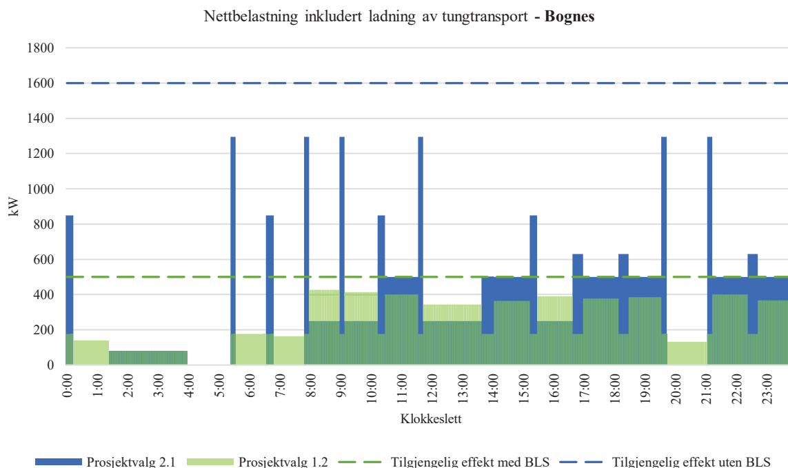
Figur 21: Nettbelastning med og uten BLS med kjøretøy er vist i figuren. Stiplede linjer representerer tilgjengelig effekt med og uten BLS, og viser hhv utnyttelse på 51% (1.2) og 33% (2.1).
