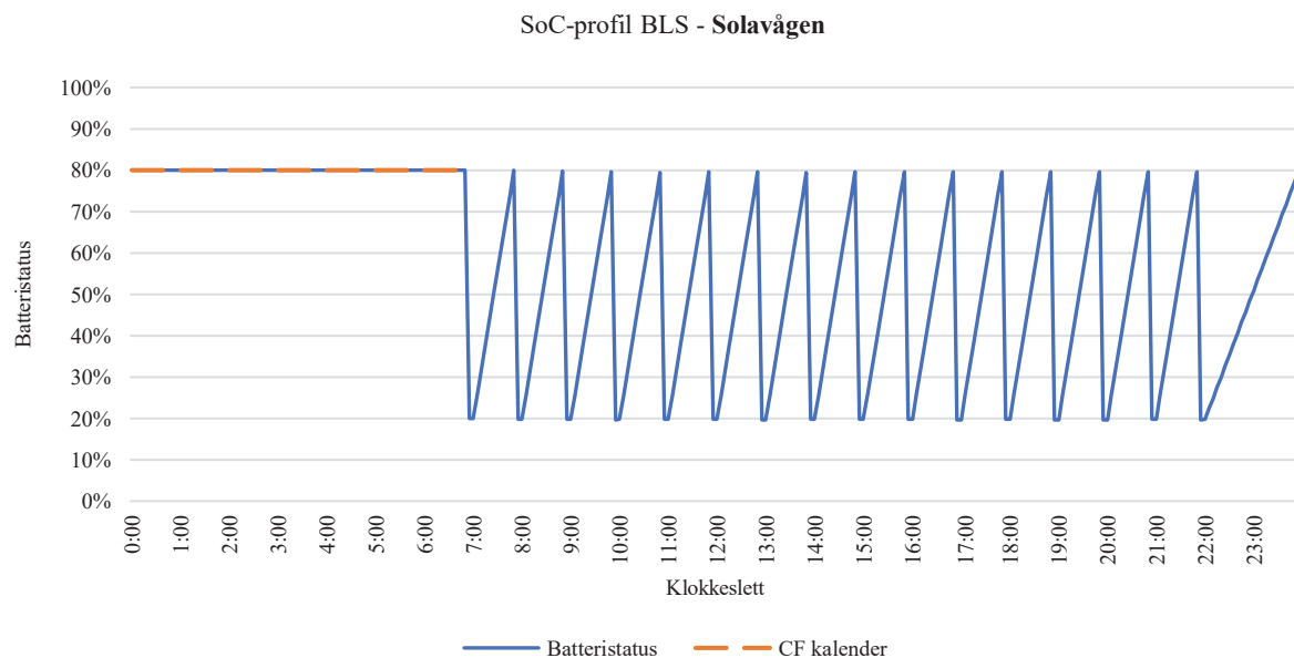
Figur 27: SoC-profil for BLS på Solavågen. BLS lagrer med en SoC på 80%, og har sykluser med dybde på 60%.
