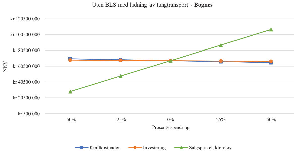
Figur 23: Følsomhetsanalyse for prosjektvalg 2.1. Parametre testet for følsomhet er kraftkostnader, nettinvestering og salgspris på el til kjøretøy. Prosjektet er mest følsomt for salgspris på el til kjøretøy.
