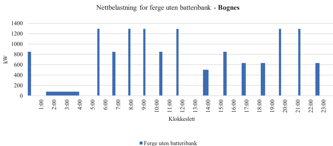
Figur 15: Netbelastning uten BLS for fergekaiaen Bognes. Effekten varierer mellom 80 og 1295 kW i løpet av døgnet. Hver søyle tilsvarer 205 kWh.
