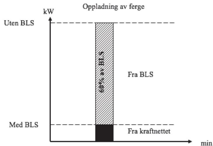
Figur 11: Skisse av batteridimensjoneringen. Det skravede området viser hvor mye batteriet må supplere fergen med. For at energiinnholdet i batteriet skal være mellom 80% og 20% ved oppladning/utladning, er det skravede området 60% av batterikapasiteten.
