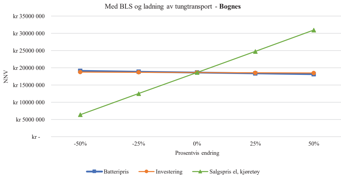
Figur 22: Følsomhetsanalyse for prosjektvalg 1.2. Parametere testet for følsomhet er batteripris, nettinvestering og salgspris på el til kjøretøy. Prosjektet er mest følsomt for salgspris på el til kjøretøy.
