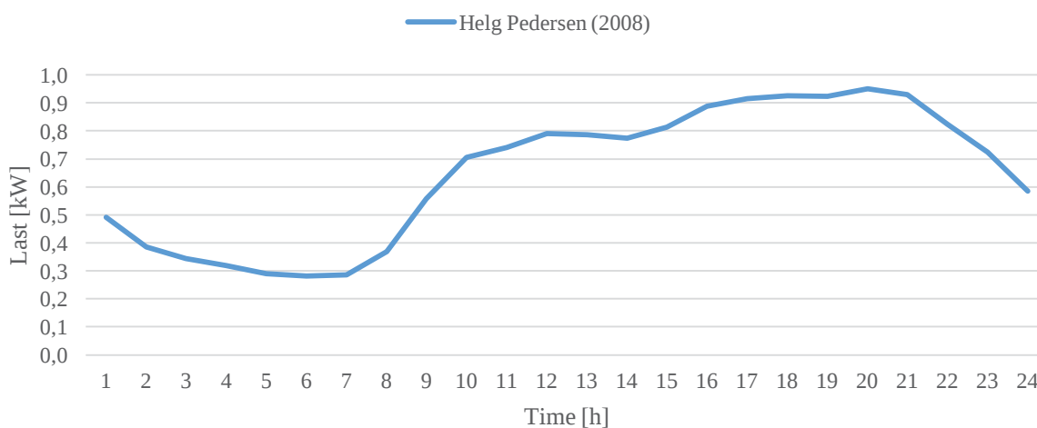
Figur 15. Lastkurver for dagen med maks last fra modell. I aggregert tilstand ved aggregering av last fra 36 leiligheter, per enhet. Opprinnelig samtidighetsfaktor. Basert på en størrelse på 90m 2 fra modellert last.
