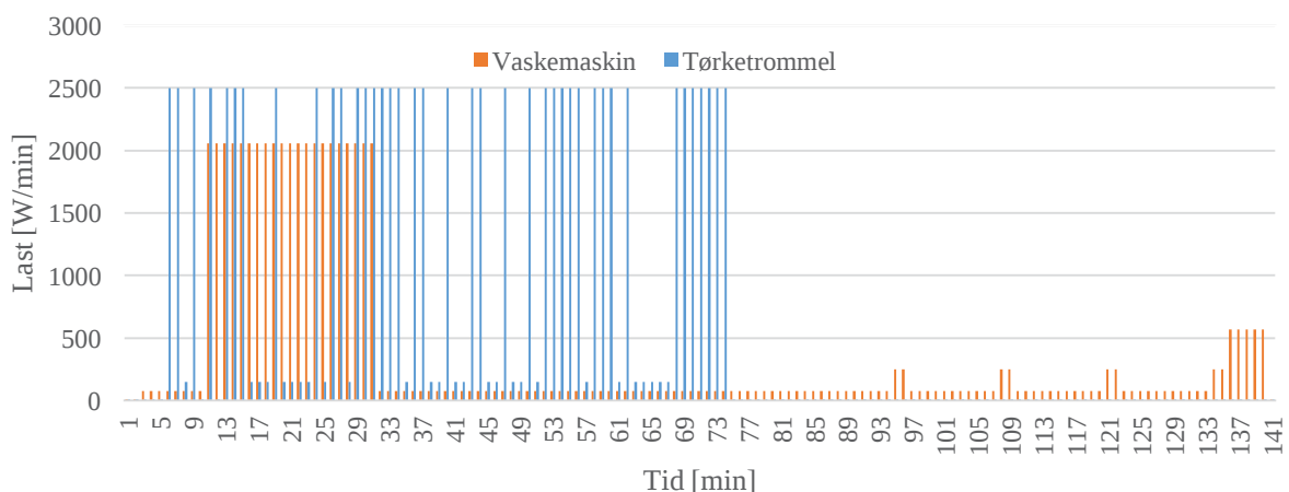
Figur 8. Empirisk effektprofil for en syklus med minuttsopløsning, vaskemaskin og tørketrommel. Hentet fra (VirginiaTech Avanced Research Institute 2013).
