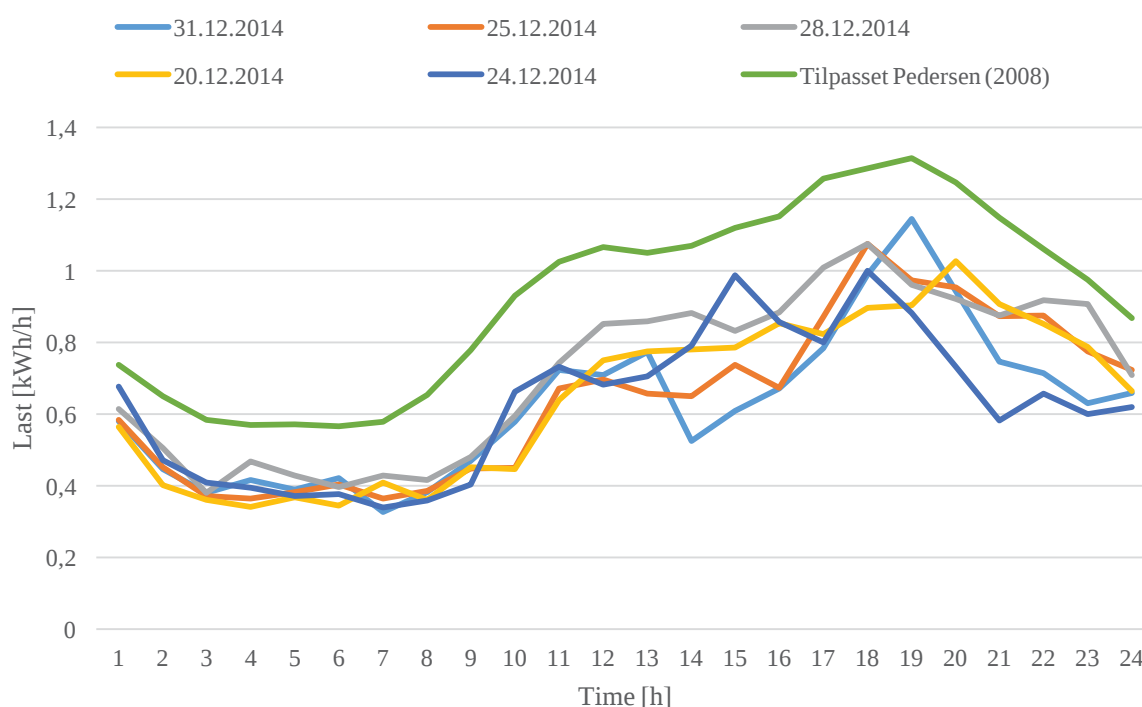
Figur 32. Lastkurver for dagen med modellert maks last og lastkurvene fra de dagene med maks last i 2014 fra reelle målinger (Ringeriks-Kraft Nett 2018). Lastkurvene er i aggregert tilstand basert på aggregering av last fra 36 leiligheter, og viser last per enhet.
