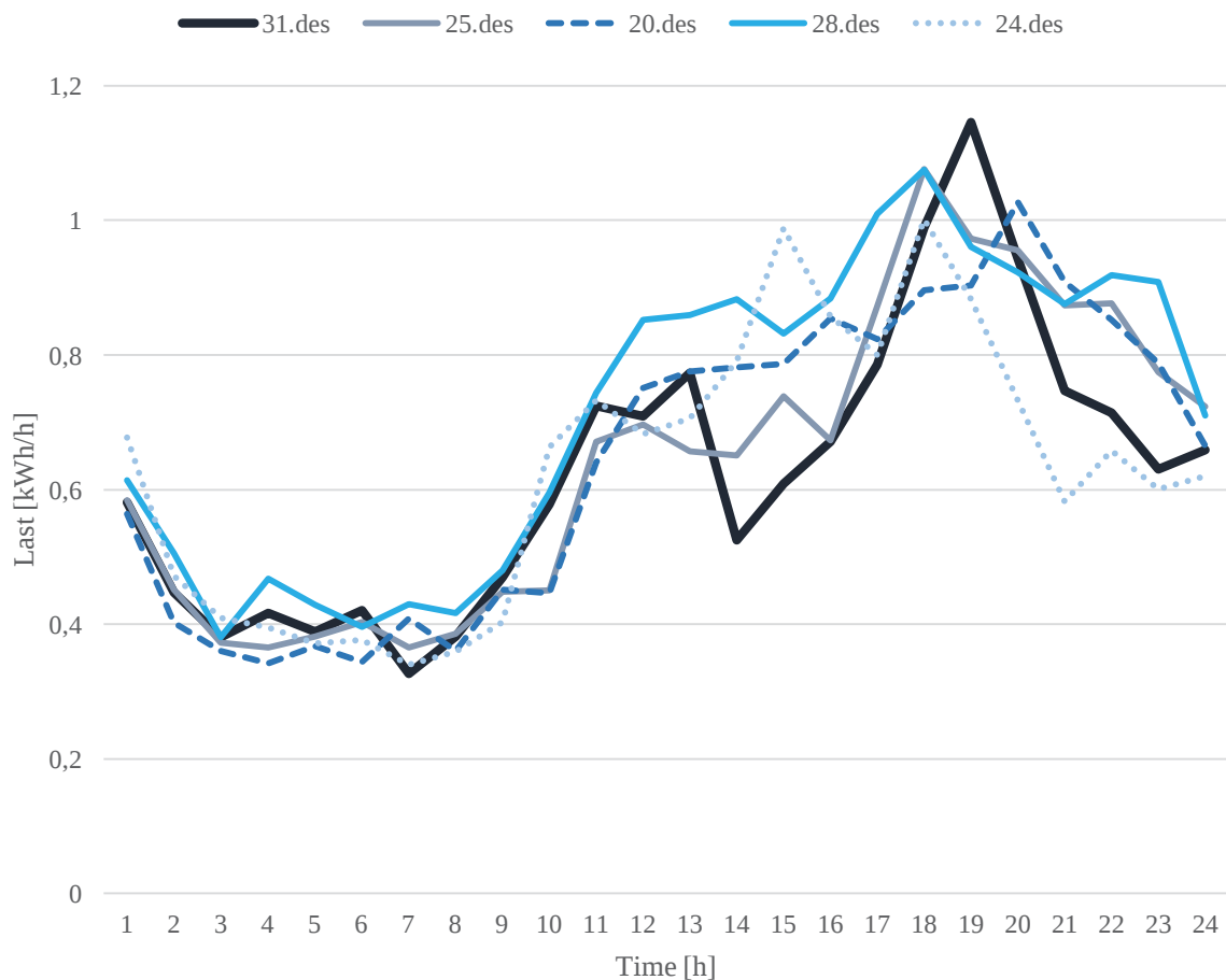
Figur 27. Lastkurver for dagene med de seks timene med maks last i 2014. 28.Desember har to av de seks høyeste timene med last som forekommer i figuren. Lastkurvene er i aggregert tilstand basert på aggregering av last fra 36 leiligheter, og viser last per enhet. Data fra (Ringeriks-Kraft Nett 2018).
