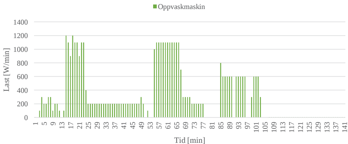
Figur 7. Empirisk effektprofil for en syklus med minuttsopløsning for oppvaskmaskin. Hentet fra (VirginiaTech Avanced Research Institute 2013).
