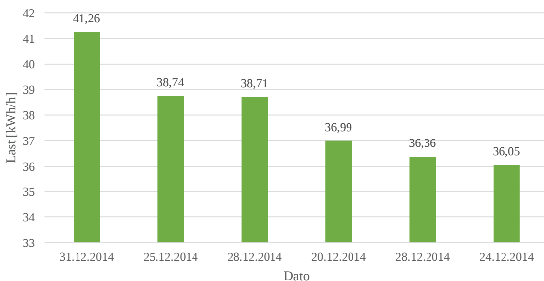
Figur 17. Seks timene med maks aggregert last per time i 2014. Reelle måledata i fra 36 leiligheter fra (Ringeriks-Kraft Nett 2018) .
