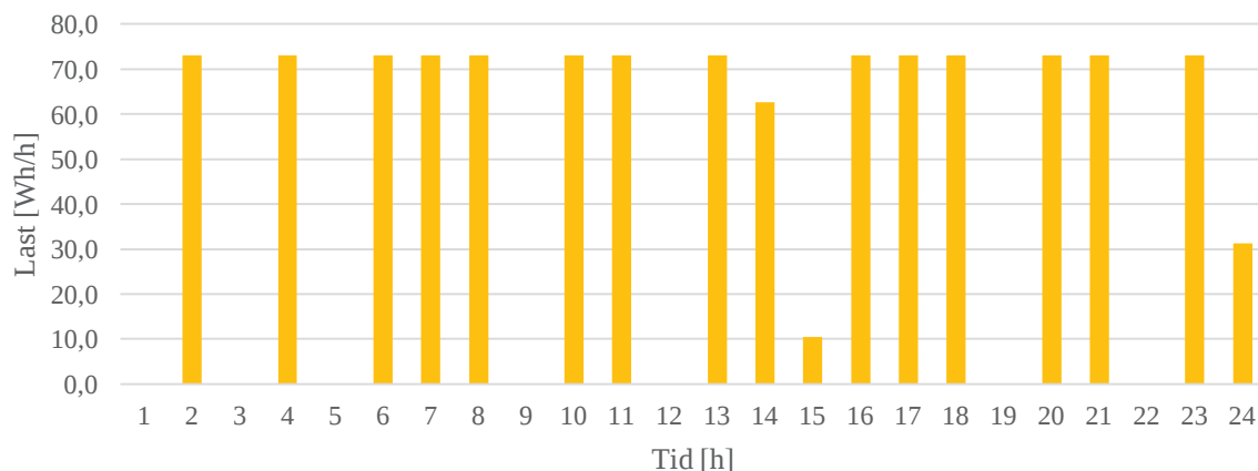
Figur 9. Simulert effektprofil gjennom et døgn med timesoppløsning for en fryser. Hentet fra (Rangøy 2013).
