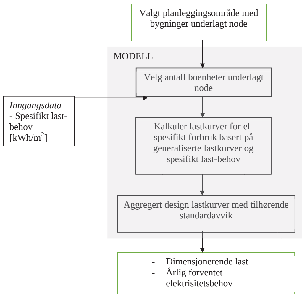
Figur 6. Fremgangsmetode for å dimensjonere last ved bruk av modell, hentet og tilpasset til denne oppgaven fra (Pedersen 2008).
