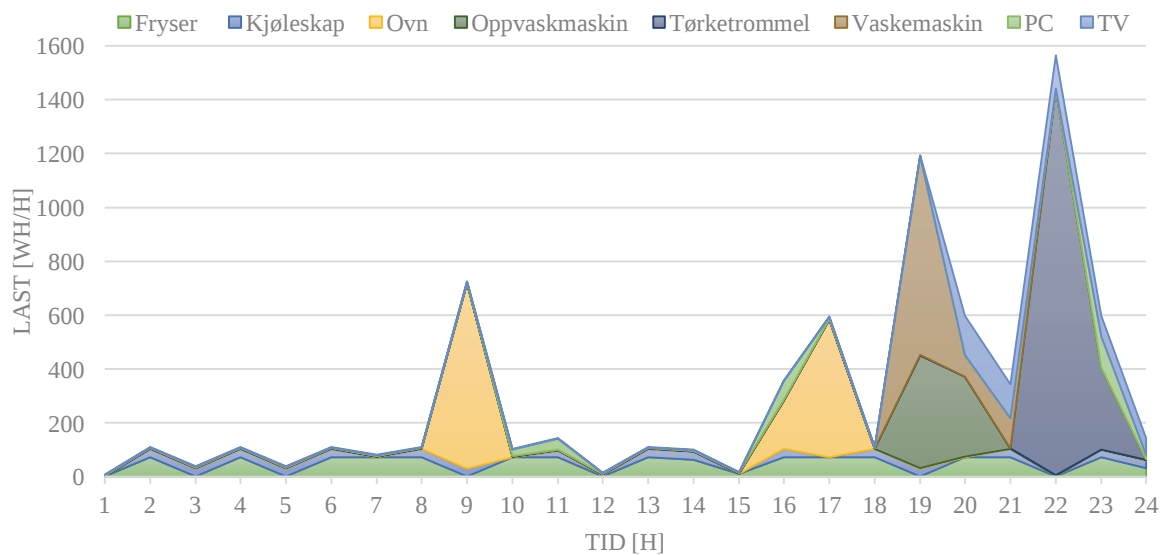
Figur 10. Simulert lastkurve. Stablet last per time for ulike husholdningsapparater i en tilfeldig husholdning på en tilfeldig dag. Data for oppvaskmaskin er empiriske, hentet fra (VirginiaTech Advanced Research Institute 2013) og øvrig materiale er simulert, og hentet fra (Rangøy 2013).
