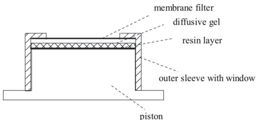
Figur 5: Skjematisk presentasjon av et tverrsnitt av en DGT-enhet (Hooda et al., 1999).
