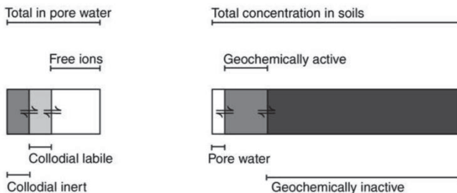
Figur 3: Skjematisk presentasjon av spormetall fordelingen i jord (høyre side) og tilstandsform i jordvæska (venstre side) (Almås & Singh, 2017).
