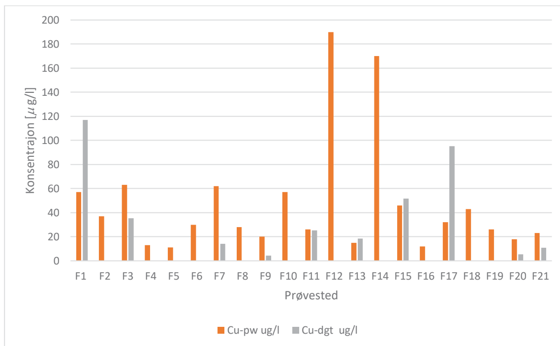
Figur 8: Sammenlikning av Cu-konsentrasjon i porevann ( \text{Cu}_{\text{pw}} ) og Cu-konsentrasjon tatt opp av DGT ( \text{Cu}_{\text{dgt}} ).
