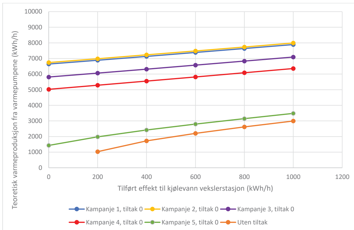
Figur 25: Teoretisk varmeproduksjon fra varmepumpene (y-akse) ved ulike tilførte energimengder til kjølevann vekslerstasjon (x-akse) ved gitte basisforutsetninger. Hver farge illustrerer teoretisk varmeproduksjon fra varmepumpene for én kampanje ved implementering av tiltak 0. De oransje punktene viser varmeproduksjonen fra varmepumpene for det nåværende systemet med de samme basisbetingelsene.
