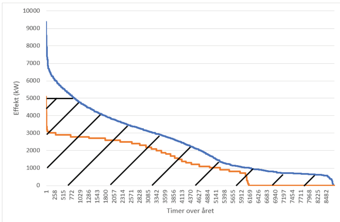
Figur 14: Varighetskurve for Sarpsborg varmesentral i 2017. Y-aksen er effekt (kW/h) og x-aksen er timer over året. Den blå linjen viser total varmeproduksjon og den oransje viser varmeproduksjonen fra varmepumpene. Det skraverte område er hva varmepumpene er dimensjonert for å dekke.
