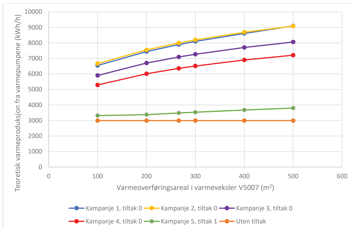
Figur 26: Teoretisk varmeproduksjon fra varmepumpene (y-akse) ved ulikt varmeoverføringsareal i varmeveksler V5007 (x-akse) ved gitte basisforutsetninger. Hver farge illustrerer teoretisk varmeproduksjon fra varmepumpene for én kampanje ved implementering av tiltak 0. De oransje punktene viser varmeproduksjonen fra varmepumpene for det nåværende systemet med de samme basisbetingelsene.
