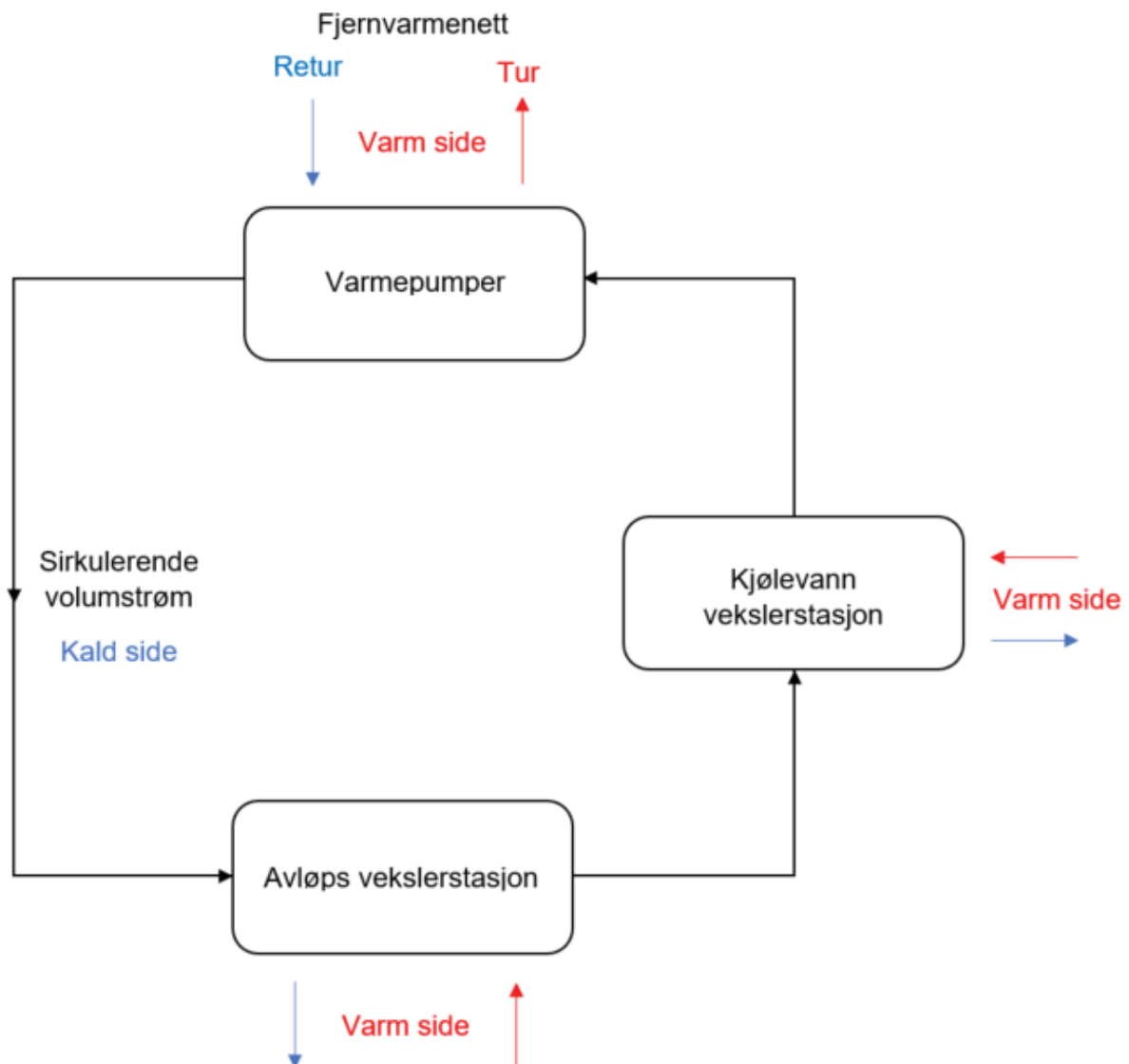
Figur 1: Prinsippskisse av det eksisterende fjernvarmesystemet. Varmepumpene utveksler tur- og returvann til fjernvarmenettet. Det sirkulerende vannet på kald side er illustrert med svarte piler og er en lukket krets som varmes opp vha. varmevekslere ved to punkter.
