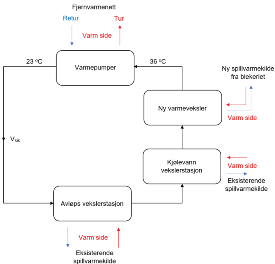
Figur 11: Prinsskisse av mulig nytt system. For å utnytte alle varmekildene best mulig er det ønskelig med lavest mulig temperatur ut av varmepumpene på kald side.
