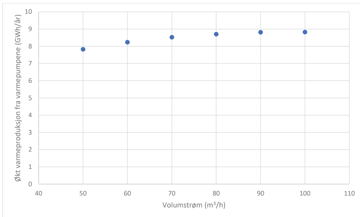
Figur 19: Økt varmeproduksjon fra varmepumpene i GWh/år langs y-aksen ved ulike konstante volumstrømnivåer i m³/h langs x-aksen.
