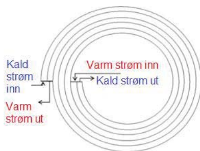
Figur 8: Prinsippskisse av en spiralvarmeveksler
