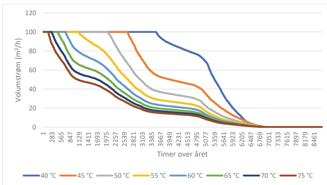
Figur 22: Volumfordeling (y-aksen i \text{m}^3/\text{h} ) over året (x-aksen i timer) ved ulike konstante temperaturer på væskestrømmen.
