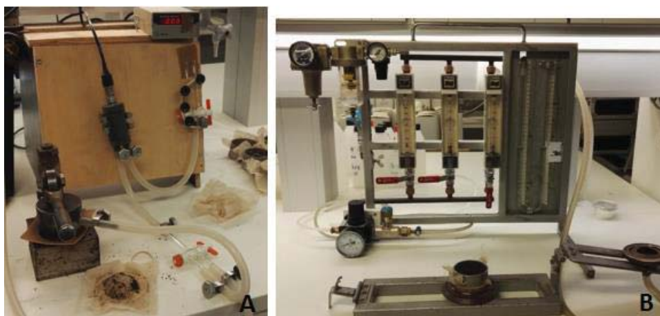
Figur 32: Luftpyknometer for måling av luftinnhold i jordprøver (A). Luftpermeameter for måling av luftstrømning gjennom jordprøver (B).
