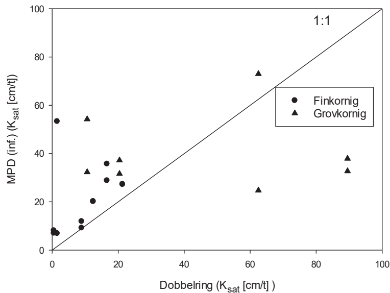
Figur 45: Korrelasjonsdiagram for MPD (inf.) og Dobbelring.
