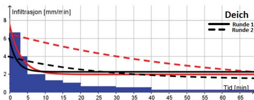
Figur 50: Infiltrasjonsrater [mm/min] målt med dobbelring. Blokk A = rød, og blokk B = svart. Nedbørintensiteter med forskjellig varighet for 20 mm regn, vises i blått. Hvert trappetrinn tilsvarer en bestemt nedbørintensitet og et regn på 20 mm. Kapasitet_A og B: 200 års regn med 9 min varighet.
