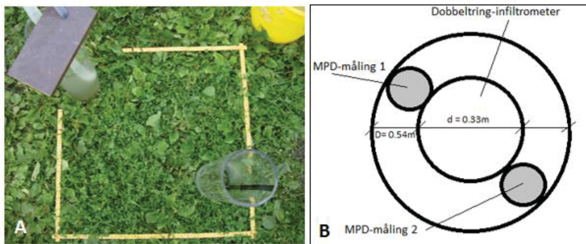
Figur 23: Infiltrasjonstester på overflaten. Forsøksrute på 60cm*60cm (A). Plassering av MPD-rør i forhold til dobbelring-infiltrimeter (B).
