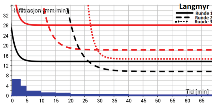
Figur 53: NB! Legg merke til at y-aksen er i annen størrelsesorden enn for de andre lokalitetene. Kapasitet_A og B: Alle regn.
