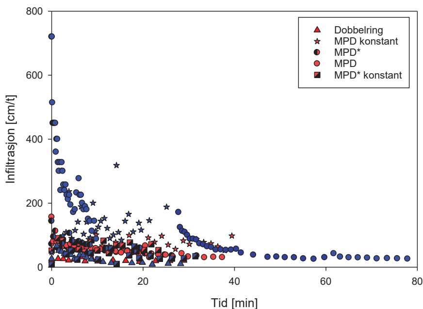
Figur I.7. 1: Infiltrasjonstester gjennomført på overflaten i Kuba, med fargekoder; rød (blokk A) og blå (blokk B). Infiltrasjon [cm/t] er plottet mot tid [min]. Forsøk med MPD-infiltrometeret med konstant trykkehøyde er inkludert, med og uten fuktet profil, hhv. MPD* konstant og MPD konstant.
