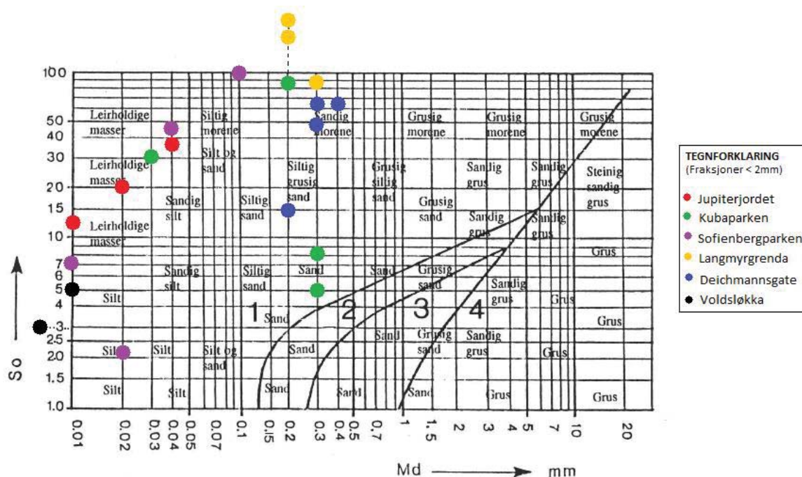
Figur P.4. 1: Vurdering av infiltrasjonsevne i et infiltrasjonsdiagram (VA-miljøblad nr. 59, 2016). Fraksjoner < 2mm er vurdert ved bestemmelse av midlere kornstørrelse ( M_d ) [mm] og sorteringsgrad ( S_o ).
