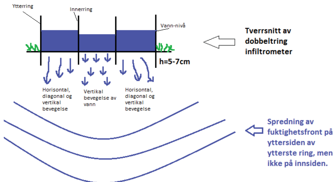
Figur 16: Tverrsnitt av dobbelring-infiltrrometer. Vannstrømning er tegnet inn, og viser hvordan man får vertikal bevegelse i inner-ringene, mens horisontal- og vertikal bevegelse i ytterringen.
