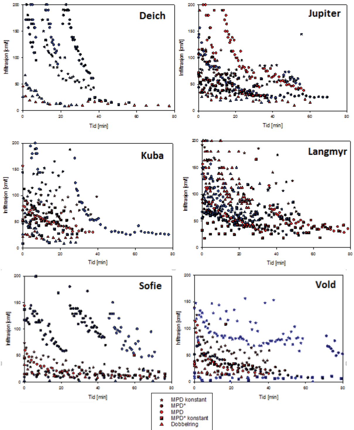
Figur M.2. 1: Infiltrasjonstester gjennomført på overflaten ved de ulike lokalitetene (fargekoder; rød =blokk A og blå =blokk B). Infiltrasjon [cm/t] er plottet mot tid [min]. MPD konstant betyr forsøk med MPD-infiltrrometeret med konstant vannnivå (trykkhøyde). * betyr at bakken var fuktet (opptil 1 time) før start av forsøket.
