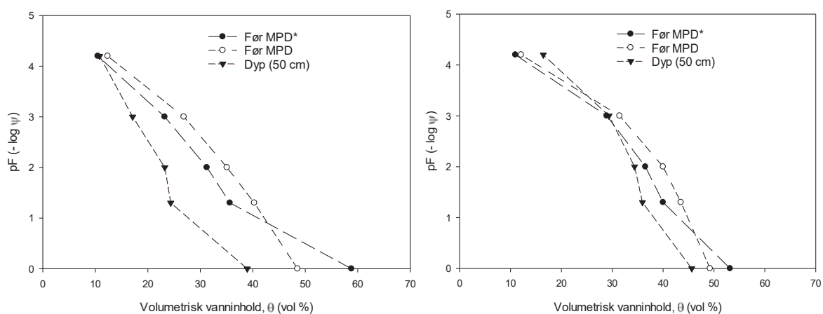
Figur K.6. 1: pF-kurver fra Sofie. Blokk A til venstre og blokk B til høyre. * betyr at bakken var fuktet (opptil 1 time) før start av forsøk.
