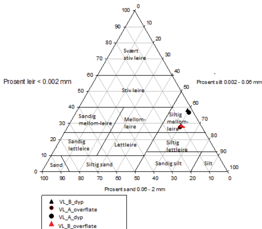
Figur L.3. 1: Jordartstrekant etter Sveistrup og Njøs (1984) for klassifisering av mineraljord (<2mm). Jordprøver fra overflaten og dypet på Voldsløkka (VL) er markert (blokk A og B).
