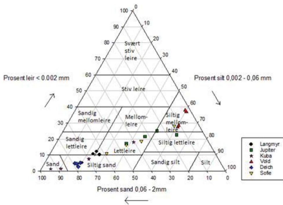
Figur 42: Jordartstrekant etter Svestrup og Njøs (1984) med inntegnet jordprøver fra overflate og dypet (blokk A og B) for alle lokaliteter.
