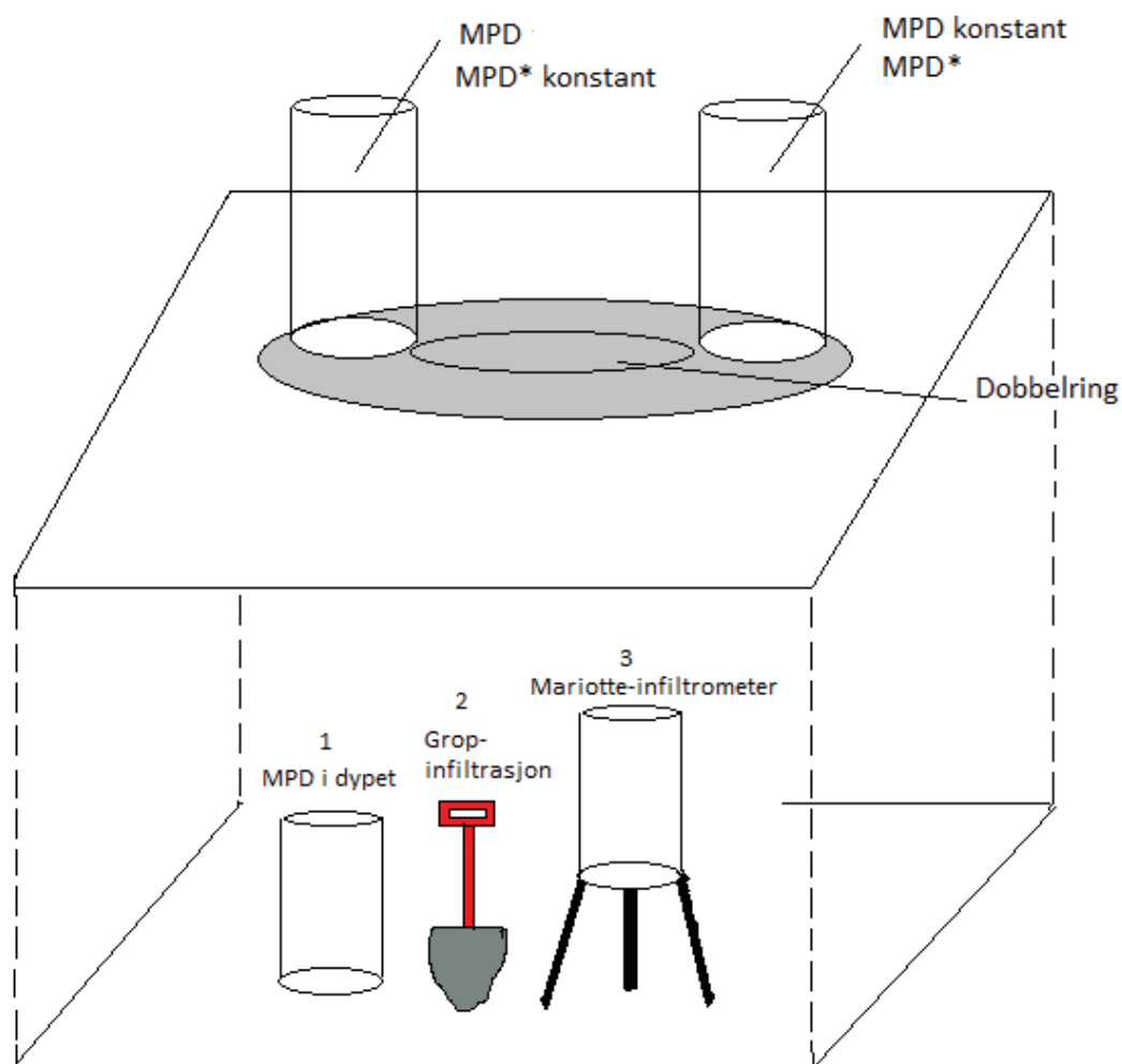
Figur D. 1: Prinsippskisse for forsøk gjennomført i en blokk (overflate og dyp). På overflaten gjennomføres forsøk med MPD-infiltrrometer (synkende og konstant vannivå) og Dobbelring-infiltrrometer. * betyr at bakken var fuktet (opptil 1 time) før start av forsøket startet. I dypet gjennomføres "MPD i dypet" etterfulgt av "Grop-infiltrasjon" og forsøk med "Mariotte-infiltrrometer».
