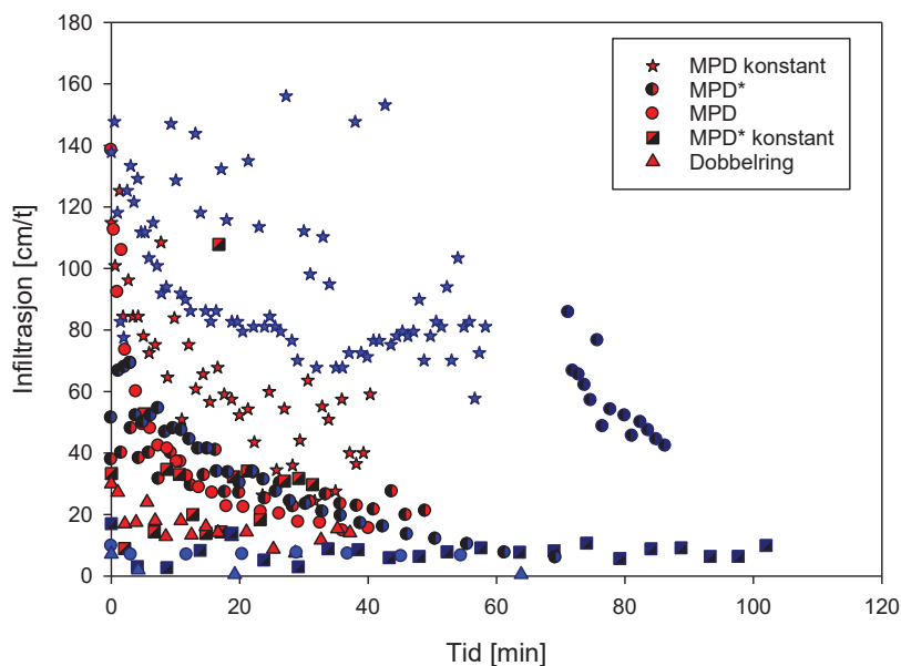
Figur L.7. 1: Infiltrasjonstester gjennomført på overflaten på Vold, med fargekoder; rød (blokk A) og blå (blokk B). Infiltrasjon [cm/t] er plottet mot tid [min]. Forsøk med MPD-infiltrrometeret med konstant trykkehøyde er inkludert, med og uten fuktet profil, hhv. MPD* konstant og MPD konstant.
