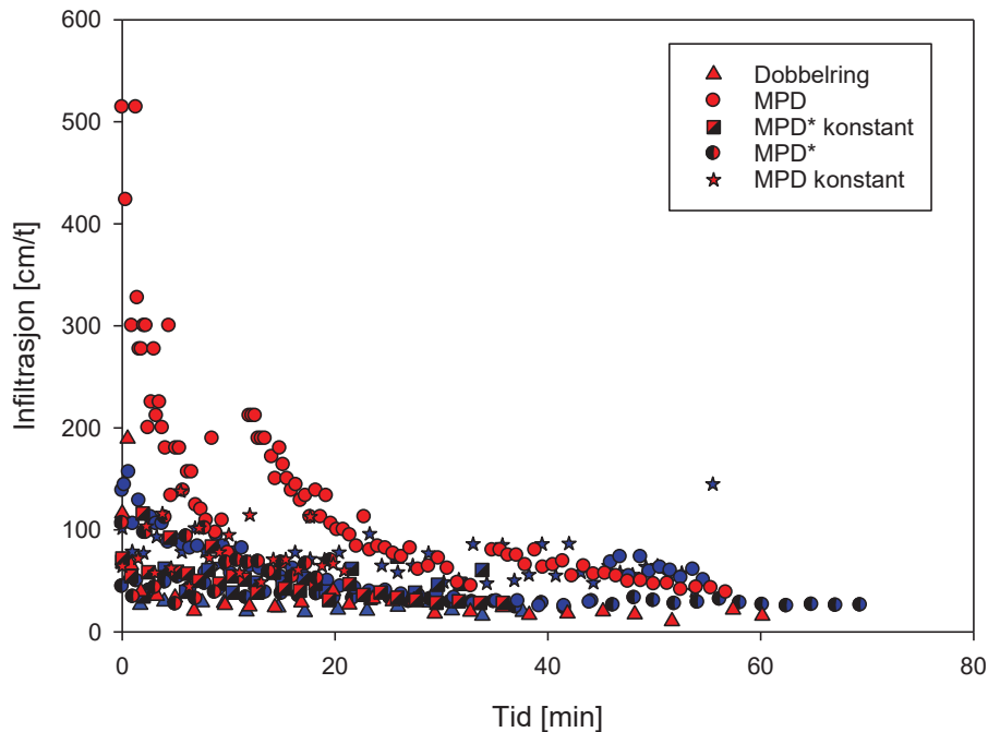
Figur H.7. 1: Infiltrasjonstester gjennomført på overflaten på Jupiter, med fargekoder; rød (blokk A) og blå (blokk B). Infiltrasjon [cm/t] er plottet mot tid [min]. Forsøk med MPD-infiltrrometeret med konstant trykkehøyde er inkludert, med og uten fuktet profil, hhv. MPD* konstant og MPD konstant.
