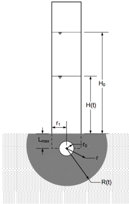
Figur S. 1: Tverrsnittprofil av MPD-rør hvor viktige parametere er oppført. H_0 representerer vannhøyde i MPD-røret ved start. H(t) representerer vannhøyde i MPD-røret ved tiden t . L_{\text{max}} angir hvor dypt ned i jorda MPD-røret er banket ned. R(t) representerer radius til fuktighetsfronten under infiltrasjonsforsøket. r_1 er indre radius til MPD-røret, og r_0 er en ekvivalent «source radius». r_0 representerer radiusen til en sfære med et overflateareal som er likt overflatearealet til den sirkulære overflaten til bunnen av MPD-røret (Nesting, 2007).
