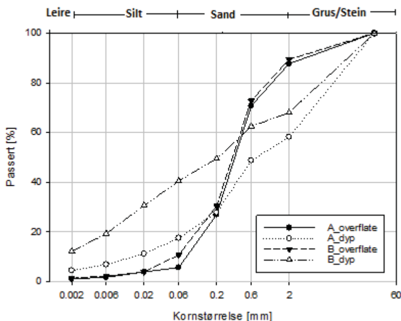
Figur I.4. 1: Kornfordelingskurver for jordprøver fra Kuba (overflate og dyp, blokk A og B). Passert [%] angir vektprosent av total jordprøve som passerer en sikt ved forskjellige siktåpninger (kornstørrelser).
