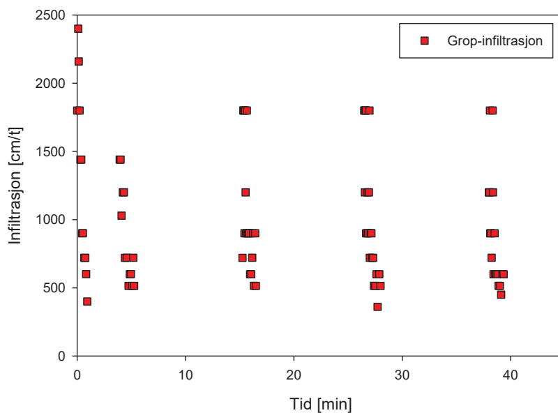
Figur G.7. 2: Grop-infiltrasjon gjennomført i dypet i Deich, med fargekoder; rød (blokk A) og blå (blokk B) (resultater fra blokk B mangler da infiltrasjonsevnen var så høy, slik at ikke sammenhengende vannhøyde og tid kunne noteres). Infiltrasjon [cm/t] er plottet mot tid [min]. «MPD i dypet» kunne ikke gjennomføres pga. steinholdg grunn. Mariotte-infiltrometeret var uegnet til bruk på jordart med stor hydraulisk ledningsevne, da infiltrasjonsraten var så høy at avlesning på Mariotte-infiltrometeret ikke var mulig.
