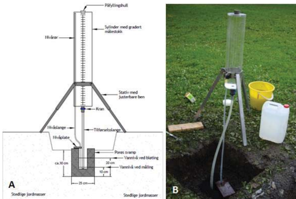
Figur 19: Oppsett av Mariotte-infiltrometer (A) (Bioforsk, 2009). Mariotte-infiltrometer i felt (B).
