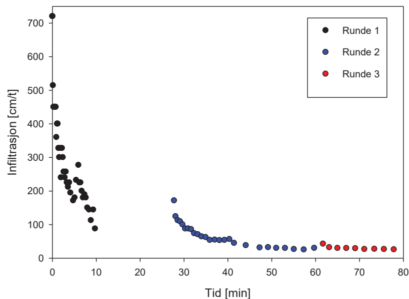
Figur 25: Resultater fra forsøk med MPD-infiltrrometer (runde 1, 2 og 3) fra Kuba, blokk B. Grafen viser hvordan infiltrasjonshastigheten stabiliserer seg med tiden. Etter 50 min (slutten av runde 2) er infiltrasjonsraten tilnærmet stabil. Det er en liten økning ved oppstart av runde 3, da det går litt tid mellom de to rundene. Fra feltnotatene er det notert at det er 18 min mellom runde 1 og 2. Ved slutten av runde 3 er K_{sat} stabil (25-26 cm/t).
