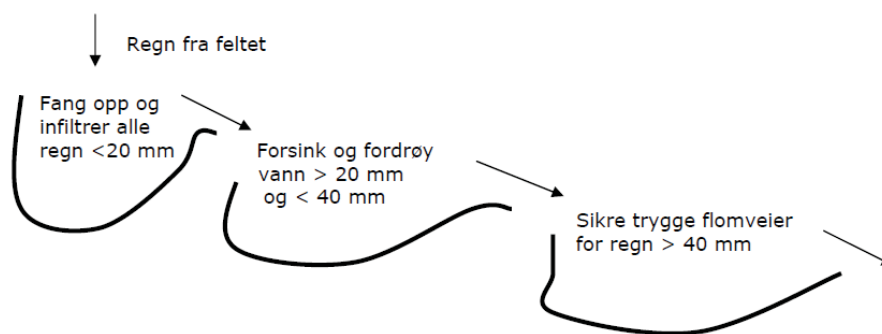
Figur 2: Tretrinnsstrategi for håndtering av nedbør. 1) Fang opp og infiltrer små regn. 2) Forsink og fordrøy større regn. 3) Sikre trygge flomveier ved styrtregn. Tallene er eksempler og må tilpasses lokalt (Lindholm et al., 2008).
