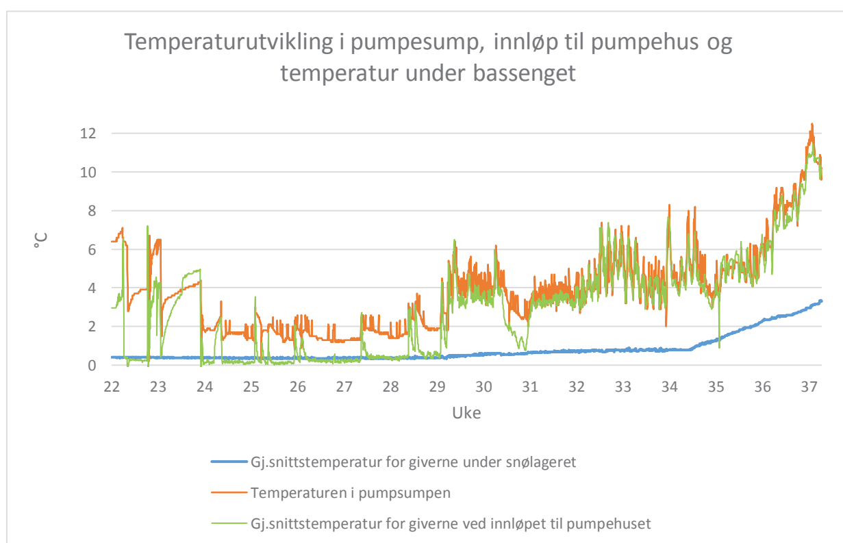
Figur 27 Utvikling av temperatur i pumpesump, gjennomsnittstemperaturen til temperaturfølerne ved innløpet til pumpehus og i gjennomsnittstemperaturen fra de fire temperaturfølerne som ligger 0,5 meter under bassenget gjennom driftsperioden
