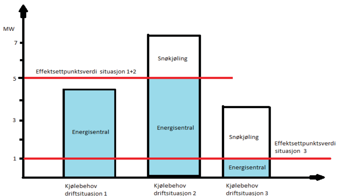
Figur 17 Effektbehov og effektsettpunktsverdi
