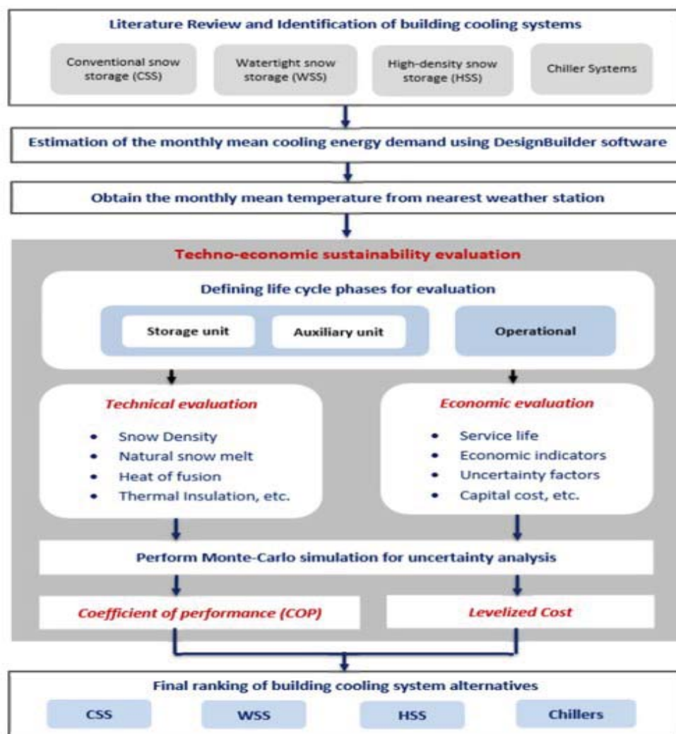
Figur 6 Foreslått rammeverk for bærekraftig evaluering av teknoøkonomisk ytelse for kjølesystemer i bygninger
