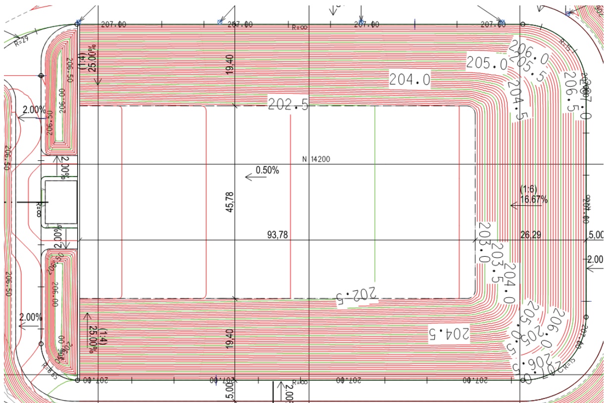
Figur 43 viser geometrien til det termiske snølageret. Bassenget har et fall på 0,5% mot pumpestasjonen.
