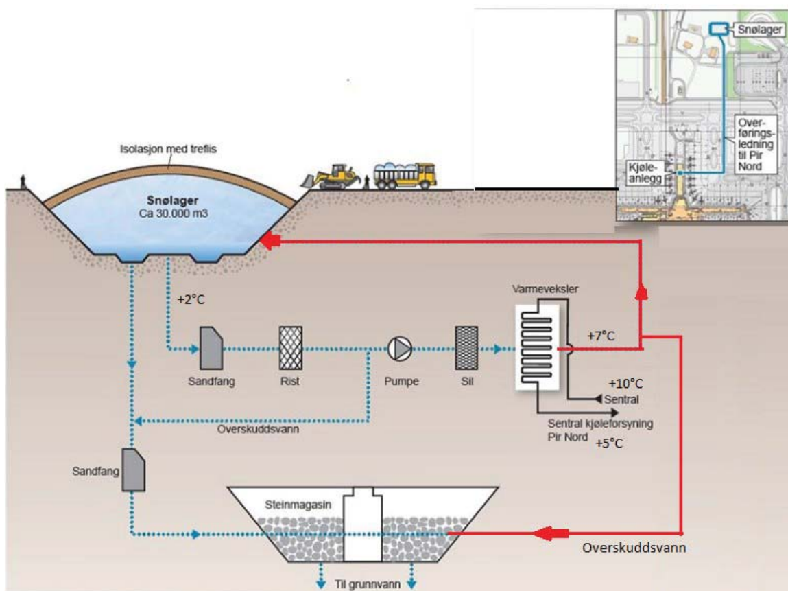
Figur 1 Prinsippskisse snøkjøleanlegg (Børresen)
