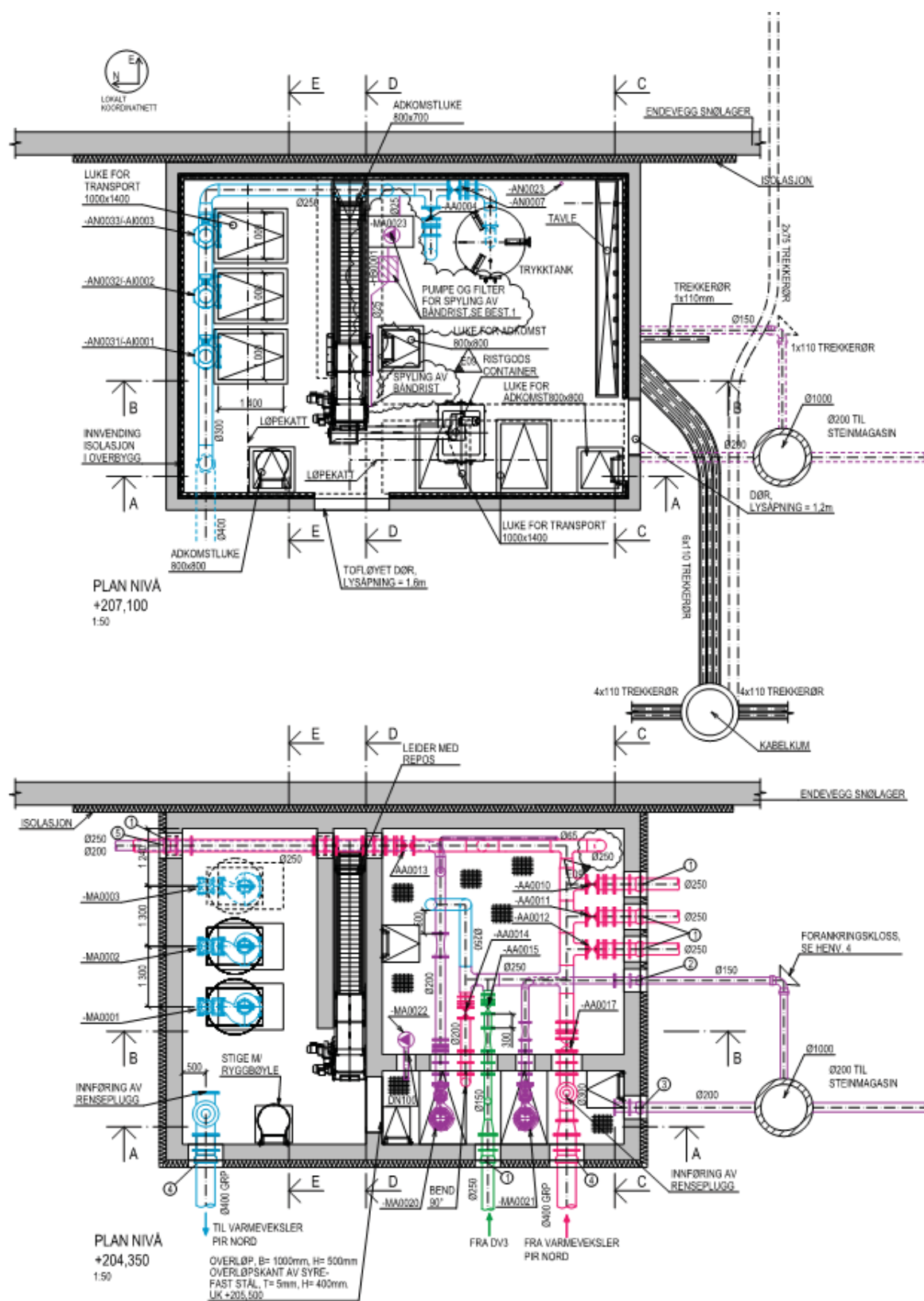
Figur 40 Plantegning pumpestasjon
