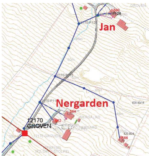
Figur 20: Strømnettet med lavspenning i blått, 22 kV-linje i rødt og transformator som rød firkant. Blå linje på nedsiden fortsetter ned til Grøslund (Loftsgård 2017).
