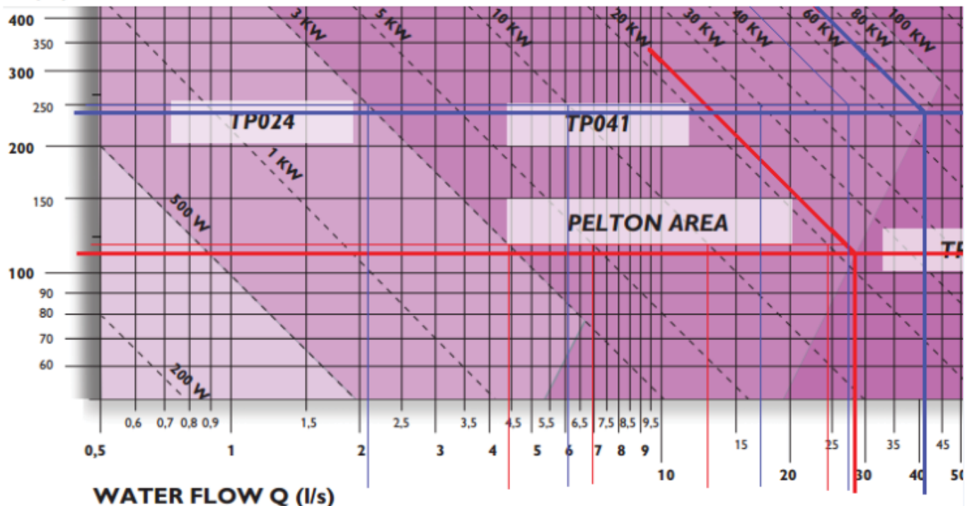
Figur 17: Effektdiagram med flere detaljer enn i figur x (den over). Tykke røde og blå linjer gir netto fallhøyde ved maks slukeevne og tilhørende effekt for de to valgte alternativene (22 kW og 73 kW). Disse vannrette linjene er 10 % lavere enn ved brutto fallhøyde angitt ved sort merke på y-akse. Tynne vannrette linjer markerer krysspunktene mellom valgte vannføringer (loddrette streker) og effekt gitt ved stiplede linjer for å finne de fire andre virkningsgradene.
