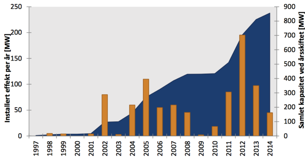
Figur 1: Installert vindkraft i Norge (NVE, 2015)
