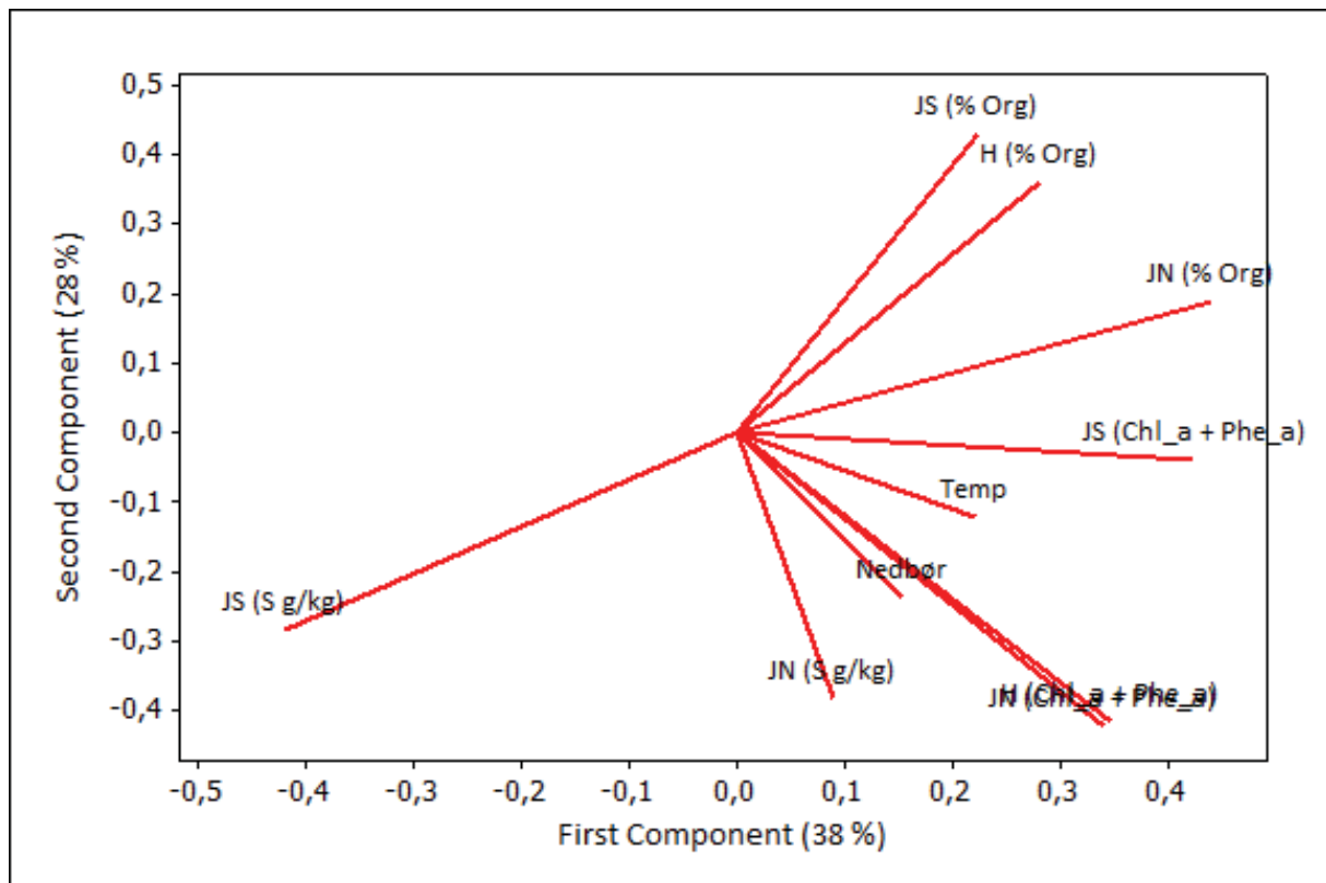
Figur 15. Prinsipal komponent analyse (PCA) for Jarenavatnet nordlig (JN) og sørlig basseng (JS), og Helgetjern (H). Figuren viser en korrelasjon mellom klorofyll a fra Jarenavatnet (nord) og Helgetjern. Temperatur og nedbør viser korrelasjon med klorofyll a for Jarenavatnet (nord og sør) og Helgetjern, men forklarer ikke hele variasjonen. Jarenavatnet (sør) er negativt korrelert med svovelinnholdet i sedimentet. Organisk materiale i Jarenavatnet (sør) og Helgetjern er korrelert. Organisk materiale og klorofyll a er plassert langt fra hverandre og indikerer ulike forklaringsvariabler.
