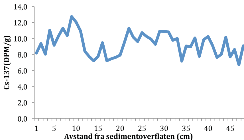
Figur 12. Innholdet av Cs-137 i sedimentsøylen fra sørlig basseng, Jarenvatnet. Resultatene for sørlig basseng viser flere mindre topper, men med en noe høyere topp ved 9 cm i sedimentsøylen.
