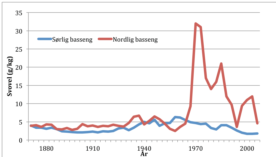
Figur 10. Svovelinholdet i sedimentet til Jarenvatnet for sørlig (blå) og nordlig basseng (rød). I sørlig basseng økes innholdet av svovel fra cirka 1930 fram til 1970 for så å reduseres. I nordlig basseng vises en drastisk økning av svovelinholdet i sedimentet på 1970-tallet, samt to senere toppe rundt 1980 og 2000.
