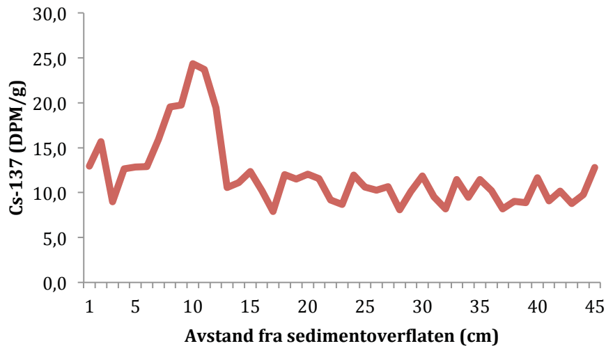
Figur 11. Innholdet av Cs-137 i sedimentsøylen fra nordlig basseng, Jarenvatnet. Figuren viser en tydelig topp ved 10 cm dybde i sedimentsøylen for nordlig basseng.
