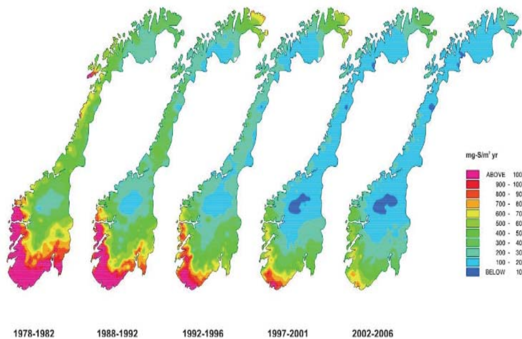
Figur 9. Viser store geografiske ulikheter i mengde avsetning av sjøsaltkorrigert svovel fra 1978 – 2006 ( \text{mg-S/m}^2/\text{år} ) (Aas et al. 2009). Jarenavatnet ligger i et av områdene hvor det har vært størst avsetning av svovel i følge kartet. Samtidig ligger Jarenavatnet i et av områdene som har hatt en rask reduksjon i avsetning av svovel, sett ut av kartet.
