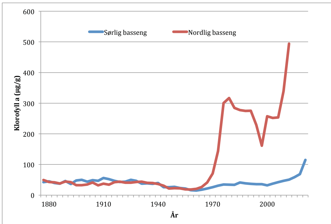
Figur 14. Viser klorofyll a (gitt som klorofyll a + hovednedbrytningsproduktet pheophytin a) for sørlig og nordlig basseng, hvor blå linje er sørlig basseng og rød linje er nordlig basseng. Figuren viser at bassengene ligger på cirka samme nivå fra slutten av 1800-tallet og fram til rundt 1960. Fra rundt 1920 fram til 1960 vises en viss nedgang. Slutten av 1960-tallet / begynnelsen av 1970-tallet viser en markant økning i det nordlige bassenget. En viss økning i det sørlige er også synlig fra rundt 1970-tallet, men forholder seg relativt stabilt hele tidsserien. Etter toppen på 1970- og 1980-tallet stabiliserer det seg noe igjen i det nordlige basseng. En nedgang er synlig i nordlig basseng rundt 2000. Dette er kun en verdi og kan være vanskelig å tolke.
