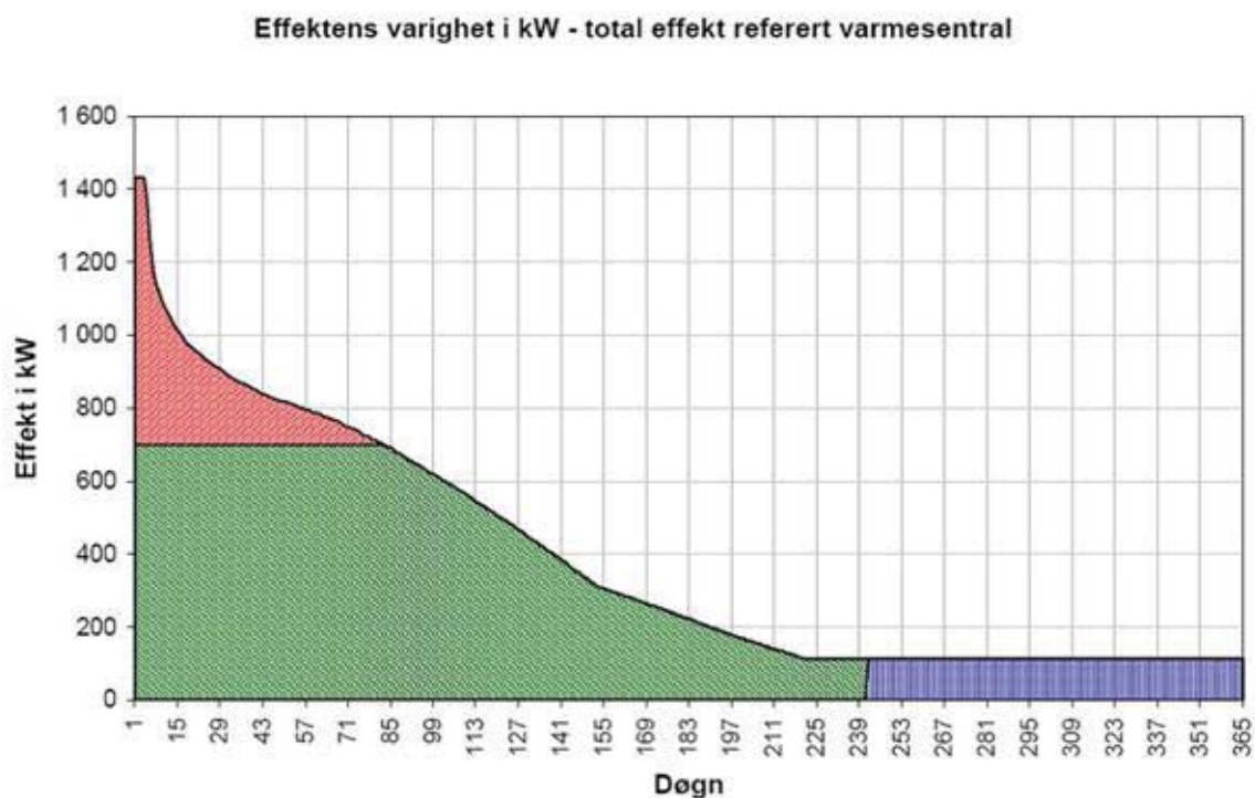
Figur 3: Eksempel på et varighetsdiagram for en varmesentral. (Fossekal 2015)
