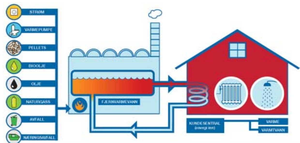
Figur 1: Prinsippskisse for fjernvarme (Kilde: Hafslund)
