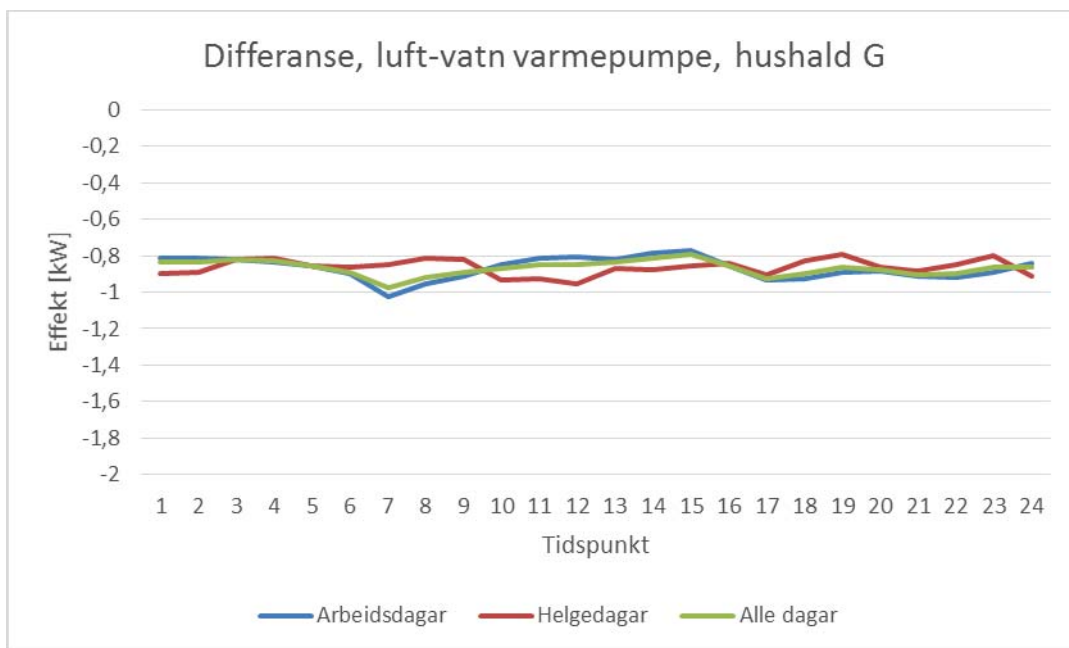
Figur 41 Differansen mellom det totale effektforbruket før og etter installasjon av luft-vatn varmepumpe hos hushald G.
