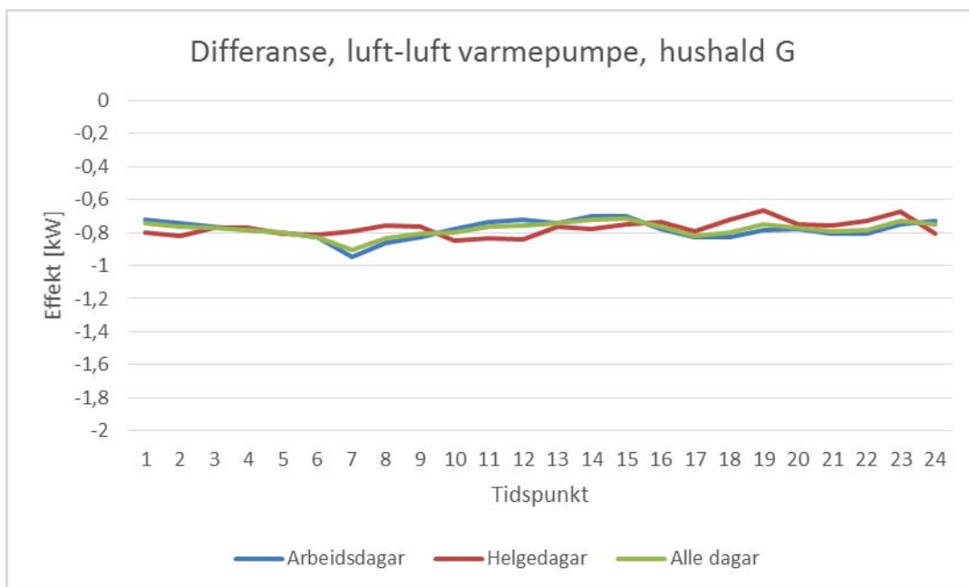
Figur 42 Differansen mellom det totale effektforbruket før og etter installasjon av luft-luft varmepumpe hos hushald G.
