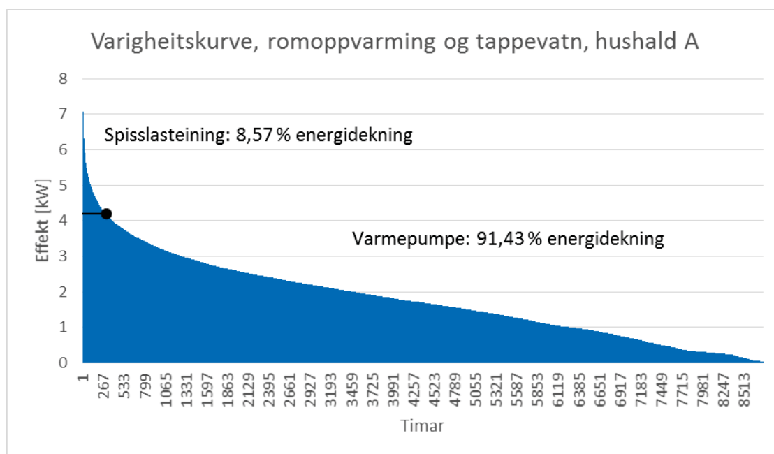
Figur 23 Varighetskurve for romoppvarming og tappevatn hos hushold A med energidekning for spisslasteining og varmepumpe.
