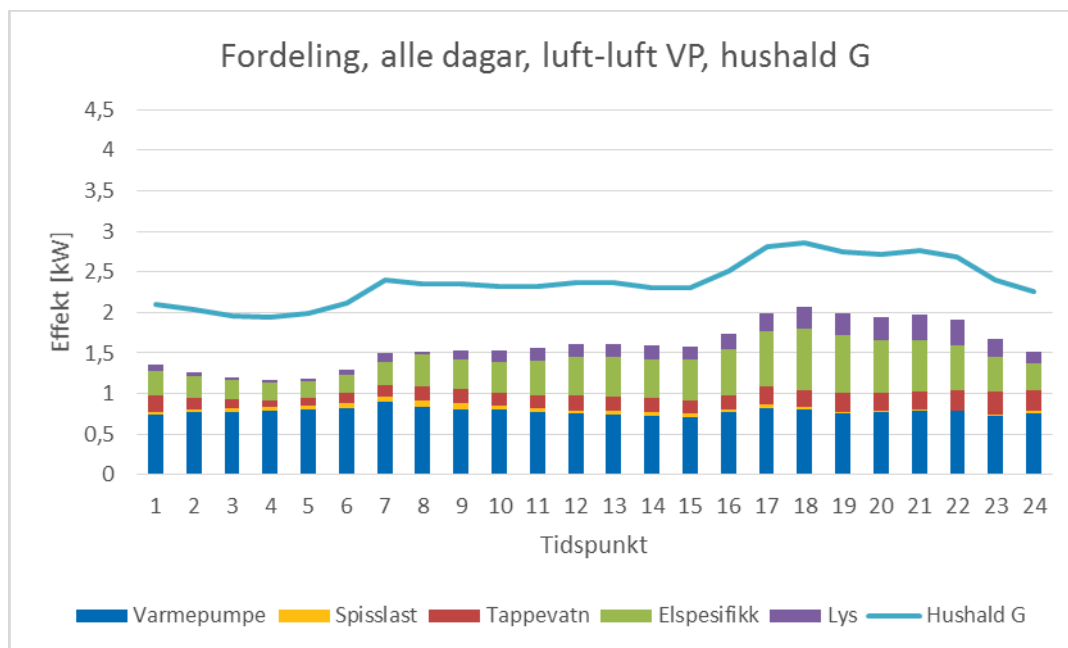
Figur 38 Fordeling, alle dagar, hos hushald G etter installasjon av luft-luft varmepumpe. Den blå linja «hushald G» syner effektforbruket utan varmepumpe.
