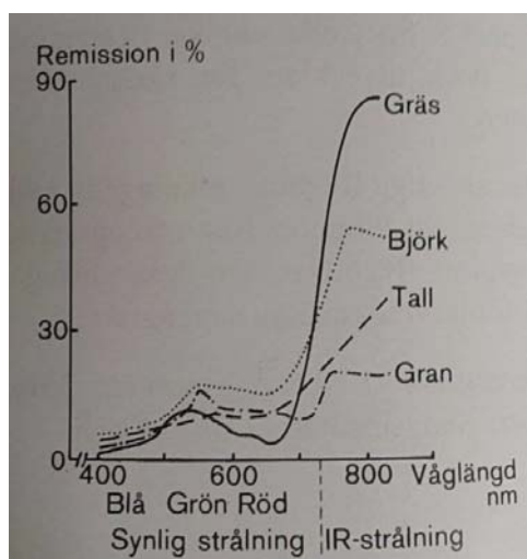
Figur 6: Spektral refleksjonsevnen, det vil si refleksjonen i forskjellige bølgelengdeområder, for noen forskjellige treslag og gress. Treslagsrefleksjonen er størst i IR-området (Axelson & Nämnden för skoglig, 1980).
