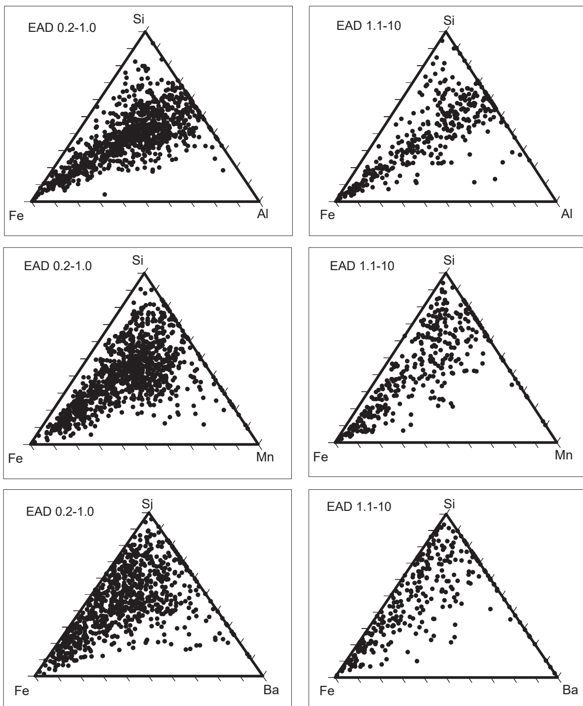
Figur 8-15: Tertiærplot fra partikler ( n = 986 ) deponert på mosenett fra industri #5 (figur 7-2) fordelt på størrelsene EAD 0.2-1.0 og n = 370 EAD 1.1-10. Resultatene er fra EDS-analyse utført i VP-SEM.
