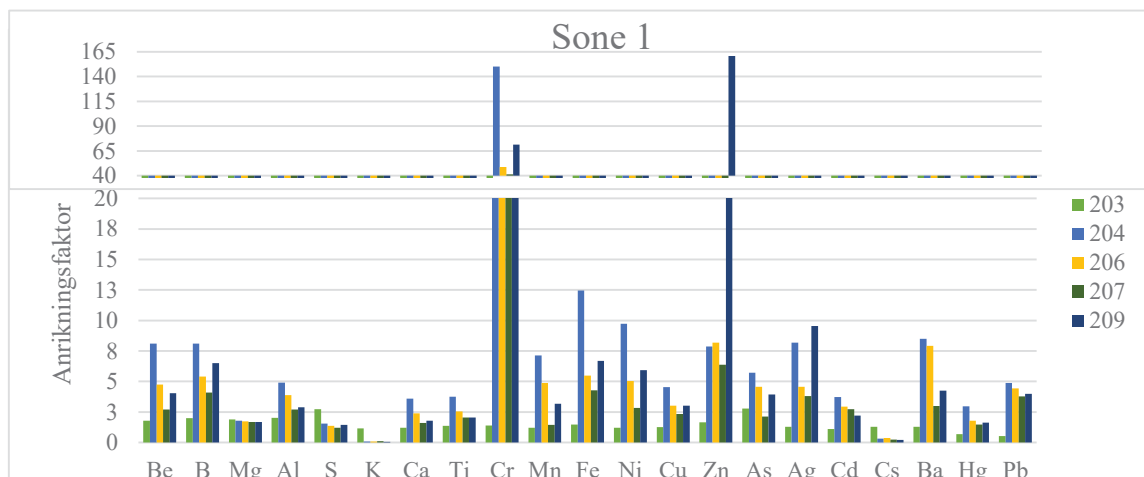
Figur 8-3: Anrikningsfaktor (beregnet ved likning 2) for grunnstoffer i H.splendens bestemt ved ICP-MS. Mosenett med de to siste årsskudd ble plassert som vist i figur 7-2 i sone 1 (figur 7-3) Y-aksen har en splitt mellom 20-40, n=5 .
