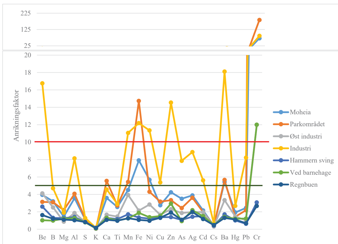
Figur 8-2: Anrikningsfaktor (beregnet ved likning 2) for grunnstoffer i H.splendens bestemt ved ICP-MS. Mosenett med de to siste årsskudd ble plassert som vist i figur 7-2. Tydelig anrikning på mose er definert mellom rød og grønn linje og åpenbar forurensning er definert over rød linje (inndeling i tabell 8-1)
