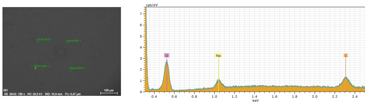
Figur F-2: EDS- spekter og bilde fra midten av stub posisjon 1 analysert på tab, karbonsignalet vises ikke i spekteret.
