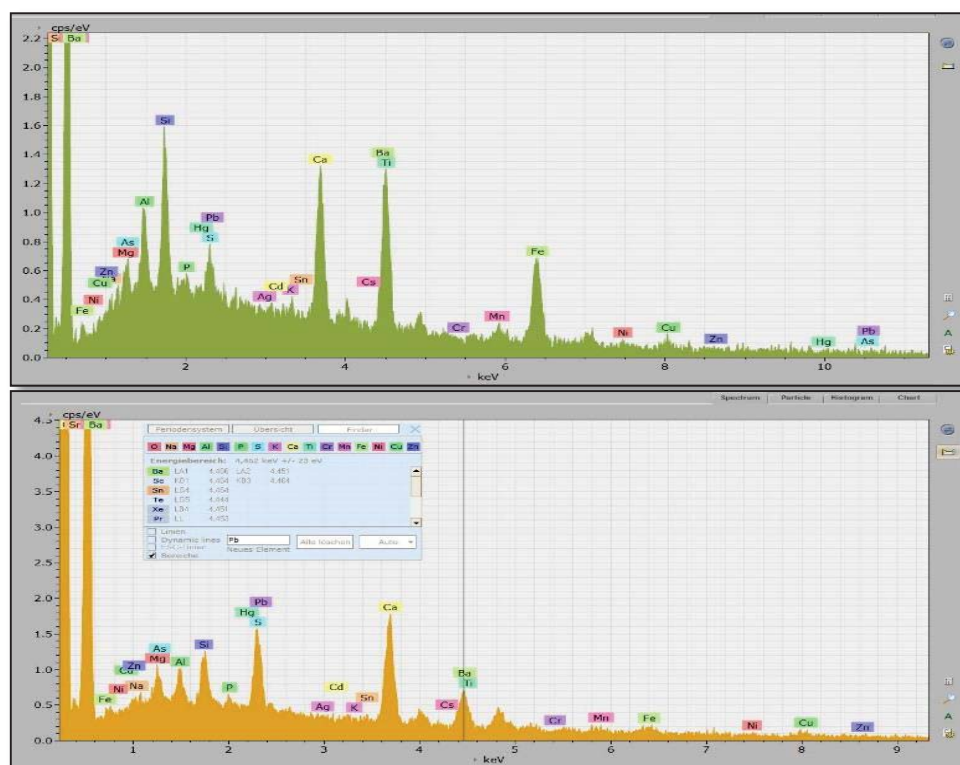
Figur 8-10: Eksempel på spekter fra titan (øverst) og barium (nederst) fra EDS på partikler avsatt på moseblad
