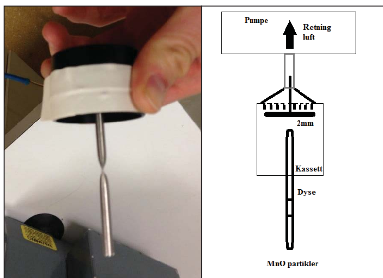
Figur 7-7: Kassett ferdig montert (til venstre, foto: privat) og en skjematisk fremstilling av oppsettet med dysen pekene mot partikler på aluminiumsplate (høyre figur)
