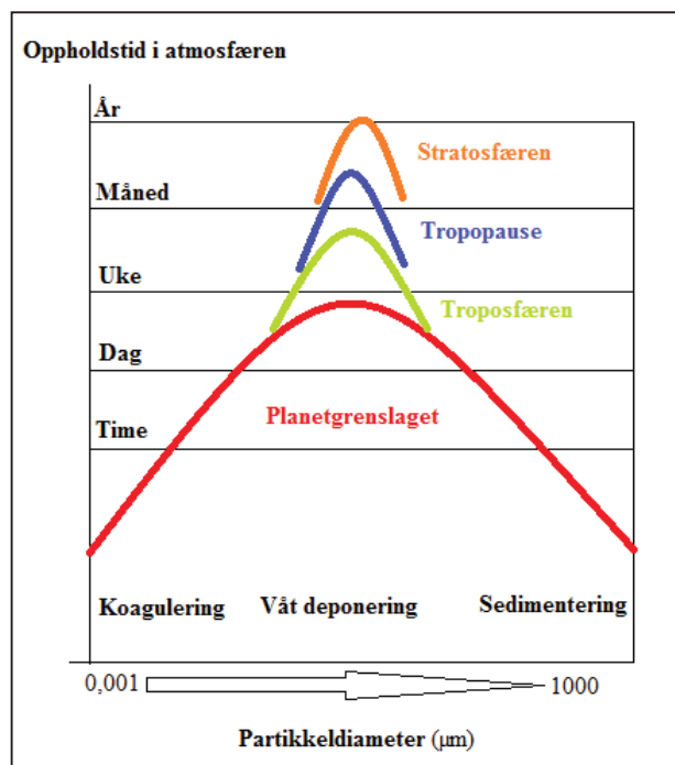
Figur 2-2: Oppholdstid og i hvilken høyde partiklene befinner seg i atmosfæren, samt forventet deponeringssitasjon (etter Jaenicke, 1980)
