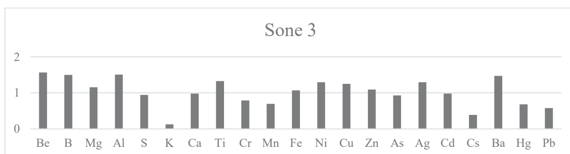
Figur 8-5: Anrikningsfaktor (beregnet ved likning 2) for grunnstoffer i H.splendens bestemt ved ICP-MS. Mosenett med de to siste årsskudd ble plassert som vist i figur 7-2 i sone 3 (figur 7-3), n=1 .
