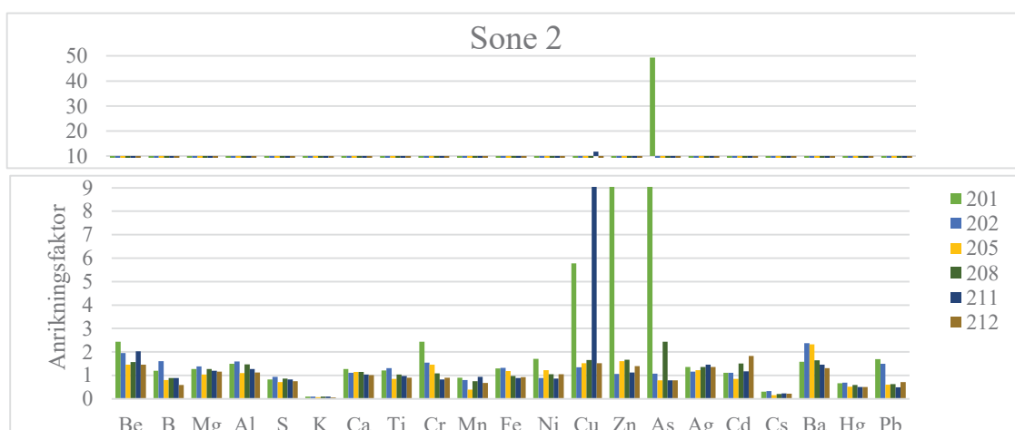
Figur 8-4: Anrikningsfaktor (beregnet ved likning 2) for grunnstoffer i H.splendens bestemt ved ICP-MS. Mosenett med de to siste årsskudd ble plassert som vist i figur 7-2 i sone 2 (figur 7-3) Y-aksen er delt mellom 9-10, n=6
