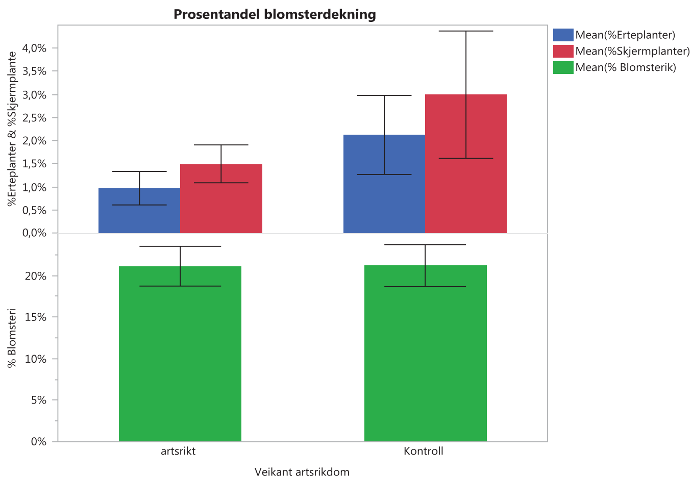
Figur 7: Prosentandel gjennomsnittlig blomsterdekning med standarfeil i de definerte artsrike veikanter og kontrollveikanter.
