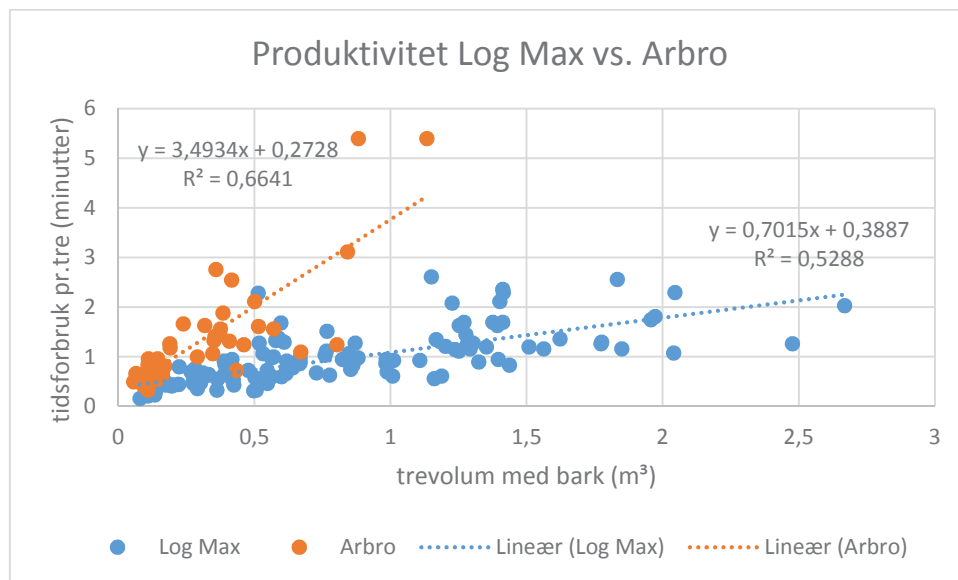
Figur 14. Produktivitet Log Max vs. Arbro, tidsforbruk (minutter / tre) i forhold til trevolum (m³).
