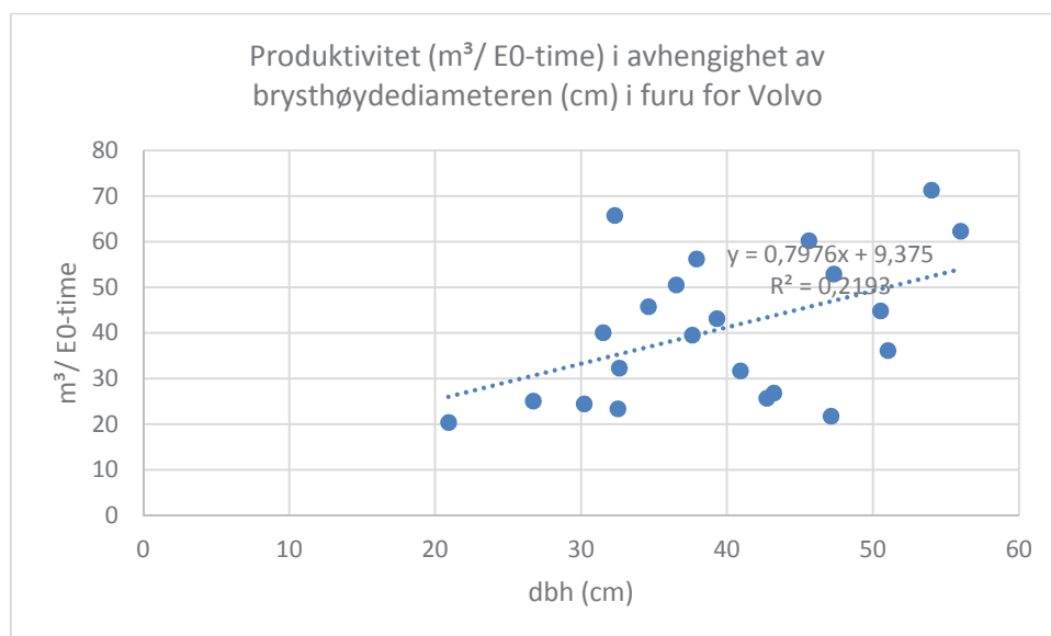
Figur 10. Produktivitet ( \text{m}^3/\text{E0-time} ) i avhengighet av brysthøydiameteren (cm) i furu for Volvo.
