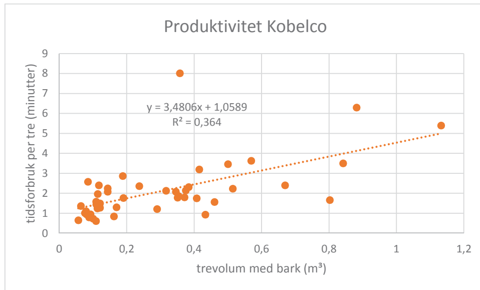
Figur 4. Produktivitet for Kobelco, tidsforbruk (minutter /tre) i forhold til trevolum (m³).
