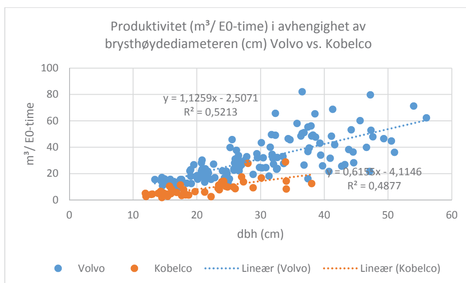
Figur 7. Produktivitet (m³/ E0-time) i avhengighet av brysthøydiameteren (cm) Volvo vs. Kobelco.
