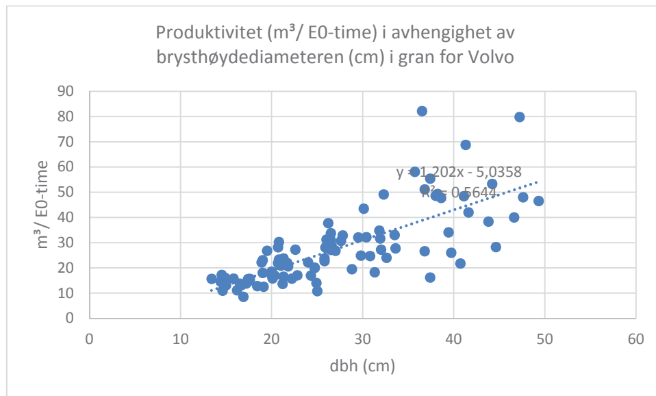
Figur 9. Produktivitet ( \text{m}^3/\text{E0-time} ) i avhengighet av brysthøydiameteren (cm) i gran for Volvo.
