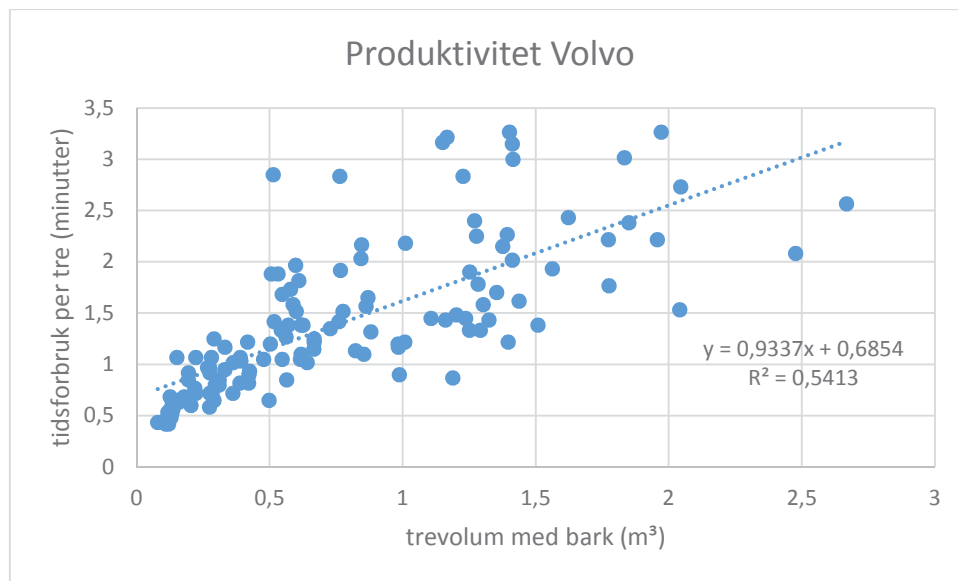
Figur 3. Produktivitet for Volvo, tidsforbruk (minutter / tre) i forhold til trevolum (m³).
