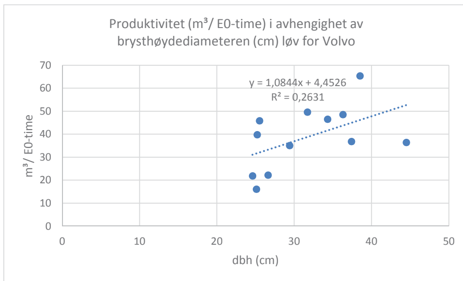
Figur 11. Produktivitet (m³/ E0-time) i avhengighet av brysthøydiameteren (cm) i løv for Volvo. Analysen av produktiviteten i avhengighet av brysthøydiameteren for gran viser et nokså likt bilde som for alle treslag samlet. Produktiviteten øker med økende brysthøydiameter. Spredningen i produktivitet er stor for trær med stor brysthøydiameter. Produktiviteten i avhengighet av brysthøye for furu og løv gir et mer tilfeldig bilde med stor spredning på trær med ulike brysthøydiameter.
