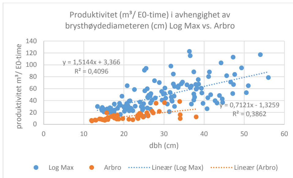
Figur 15. Produktivitet ( \text{m}^3/\text{E0-time} ) i avhengighet av brysthøydiameteren (cm) Log Max vs. Arbro. Regresjonslinjene viser at produktiviteten øker med økende brysthøydiameter for begge maskinene. Jo større brysthøydiameteren er, desto større er produktiviteten. Stigningstallet på regresjonslinjen til Log Max aggregatet er på 1,51. Stigningstallet på regresjonslinjen til Arbro aggregatet er på 0,71. Stigningstallet er altså dobbelt så stort for Log Max. Dette betyr at økningen i produktivitet når brysthøydiameter øker er mye større for Log Max aggregatet enn for Arbro aggregatet.
