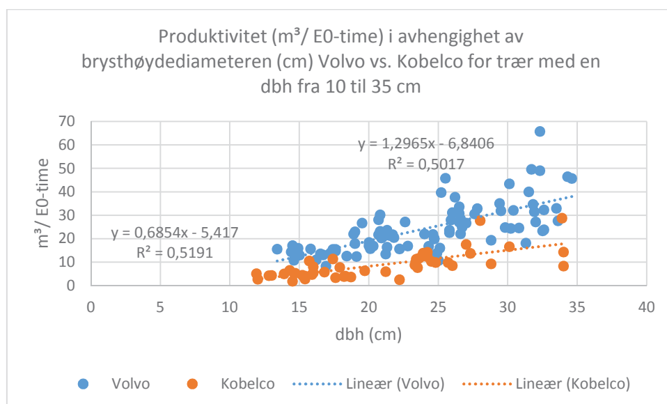
Figur 8. Produktivitet (m³/ E0-time) i avhengighet av brysthøydiameteren (cm) Volvo vs. Kobelco for trær med en dbh fra 10 til 35 cm.
