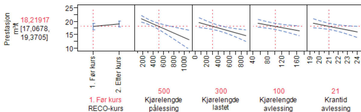
Figur 33: Lassbærer 1. Forklaringsvariabler til variasjon i prestasjon
