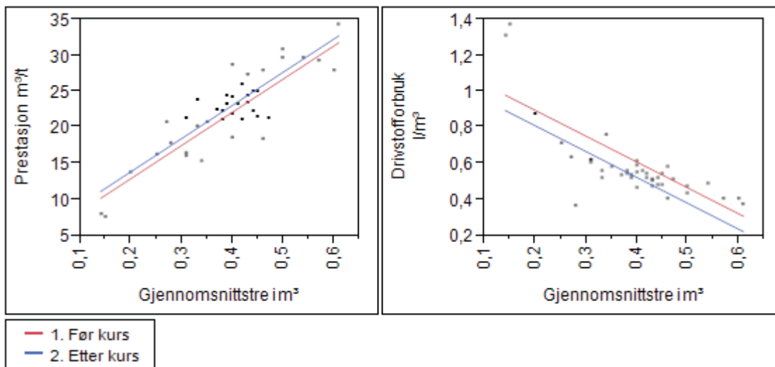
Figur 20: Hogstmaskin 1. Prestasjon og drivstofforbruksmodell ved varierende gjennomsnittlig trestørrelse i kubikkmeter
