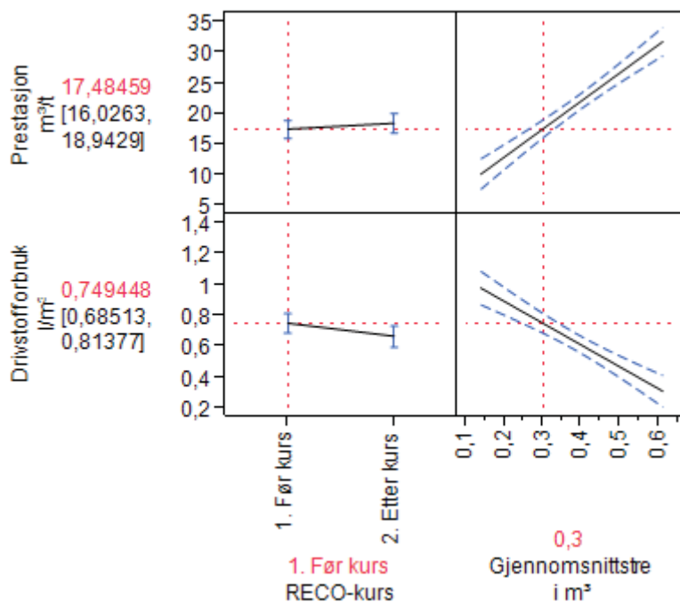
Figur 21: Hogstmaskin 1. Forklaringsvariabler til variasjon i prestasjon og drivstofforbruk
