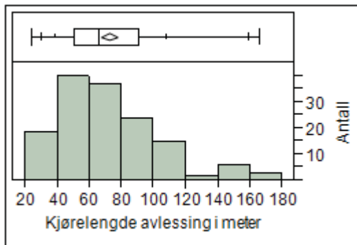
Figur 15: Fordeling av kjørelengde avlessing for lassbærer, meter
