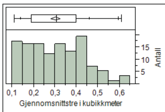
Figur 6: Fordeling av gjennomsnittlig trestørrelse for hogstmaskiner, kubikkmeter pr tre
