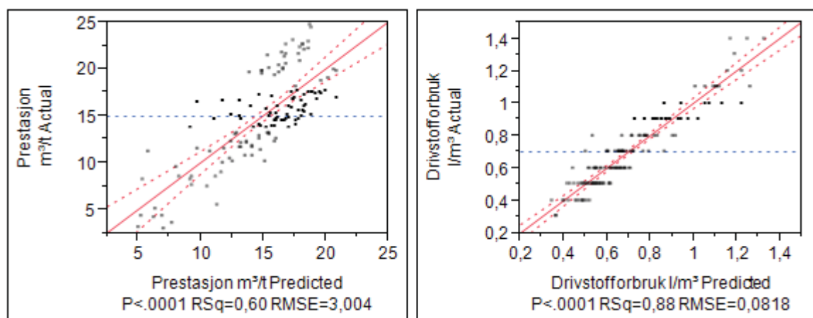
Figur 44: Samtlige lassbærere. Prestasjon og drivstofforbruksmodell
