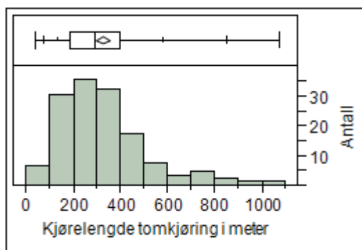
Figur 12: Fordeling av kjørelengde tomkjøring for lassbærer, meter
