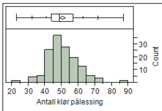
Figur 16: Fordeling av antall klør pålessing for lassbærer
