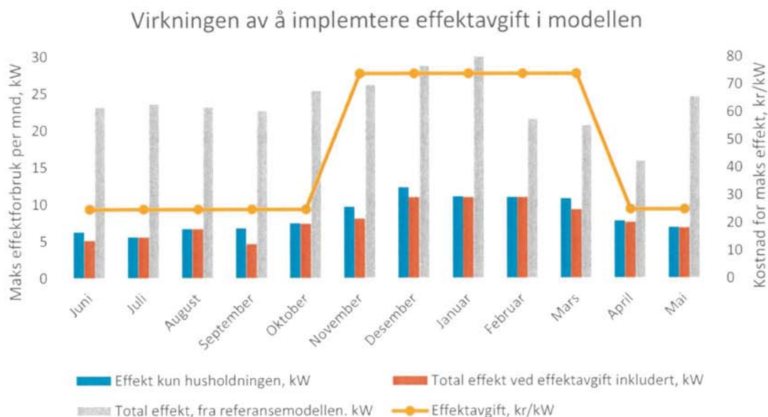
Figur 14. Virkningen av å implementere effektaggift i modellen, nivå 2
