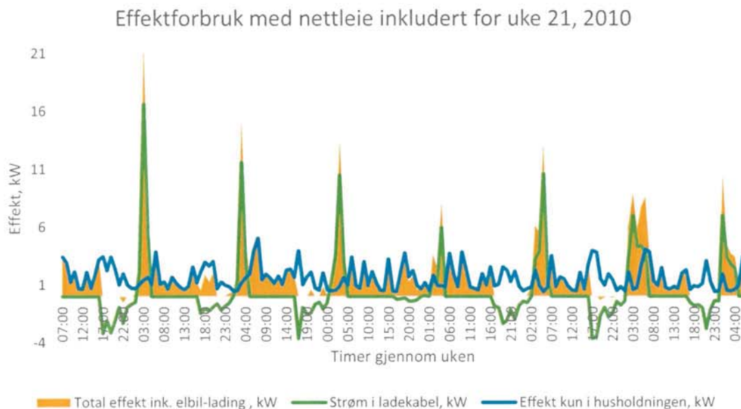
Figur 11. Effektforbruket med nettleie inkludert for uke 21, 2010
