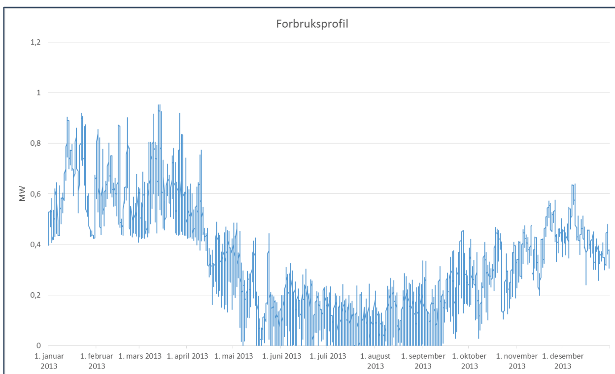
Figur 4 Beregnet forbruksprofil f.o.m 1. januar t.o.m. 31. desember 2013.
