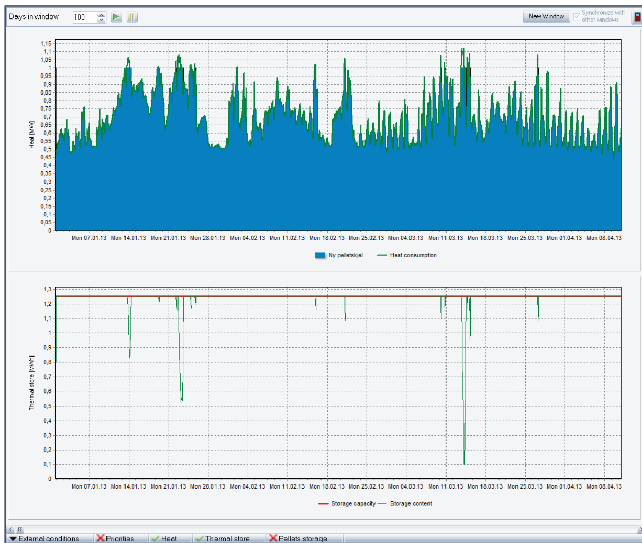
Figur 13 Utsnitt av beregnet varmeproduksjon og endringer i lagerkapasitet for et tenkt år med høyere energibehov og varmeproduksjon fra pellets til etterspørsel og lager, samt olje som reservelast, vinter.
