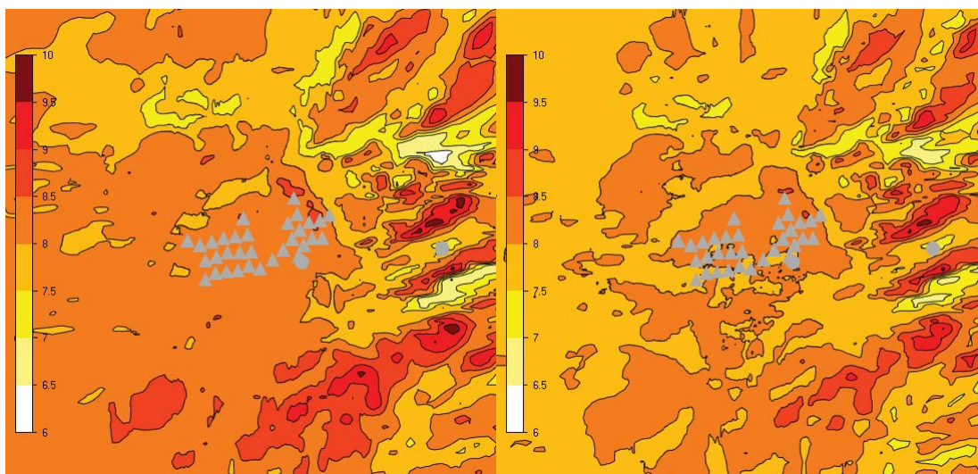
Figur 20: Vindressurskart ved 80 meters høyde for referansemodellen (til venstre) og skogsmodell 1 (til høyre).
