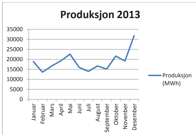
Figur 26: Energiproduksjon per måned 2013.
