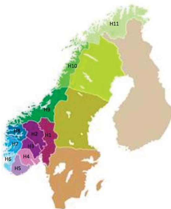
Figur 3.3 – Hydrologiregioner etter HBV-modellen
