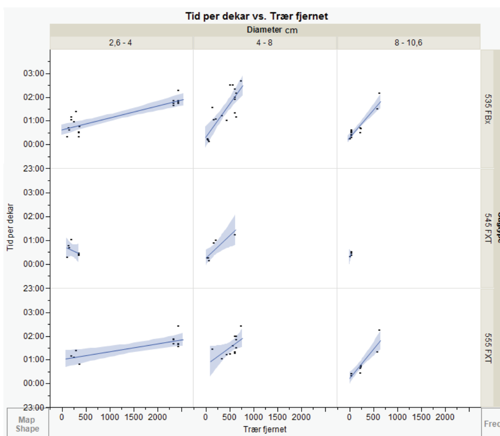
Figur 10. Prestasjonstider per dekar for hver sag, gruppert i diameterklasser og vist mot uttaksstyrke. Merk at det lave antallet observasjoner for sagtype 545 FXT ved visse variabler gir dårlige trendlinjer. Blå linje = tid per dekar.
