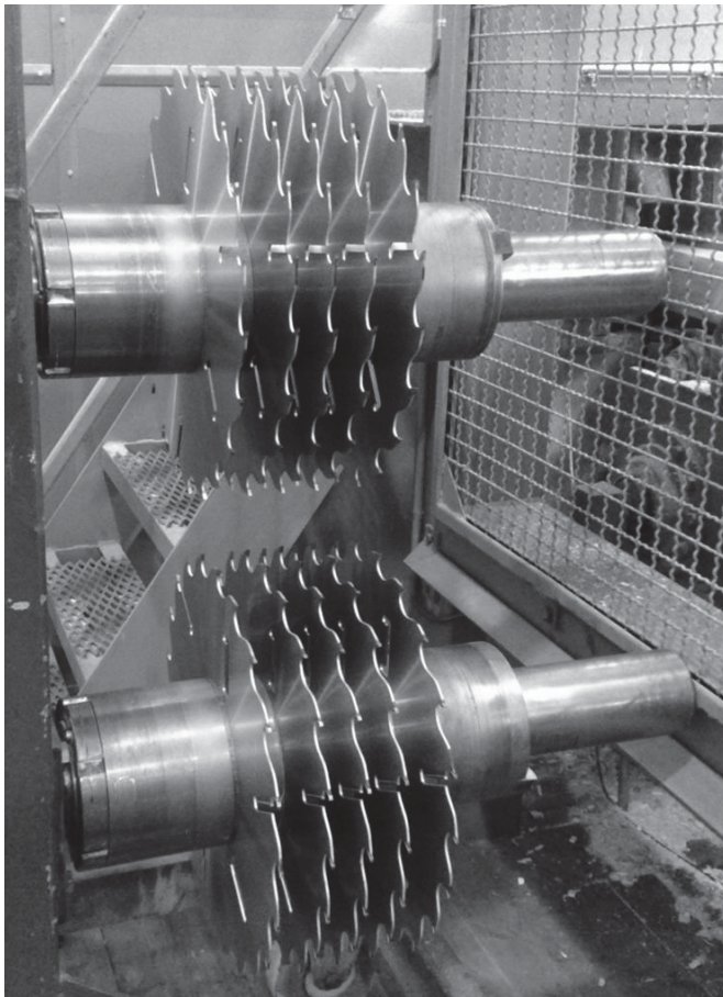
Figur 2 Bilde av over- og underliggende sagblad. Avstanden mellom bladene er det som utgjør postningen. (Foto: Brede Rogstadkjærnet)
