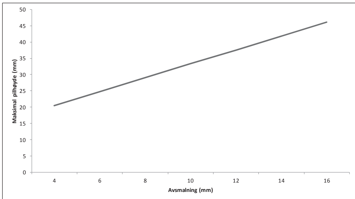
Figur 22 Visualisering av Modell I. Avsmalning (mm/m) langs x-aksen og pilhøyde (mm) langs y-aksen. Verdiene som fremkommer er de maksimale verdiene forklaringsvariablene kan ha, uten at det forventes vankant.
