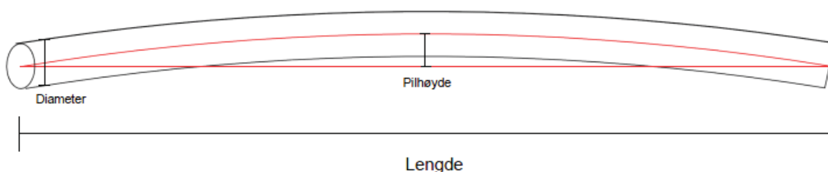
Figur 8 De grå strekene viser omrisset av en tømmerstokk sett fra siden. Den øvre røde linjen er senterlinja som følger kroken, den nedre er ei referanselinja som går mellom senter av endeflatene.
