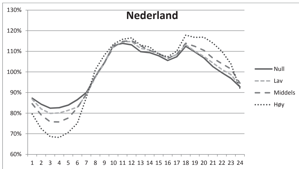
Figur 5.5: Prisvariasjon for time på døgnet for Nederland i 2030 (100 % er døgngjennomsnittspris).
