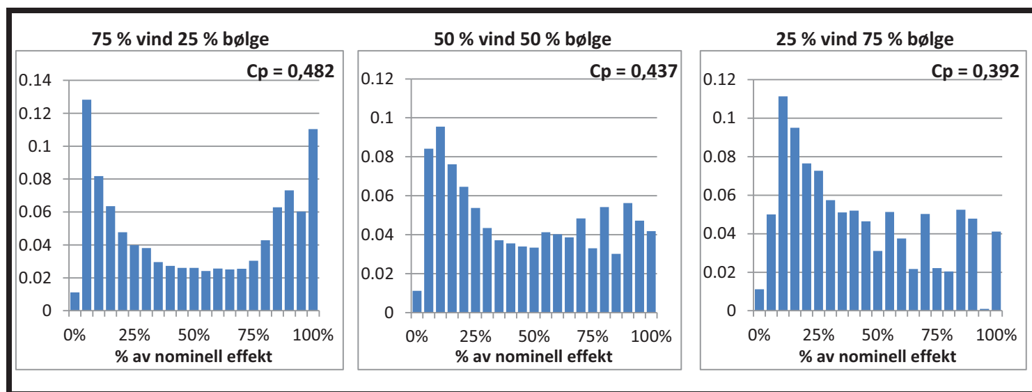
Figur 3.19 Produksjonskurver for forskjellige kombinasjoner av vind- og bølgekraft for Utsira Nord
