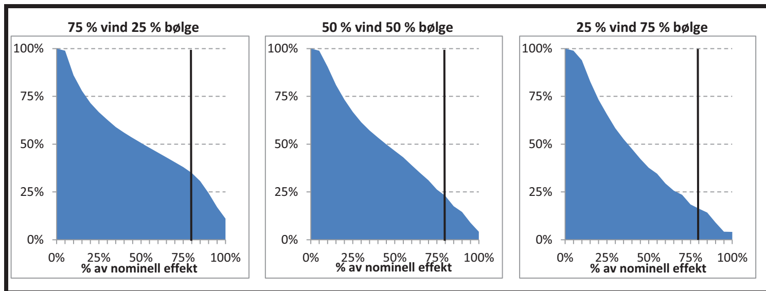
Figur 3.32 Optimeringskurve for forskjellige kombinasjoner av vind- og bølgekraft for Utsira Nord
