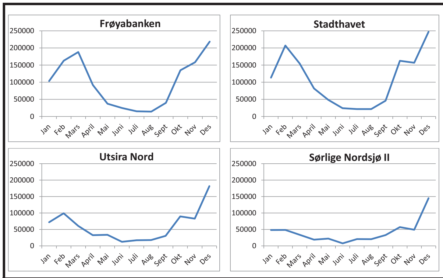
Figur 3.1 Teoretisk bølgekraft produksjon ved de fire områdene i 2011 (y aksen = kWh/m bølgefront)
