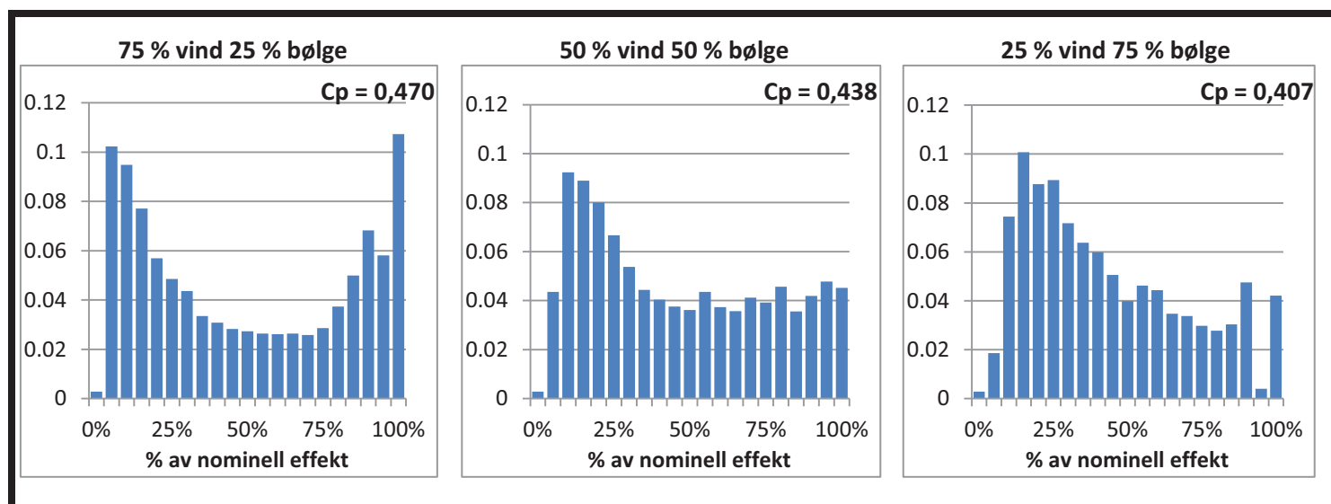
Figur 3.15 Produksjonskurver for forskjellige kombinasjoner av vind- og bølgekraft for Frøyabanken
