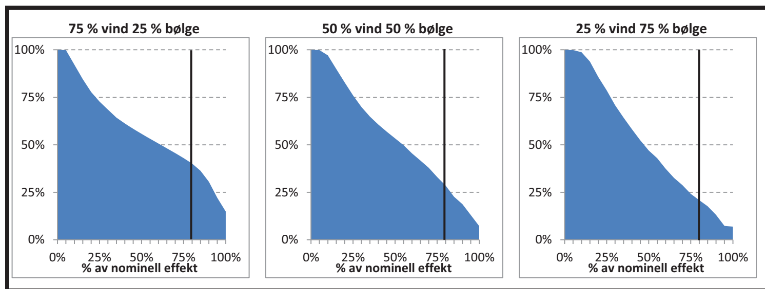
Figur 3.30 Optimeringskurve for forskjellige kombinasjoner av vind- og bølgekraft for Stadthavet
