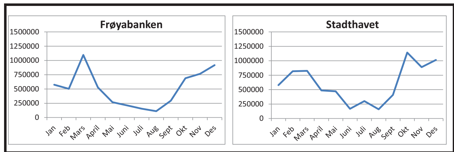
Figur 3.2 Teoretisk vindkraft produksjon ved Frøyabanken og Stadthavet i 2011 (y aksen = kWh/m 2 )
