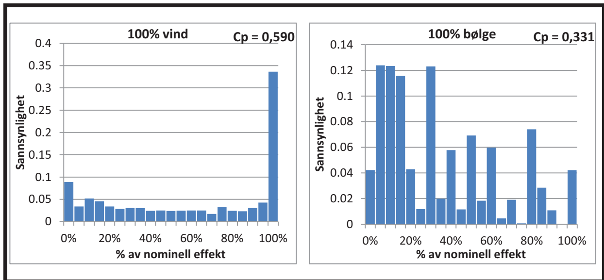
Figur 3.20 Produksjonskurver ved 100 % vindpark og 100 % bølgepark for Sørliche Nordsjø II
