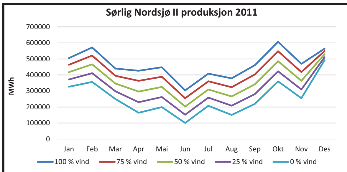
Figur 3.25 Produksjon ved forskjellige kominasjoner av vind og bølge for Sørlige Nordsjø II i 2011
