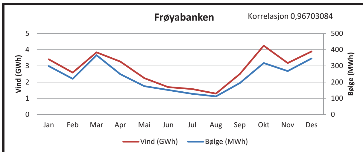
Figur 3.9 Produksjonen til en Vestas V164-7MW vindturbin og et Pelamis P2 bølgekraftverk i 2011
