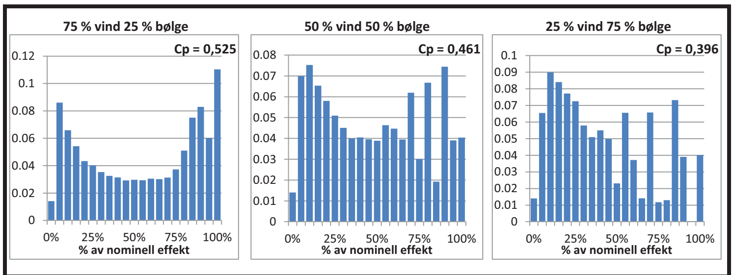
Figur 3.21 Produksjonskurver for forskjellige kombinasjoner av vind- og bølgekraft for Sørliche Nordsjø II
