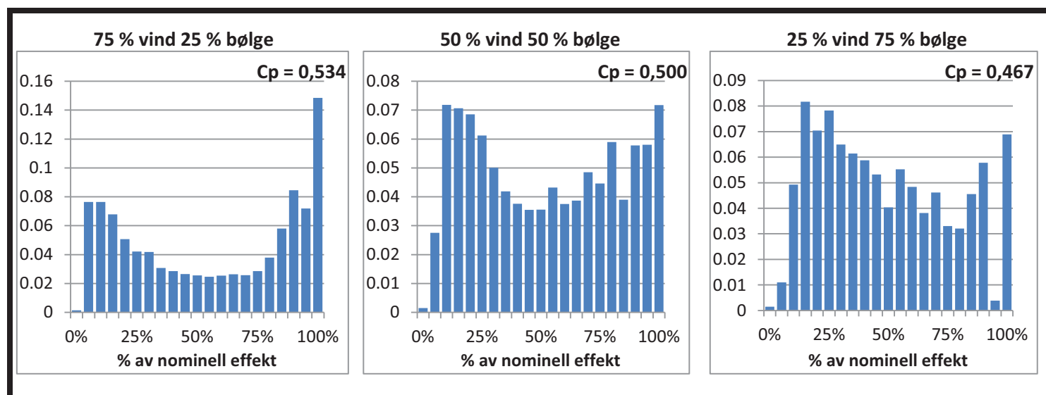
Figur 3.17 Produksjonskurver for forskjellige kombinasjoner av vind- og bølgekraft for Stadthavet
