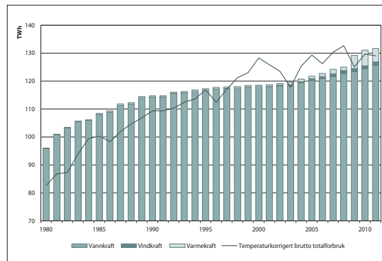
Figur 4: Normal produksjonsevne og temperaturkorrigert forbruk i Norge. Kilde (Regjeringen 2012b)
