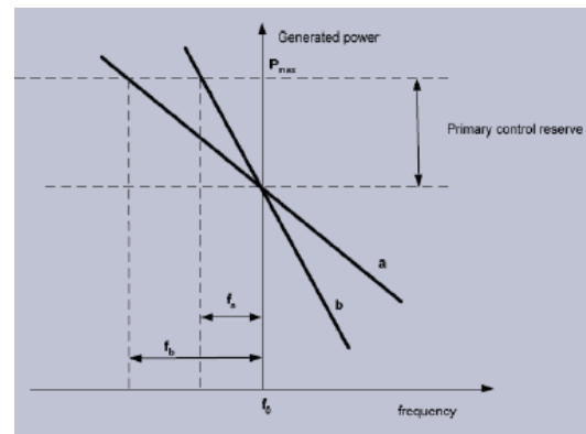
Figur 15 - Forskjellig generator "droop". Kilde (Gjengedal 2012b)
