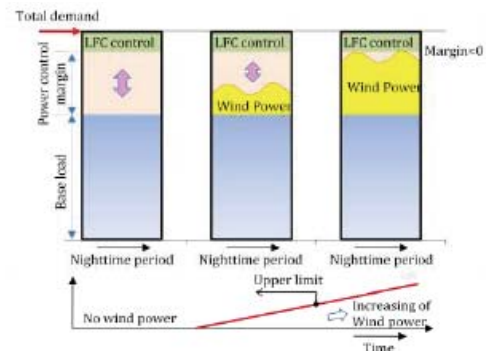
Figur 19 - Vindkraft og påvirkning på kontrollreservene på natten. Kilde (IEA 2009)
