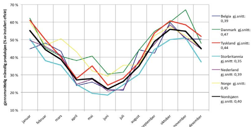
Figur 4-4: Gjennomsnittelig månedlig produksjonsnivå vist i prosent av installert effekt. Alle land i medium scenario
