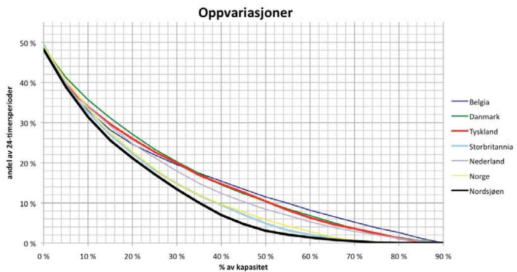
Figur 5-4: Kurven viser hvor mange prosent av 24-timersvariasjonene som er større enn gitte størrelser av variasjoner. Alle land i medium scenario
