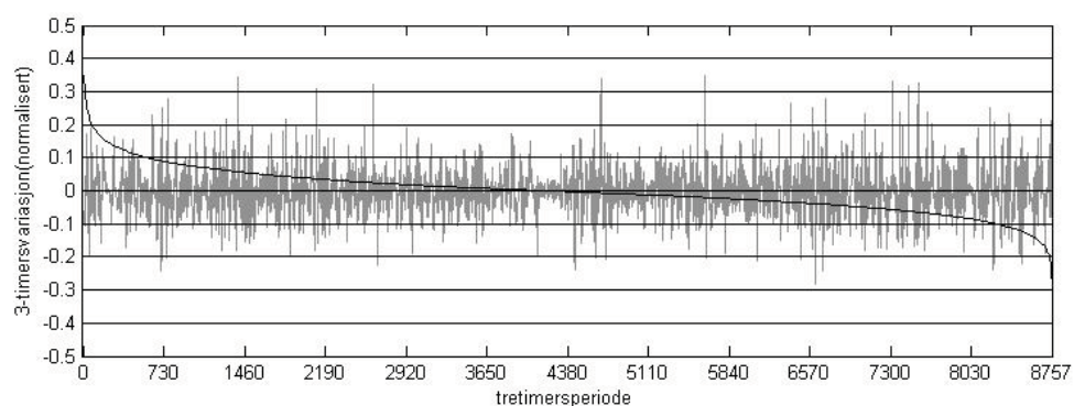
I tidsserie(varighetskurve). Medium scenario
