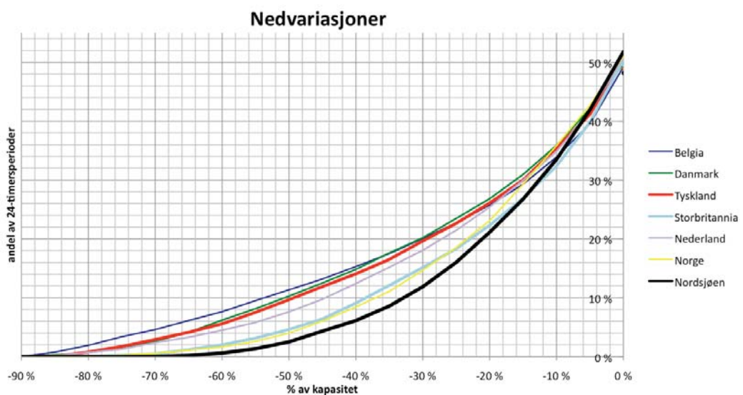
Figur 5-5: Kurven viser hvor mange prosent av 24-timersvariasjonene som er mindre enn gitte størrelser av variasjoner. Alle land i medium scenario
