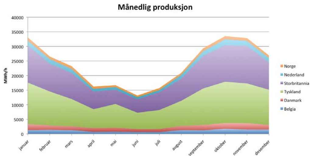
Figur 4-3: Gjennomsnittelig månedlig produksjonsnivå i Nordsjøen ved medium scenario
