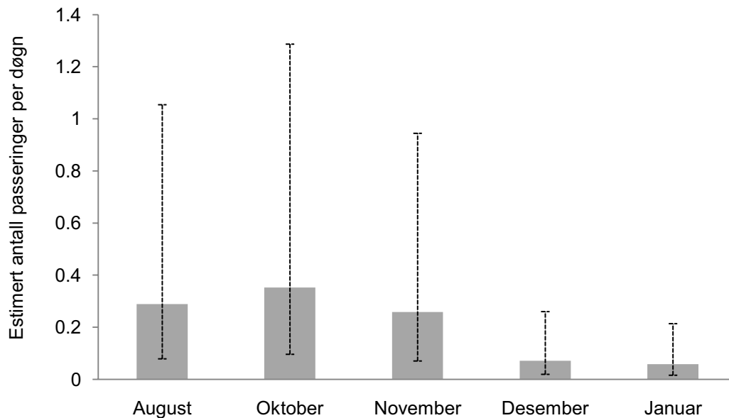
Figur 13. Forventet antall passeringer per døgn per måned, for de ulike passasjene inkludert i analysen samlet, oppgitt som medianen av de tilbaketransformerte dataene. Stiplede linjer viser 95 % konfidensintervall. Øvre og nedre grense for konfidensintervallet er også estimert ved tilbaketransformering av testverdier, basert på log10 – transformerte grunndata, for å illustrere resultatet. Det er i testen kontrollert for tilfeldig effekt av passasje, noe som også påvirker gjennomsnittets størrelse ( N = 25 observasjoner, tilfeldig effekt = 5 passasjer).
