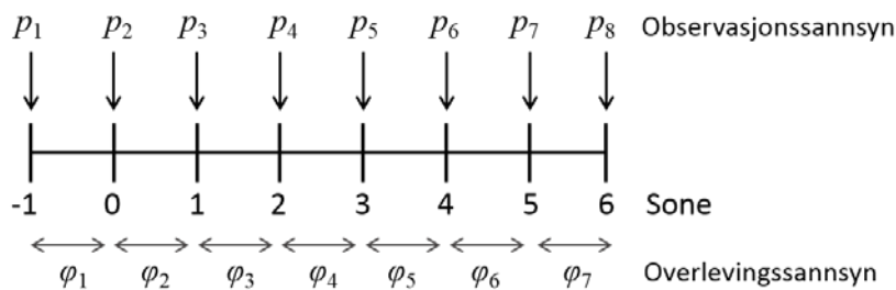
Figur 9. A. Lagnadsdiagram for laksesmolt med fem døme på observasjonshistorier med gjevne parameterar for såkalla Cormack-Jolly-Seber modellstruktur (CJS). \phi_i tyder overlevingssannsyn mellom sone i og i+1 og p_i er observasjonssannsyn i sone i . B. CJS-parameterisering av modellen [ \phi(\text{sone}) , p(\text{sone}) ]. Her vil kvar sone ha eigne estimat for begge parametertypene. For siste sona kan ikkje p og \phi estimerast kvar for seg (berre produktet av dei to).
