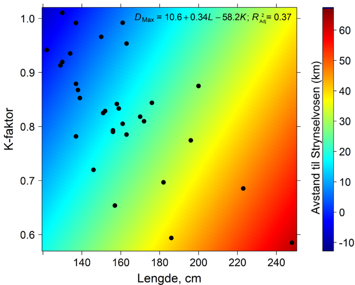
Figur 23. Estimert maksimumsavstand ( D_{Max} ) for AT-merka auresmolt frå Stryneelva i 2017 som funksjon av lengde ( L ) og kondisjonsfaktor ( K ) ved merking. Estimata er framsett som fargekonturar som kjem frå modellen som er gjeve i høgre hjørne av figuren. Dei svarte punkta er observerte lengde og kondisjonsfaktorar. Negative tal for avstand tyder at fisken er i elva, oppstrøms utosen.
