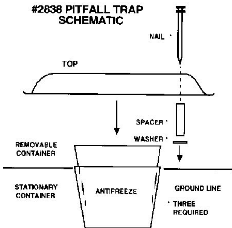
Figur 3. Skjematisk skisse av fallfelle (figur fra BioQuip; produsenten som vi har kjøpt fellene av). Hver felle består av to like begre som er plassert oppi hverandre. Fellene ble gravd ned i flukt med bakken. Det ytterste begeret stod permanent nedgravd i jorden gjennom hele feltsesongen. Det innerste begeret ble fylt halvveis opp (2.5 dl) med en 1:1 blanding av propylenglykol (ikke-giftig konserveringsvæske) og vann (et blandingsforhold som gir stabilt væskevolum i en hel måned), pluss noen dråper Zalo som overflatevirkemiddel. Etter at fellene var plassert nede i jorden, ble det montert tak over for å hindre oversvømmelse (regnvann) og at større dyr (mus, frosk etc) druknet i fellene.
