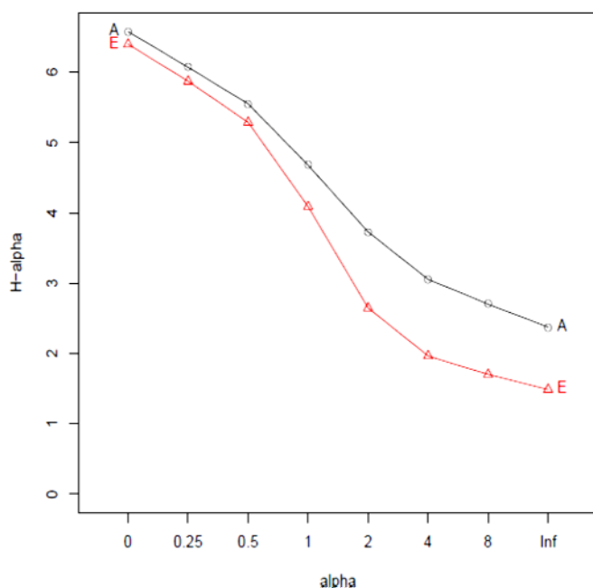
Figur 22. Artsrikdom og biodiversitet av biller fanget midt i kraftgater (A) og 100 m inne i skog (E) , basert på aggregerte data fra 20 målestasjoner (materiale fra både vindusfeller, fallfeller og slagghåving). Figuren viser Rényi diversitetsprofiler for hvert habitat. Utgangsposisjonen på venstre side av profilene indikerer artsrikdom; profiler som starter høyere oppe har høyere artsrikdom. Hvis man tar antilogaritmen ( e^{H\text{-verdi}} ) for \alpha = 0 , får man artsrikdom (A: 721 arter, E: 602). Se også Figur 6 for forklaring av diagrammet. Profiler som ligger høyere enn andre profiler for alle verdier av \alpha , har høyere biodiversitet. Jo brattere kurve, jo større er forskjell i andel av ulike billearter. Billene ble fanget på de samme 4 m x 5 m prøveflatene som beskrevet i teksten til Figur 2, med tre ulike innsamlingsmetoder på hver prøveflate: fallfeller, vindusfeller og slagghåv.
