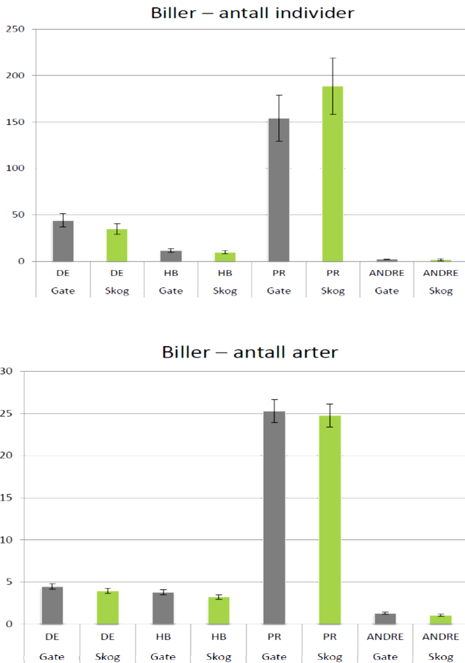
Figur 27. Antall individer (øverst) og arter (nederst) av biller fanget med fallfeller i kraftgater og skog, fordelt på ulike funksjonelle grupper. Figurene viser estimerte gjennomsnittsverdier og tilhørende standardfeil (mål på usikkerhet) for hhv antall individer og antall arter fanget i to fallfeller utplassert i hhv subplot 1 og subplot 5 i 4m x 5m plott (prøveflater) vist i Figur 2, på 20 stasjoner markert med oransje punkter i Figur 1. Alle billeartene i materialet ble kategorisert etter deres viktigste økologiske funksjon, og plassert i en av følgende kategorier: HB – herbivor (plantespiser), FU – fungivor (soppspiser), PR – predator, DW – dead wood (død ved), LW – live wood (levede ved), DE – detritivor (spiser diverse (dødt) organisk materiale). Kategoriene FU, DW og LW hadde svært få arter og individer, og ble slått sammen i kategorien 'ANDRE' før statistiske analyser av materialet.
