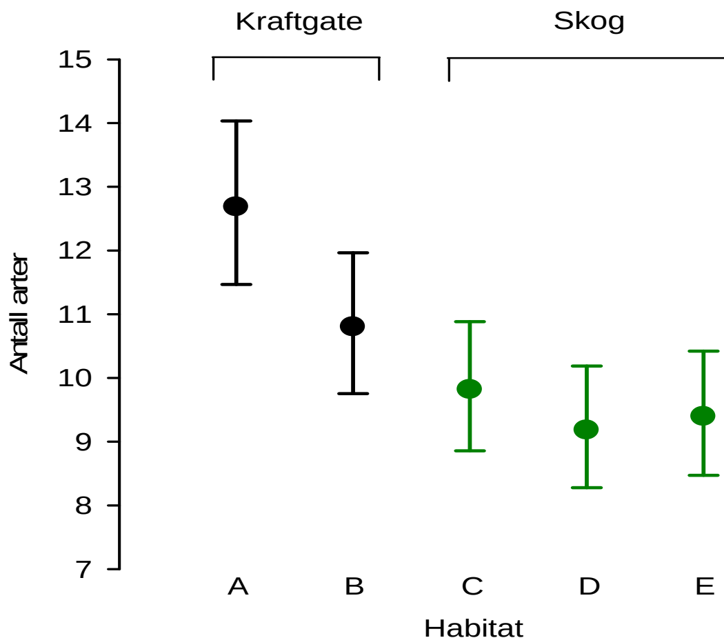
Figur 8. Artsrikdom av karplanter var høyere midt i kraftgatene (habitat A) enn i skog (C: skogkant, D: halv gatebredde inn i skogen og E: 100 m inn i skogen). Figuren viser estimerte gjennomsnittverdier og 95% konfidensintervaller for fem ulike habitater (A, B: i kanten av kraftgaten, C, D og E), kontrollert for variasjon mellom målestasjoner. På hver av de 51 målestasjonene ligger prøveflatene i gradienter vinkelrett på kraftgaten: i midten av kraftgaten (A), i kraftgaten langs skogkanten (B), i skogen i kanten mot kraftgaten (C), like langt inn i skogen som halve kraftgatebredden (D) og 100 m inne i skogen (E). Det er fire prøveflater (4m x 5m) i hvert av habitatene A, B, C, D og E i kraftgatens lengderetning, altså 20 prøveflater på hver målestasjon. Verdiene i diagrammet er basert på feltregistreringer av gjennomsnittlig dekningsgrad av alle karplantearter i 5 stk 1m x 1m subplot plassert langs midtlinja i hver prøveflate.
