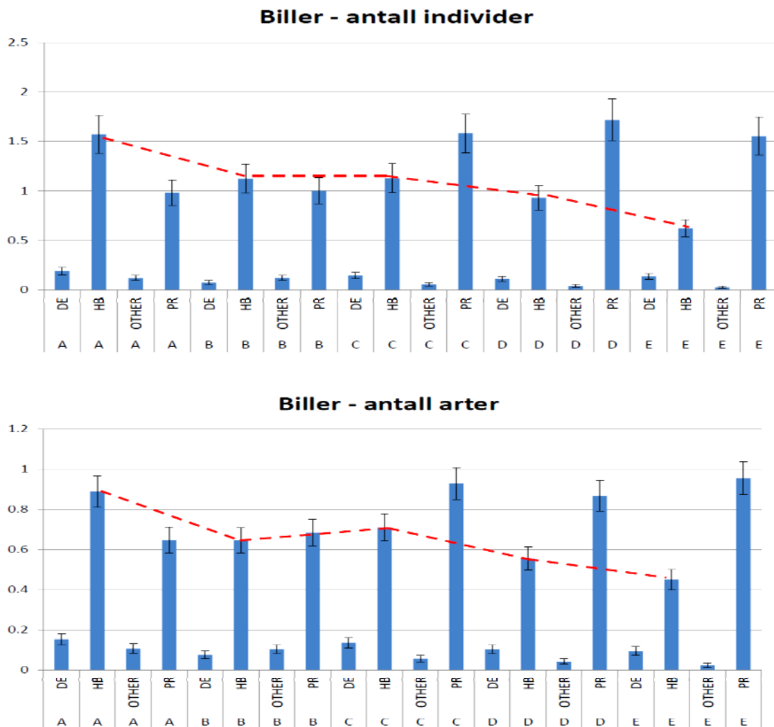
Figur 29. Antall individer (øverst) og arter (nederst) av biller fanget med slagghåv i ulike habitater i kraftgater (A, B) og skog (C, D, E), fordelt på ulike funksjonelle grupper. Figurene viser estimerte gjennomsnittsverdier og tilhørende standardfeil (mål på usikkerhet) for hhv antall individer og antall arter fanget pr 4m x 5m plott (prøveflater) vist i Figur 2, på 51 målestasjoner vist i Figur 1. Alle billeartene i materialet ble kategorisert etter deres viktigste økologiske funksjon, og plassert i en av følgende økologiske grupper: HB – herbivor (plantespiser), FU – fungivor (soppspiser), PR – predator, DW – dead wood (død ved), LW – live wood (levende ved), DE – detritivor (spiser diverse (dødt) organisk materiale). Kategoriene LW, DW og FU hadde få arter, og ble derfor slått sammen med kategorien 'OTHER' før statistiske analyser av materialet. Habitat A er midt i kraftgaten, B er i kraftgatesiden av kantsonen, C er i skogsiden av kantsonen, D er like langt inn i skogen som avstanden mellom midt i kraftgaten og kanten av kraftgaten, og E er 100 meter inn i skogen.
